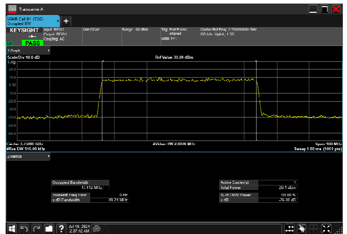
n78_3_50MHz_30kHz_3750MHz_CP-OFDM QPSK_RB133@0 47.412MHz
