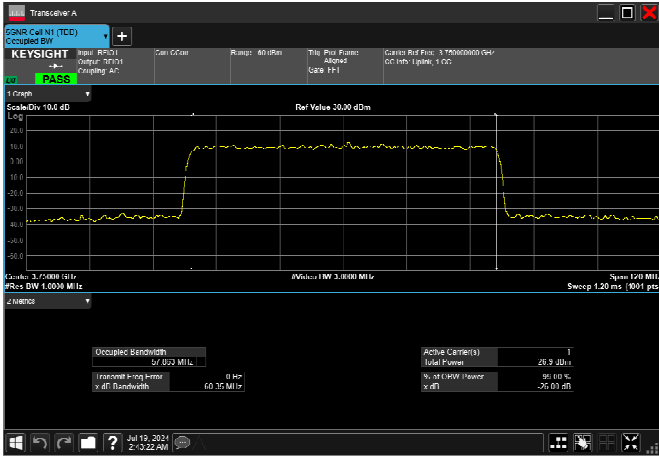
n78_3_60MHz_30kHz_3750MHz_CP-OFDM QPSK_RB162@0 57.619MHz
