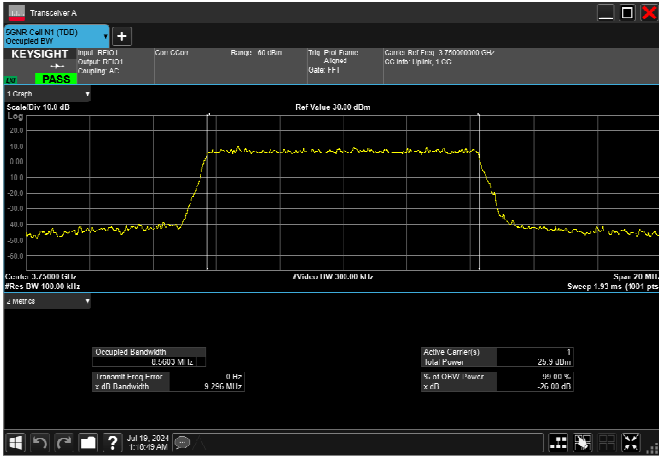
n78_3_10MHz_30kHz_3750MHz_CP-OFDM QPSK_RB24@0 8.563MHz
