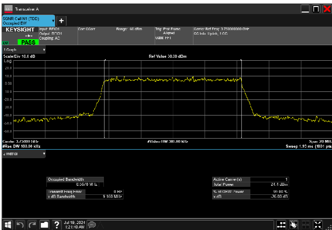
n78_3_10MHz_30kHz_3750MHz_CP-OFDM 64 QAM_RB24@0 8.568MHz
