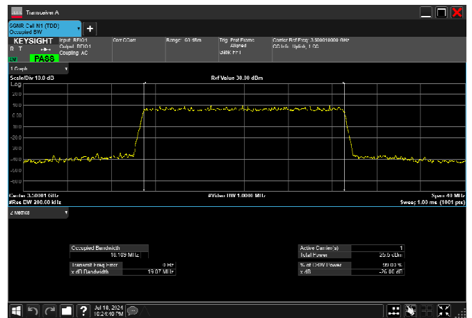
n78_1_20MHz_30kHz_3500MHz_CP-OFDM QPSK_RB51@0 18.109MHz
