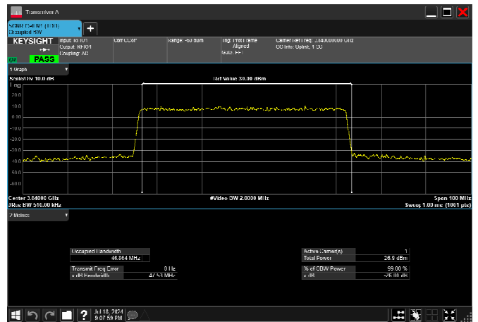
n77_3_50MHz_30kHz_3840MHz_CP-OFDM QPSK_RB133@0 47.430MHz
