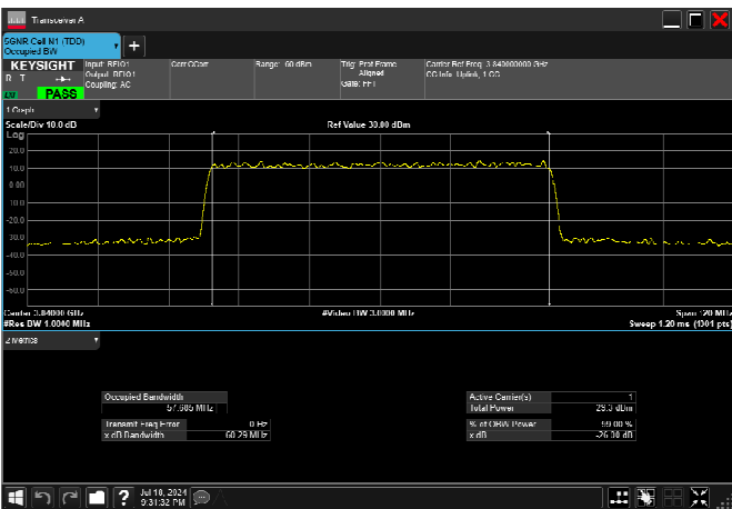
n77_3_60MHz_30kHz_3840MHz_DFT-s-OFDM QPSK_RB162@0 57.685MHz
