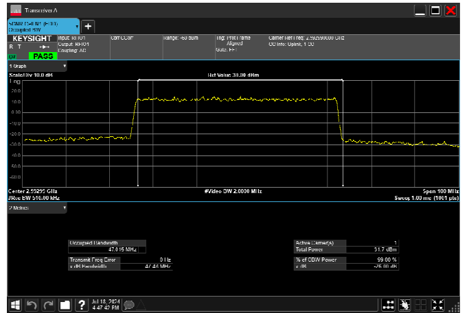
n41_50MHz_30kHz_2592.99MHz_CP-OFDM QPSK_RB133@0 47.416MHz
