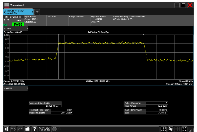
n41_30MHz_30kHz_2592.99MHz_CP-OFDM QPSK_RB78@0 27.859MHz
