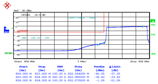
10MHz_Low_16QAM_50@0
