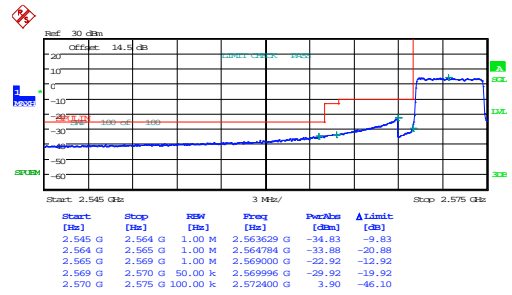
5MHz_Low_QPSK_25@0
