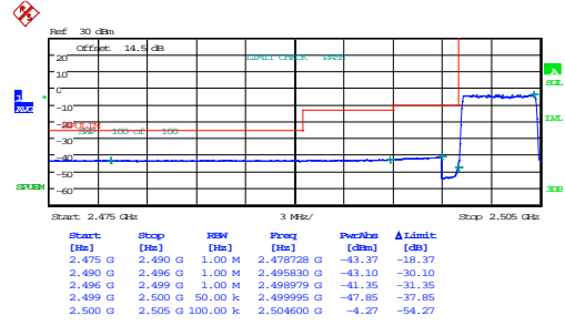
5MHz_Low_QPSK_25@0
