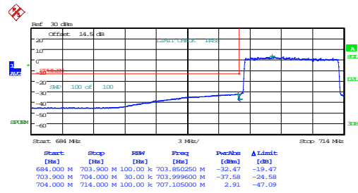
10MHz_Low_16QAM_50@0
