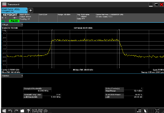
n41_10MHz_30kHz_2592.99MHz_DFT-s-OFDM QPSK_RB24@0 8.540MHz
