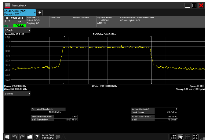
n38_20MHz_30kHz_2595MHz_DFT-s-OFDM 16 QAM_RB50@0 18.034MHz
