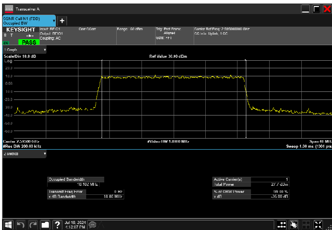
n38_20MHz_30kHz_2595MHz_DFT-s-OFDM QPSK_RB50@0 18.102MHz
