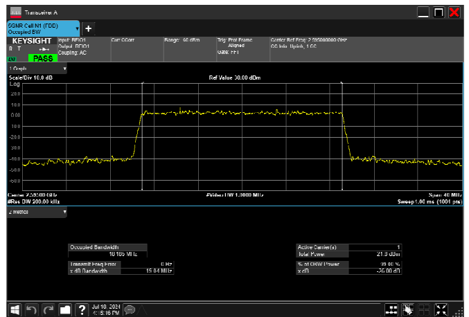
n38_20MHz_30kHz_2595MHz_CP-OFDM 256 QAM_RB51@0 18.185MHz
