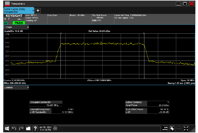
n38_20MHz_30kHz_2595MHz_DFT-s-OFDM \pi/2 BPSK_RB50@0 18.022MHz
