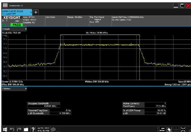
n38_10MHz_30kHz_2595MHz_DFT-s-OFDM QPSK_RB24@0 8.609MHz
