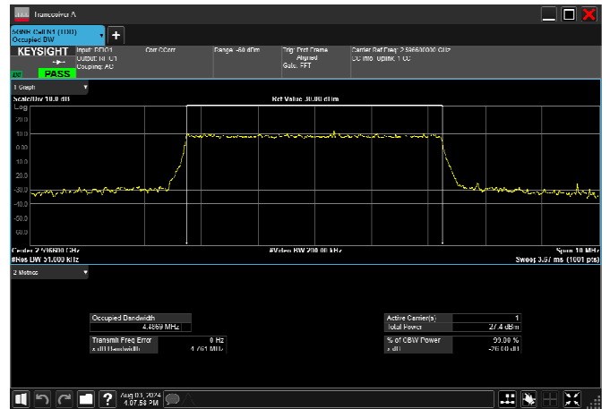
n38_5MHz_15kHz_2595MHz_CP-OFDM QPSK_RB25@0 4.468MHz
