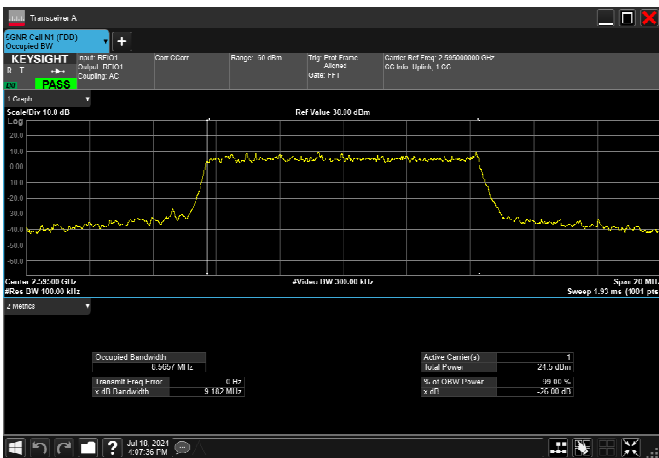
n38_10MHz_30kHz_2595MHz_CP-OFDM 64 QAM_RB24@0 8.566MHz
