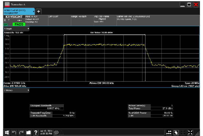
n38_10MHz_30kHz_2595MHz_DFT-s-OFDM \pi/2 BPSK_RB24@0 8.601MHz
