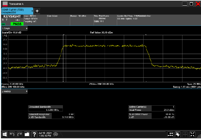
n38_10MHz_30kHz_2595MHz_CP-OFDM QPSK_RB24@0 8.570MHz
