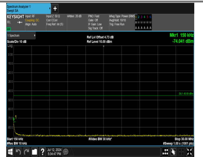
7-7-20MHz-20MHz-QPSK-QPSK-20850-21048-1RB#0-1R B#99-0.15~30MHz-PASS
