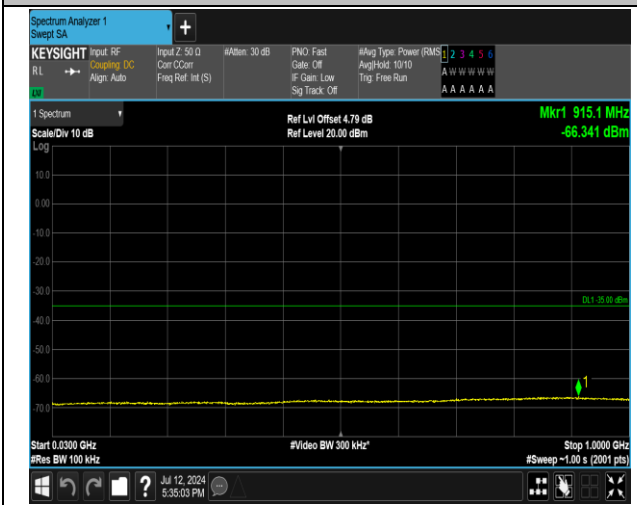
7-7-20MHz-20MHz-QPSK-QPSK-20850-21048-1RB#0-1R B#99-30~1000MHz-PASS
