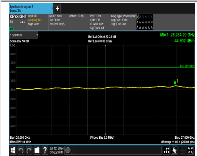
7-7-20MHz-15MHz-QPSK-QPSK-21026-21197-1RB#99-0 RB#0-20000~27000MHz-PASS
