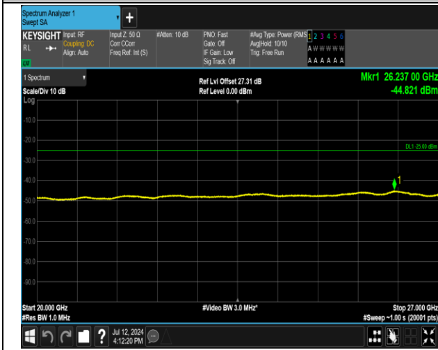
7-7-20MHz-15MHz-QPSK-QPSK-21201-21372-1RB#99-0 RB#0-20000~27000MHz-PASS
