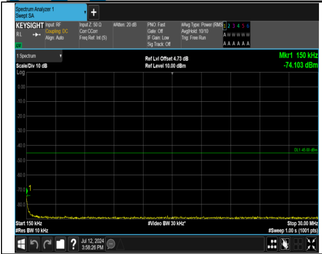
7-7-20MHz-15MHz-QPSK-QPSK-21026-21197-1RB#99-0 RB#0-0.15~30MHz-PASS
