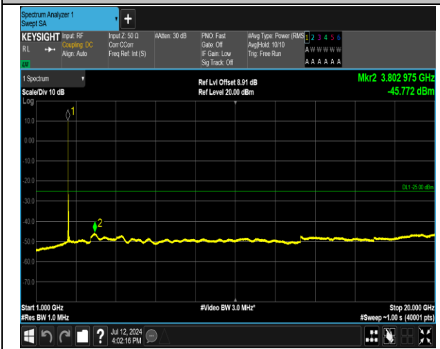
7-7-20MHz-15MHz-QPSK-QPSK-21026-21197-1RB#0-1R B#74-1000~20000MHz-PASS
