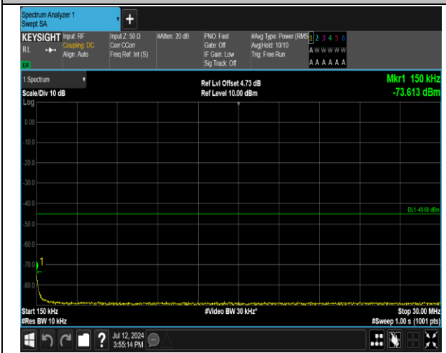
7-7-20MHz-15MHz-QPSK-QPSK-21026-21197-1RB#0-0RB#0-0.15~30MHz-PASS
