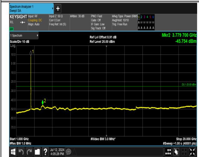
7-7-20MHz-15MHz-QPSK-QPSK-21026-21197-100RB#0-75RB#0-1000~20000MHz-PASS
