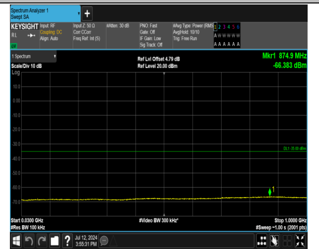
7-7-20MHz-15MHz-QPSK-QPSK-21026-21197-1RB#0-0RB#0-30~1000MHz-PASS
