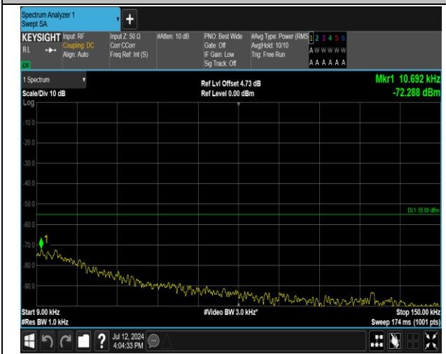
7-7-20MHz-15MHz-QPSK-QPSK-21026-21197-100RB#0-75RB#0-0.009~0.15MHz-PASS
