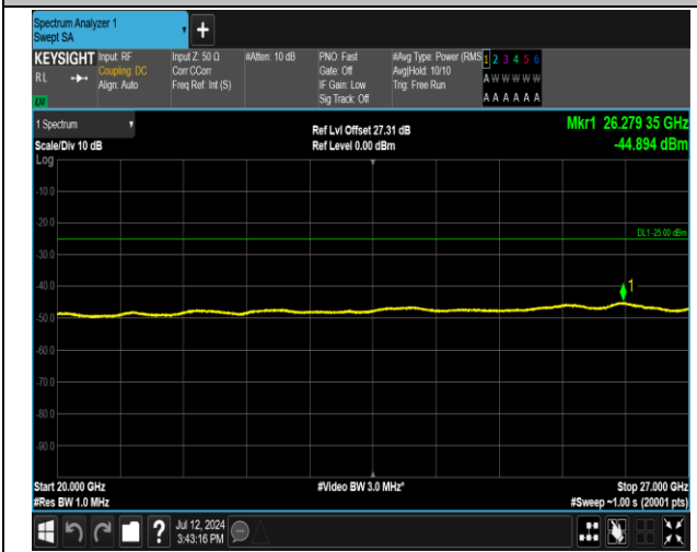
7-7-20MHz-15MHz-QPSK-QPSK-20850-21021-1RB#0-0R B#0-20000~27000MHz-PASS
