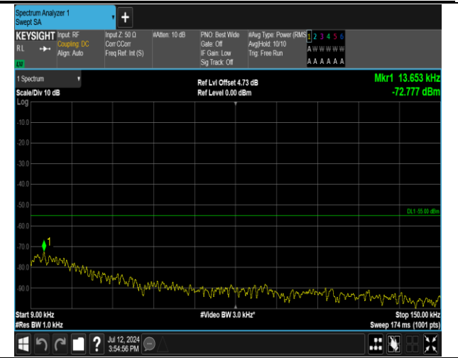
7-7-20MHz-15MHz-QPSK-QPSK-21026-21197-1RB#0-0RB#0-0.009~0.15MHz-PASS
