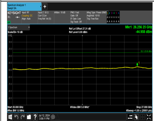
7-7-20MHz-15MHz-QPSK-QPSK-21026-21197-1RB#0-0RB#0-20000~27000MHz-PASS
