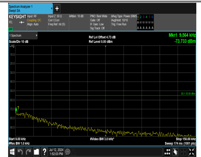
7-7-20MHz-10MHz-QPSK-QPSK-20850-20994-1RB#0-0RB#0-0.009~0.15MHz-PASS
