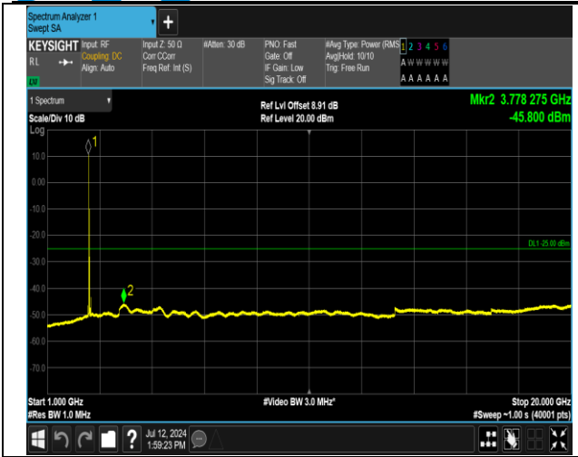
7-7-20MHz-10MHz-QPSK-QPSK-20850-20994-1RB#0-1R B#49-1000~20000MHz-PASS
