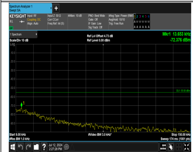
7-7-20MHz-10MHz-QPSK-QPSK-21251-21395-100RB#0-0 50RB#0-0.009~0.15MHz-PASS
