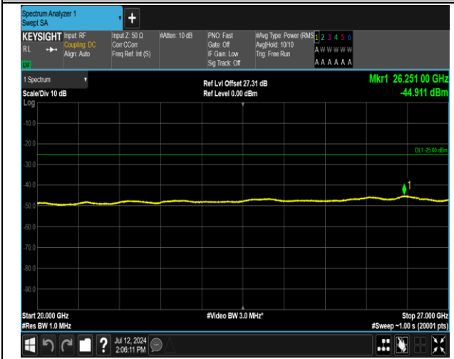
7-7-20MHz-10MHz-QPSK-QPSK-21051-21195-1RB#0-0RB#0-20000~27000MHz-PASS
