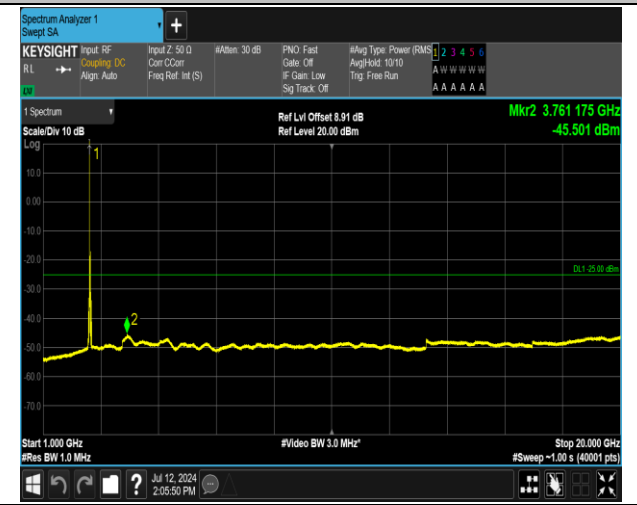
7-7-20MHz-10MHz-QPSK-QPSK-21051-21195-1RB#0-0RB#0-1000~20000MHz-PASS
