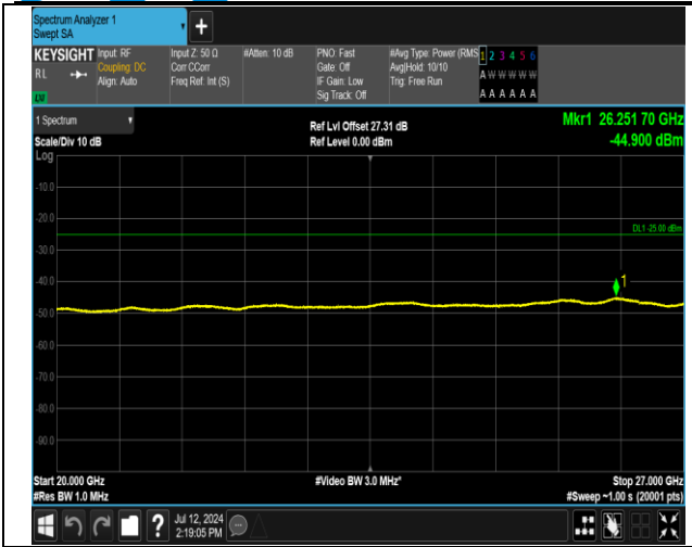
7-7-20MHz-10MHz-QPSK-QPSK-21251-21395-1RB#0-0R B#0-20000~27000MHz-PASS
