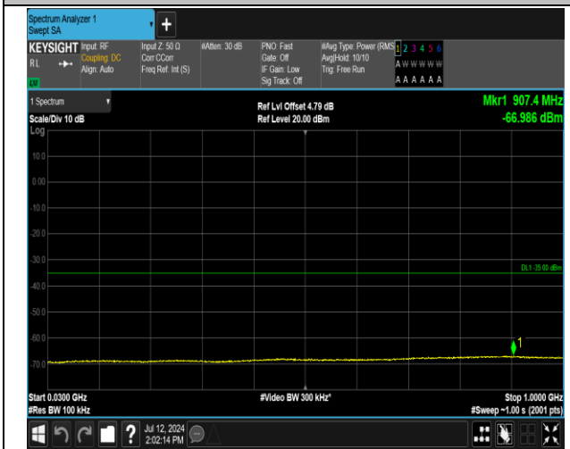
7-7-20MHz-10MHz-QPSK-QPSK-20850-20994-100RB#0-50RB#0-30~1000MHz-PASS
