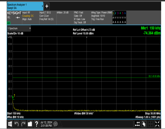
7-7-20MHz-10MHz-QPSK-QPSK-20850-20994-100RB#0-50RB#0-0.15~30MHz-PASS
