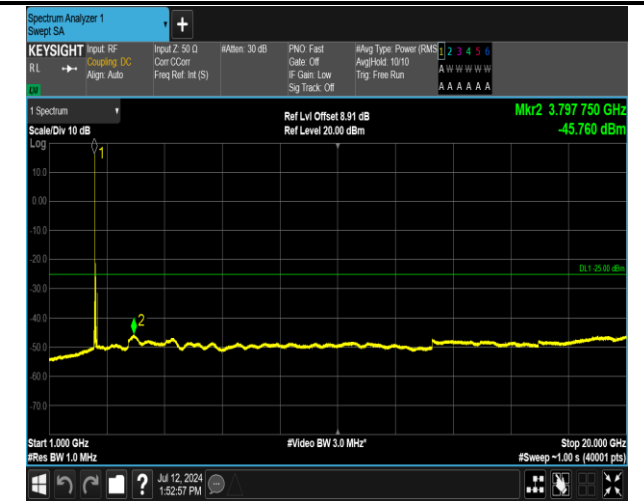
7-7-20MHz-10MHz-QPSK-QPSK-20850-20994-1RB#0-0R B#0-1000~20000MHz-PASS
