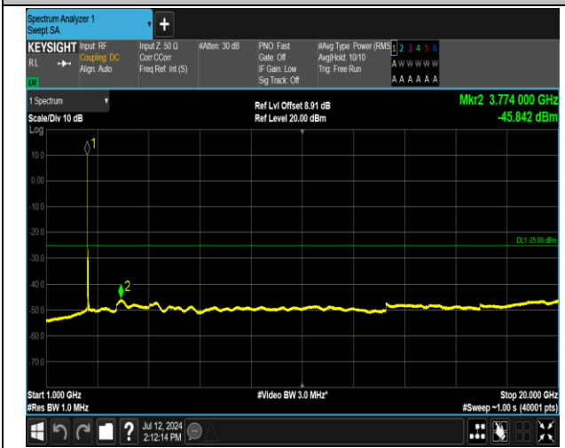
7-7-20MHz-10MHz-QPSK-QPSK-21051-21195-1RB#0-1R B#49-1000~20000MHz-PASS
