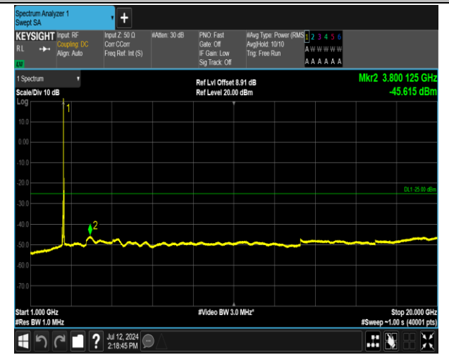
7-7-20MHz-10MHz-QPSK-QPSK-21251-21395-1RB#0-0RB#0-1000~20000MHz-PASS
