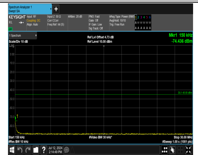
7-7-20MHz-10MHz-QPSK-QPSK-21051-21195-100RB#0-50RB#0-0.15~30MHz-PASS
