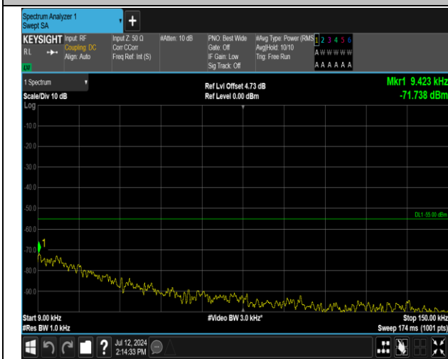
7-7-20MHz-10MHz-QPSK-QPSK-21051-21195-100RB#0-50RB#0-0.009~0.15MHz-PASS
