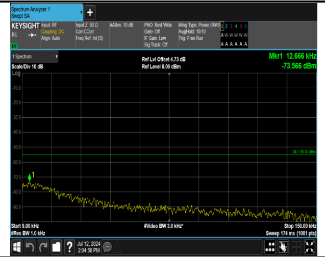
7-7-20MHz-10MHz-QPSK-QPSK-21051-21195-1RB#0-0RB#0-0.009~0.15MHz-PASS
