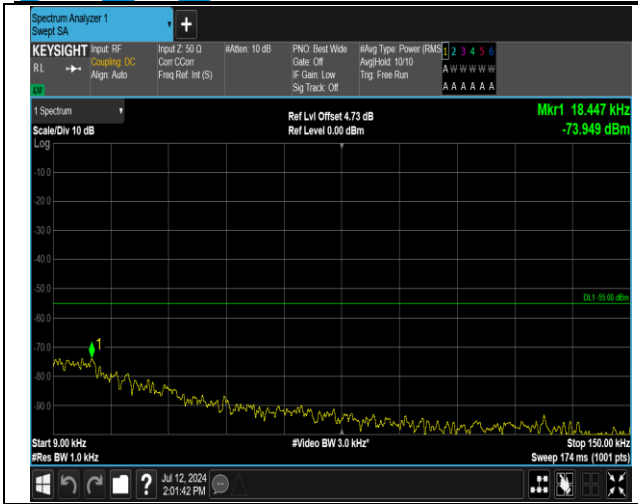
7-7-20MHz-10MHz-QPSK-QPSK-20850-20994-100RB#0-50RB#0-0.009~0.15MHz-PASS
