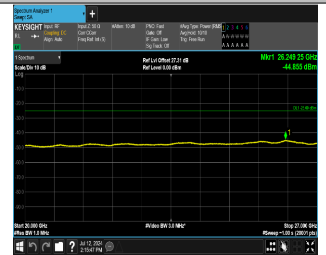
7-7-20MHz-10MHz-QPSK-QPSK-21051-21195-100RB#0-50RB#0-20000~27000MHz-PASS
