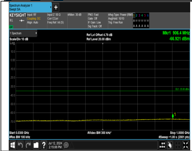
7-7-20MHz-10MHz-QPSK-QPSK-21051-21195-100RB#0-50RB#0-30~1000MHz-PASS
