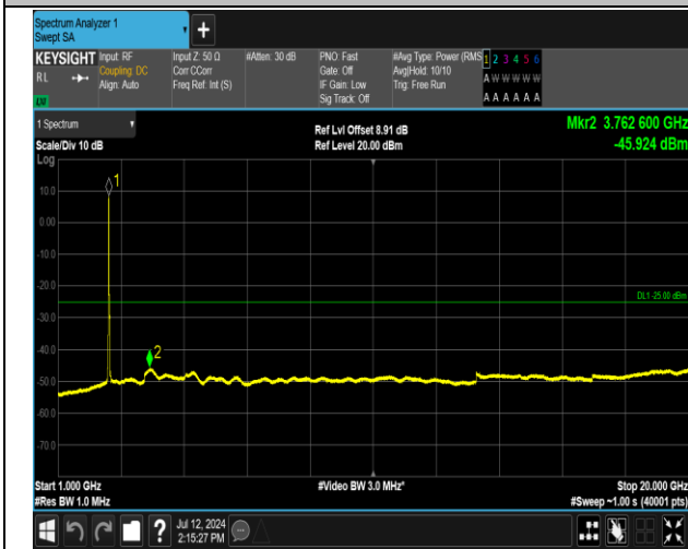
7-7-20MHz-10MHz-QPSK-QPSK-21051-21195-100RB#0-50RB#0-1000~20000MHz-PASS
