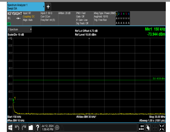
7-7-20MHz-10MHz-QPSK-QPSK-20850-20994-1RB#0-1R B#49-0.15~30MHz-PASS
