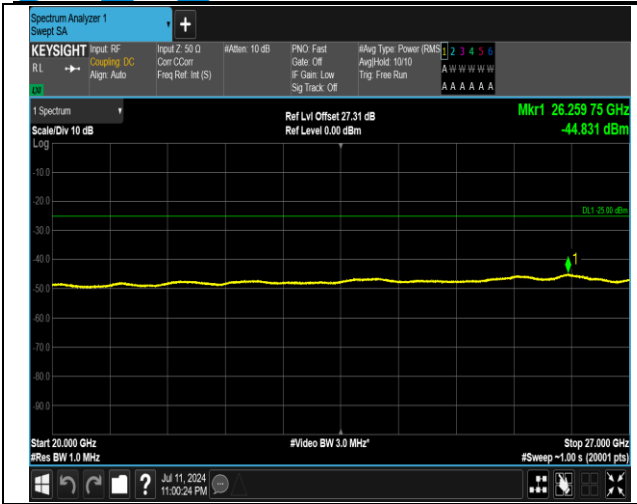
7-7-15MHz-20MHz-QPSK-QPSK-21179-21350-1RB#0-1R B#99-20000~27000MHz-PASS
