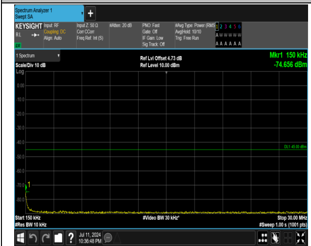
7-7-15MHz-20MHz-QPSK-QPSK-20828-20999-75RB#0-1 0ORB#0-0.15~30MHz-PASS
