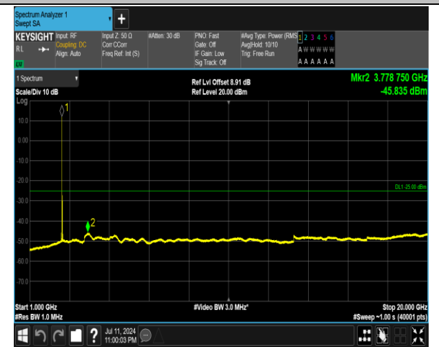
7-7-15MHz-20MHz-QPSK-QPSK-21179-21350-1RB#0-1R B#99-1000~20000MHz-PASS
