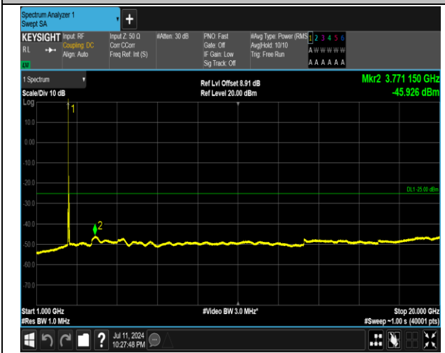
7-7-15MHz-20MHz-QPSK-QPSK-20828-20999-1RB#0-0R B#0-1000~20000MHz-PASS
