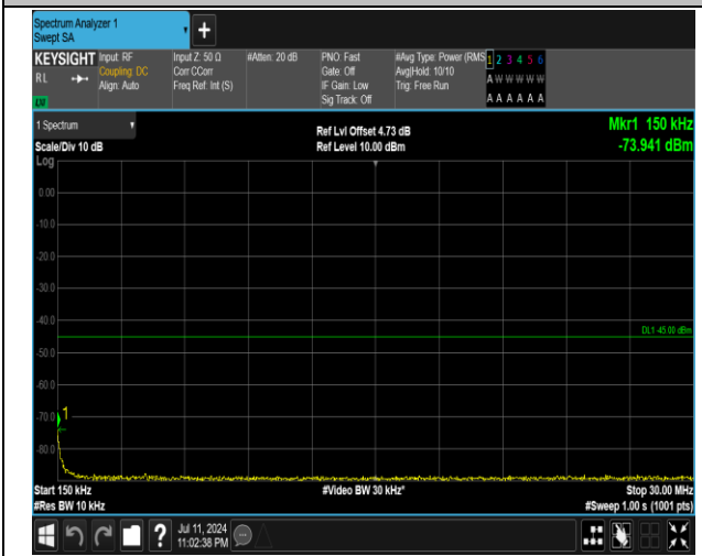
7-7-15MHz-20MHz-QPSK-QPSK-21179-21350-75RB#0-1 00RB#0-0.15~30MHz-PASS
