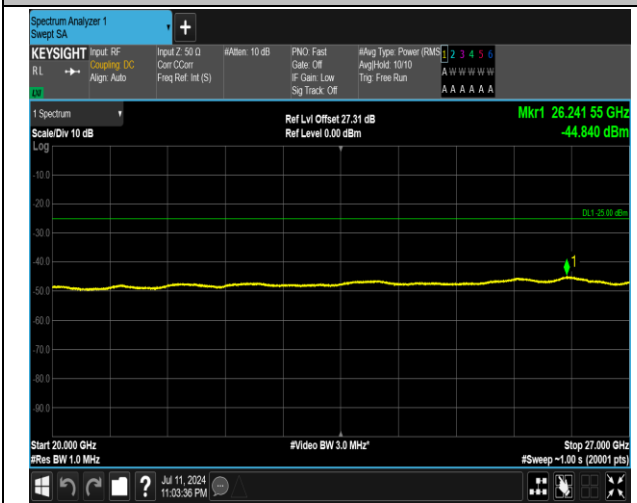
7-7-15MHz-20MHz-QPSK-QPSK-21179-21350-75RB#0-1 00RB#0-20000~27000MHz-PASS
