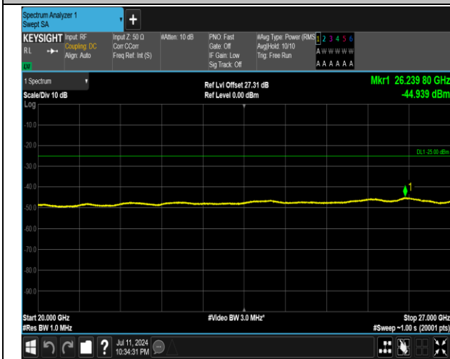
7-7-15MHz-20MHz-QPSK-QPSK-20828-20999-1RB#0-1R B#99-20000~27000MHz-PASS
