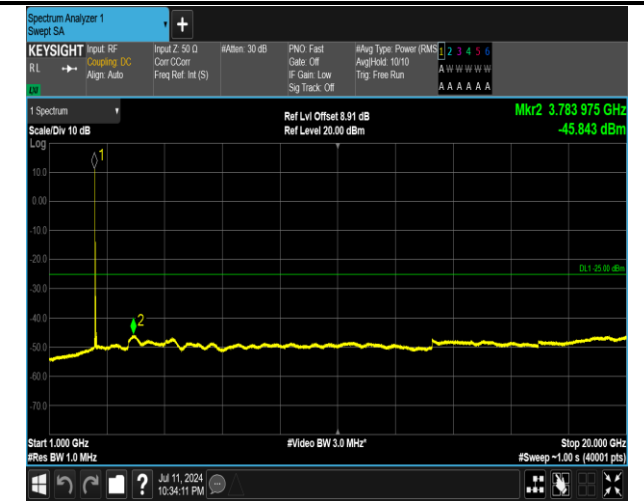
7-7-15MHz-20MHz-QPSK-QPSK-20828-20999-1RB#0-1R B#99-1000~20000MHz-PASS
