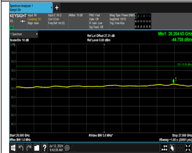
7-7-15MHz-15MHz-QPSK-QPSK-21025-21175-1RB#0-1R B#74-20000~27000MHz-PASS
