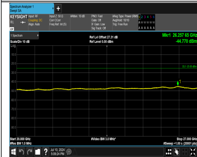
7-7-15MHz-10MHz-QPSK-QPSK-20825-20945-1RB#0-1R B#49-20000~27000MHz-PASS
