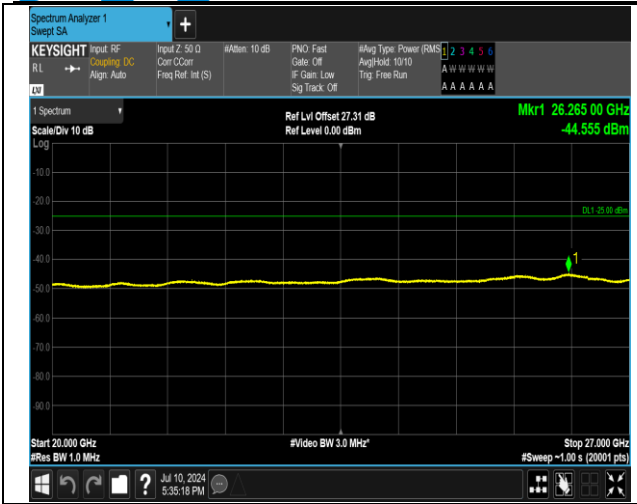
7-7-15MHz-10MHz-QPSK-QPSK-21277-21397-1RB#0-1R B#49-20000~27000MHz-PASS
