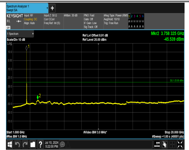
7-7-15MHz-10MHz-QPSK-QPSK-21051-21171-1RB#0-1R B#49-1000~20000MHz-PASS
