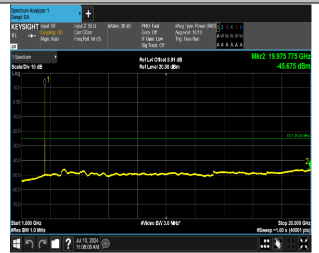
7-7-10MHz-20MHz-QPSK-QPSK-21006-21150-1RB#0-1R B#99-1000~20000MHz-PASS
