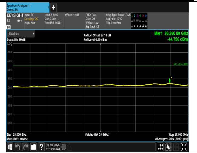
7-7-10MHz-20MHz-QPSK-QPSK-21206-21350-1RB#0-0R B#0-20000~27000MHz-PASS
