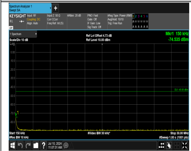
7-7-10MHz-20MHz-QPSK-QPSK-21006-21150-1RB#0-1R B#99-0.15~30MHz-PASS
