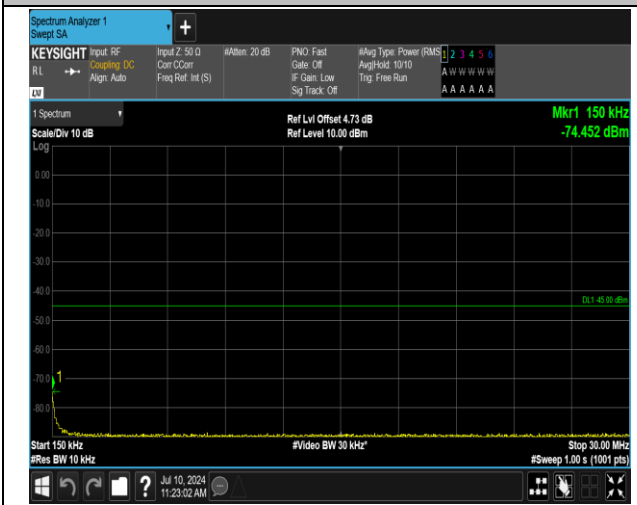
7-7-10MHz-20MHz-QPSK-QPSK-21206-21350-50RB#0-1 00RB#0-0.15~30MHz-PASS
