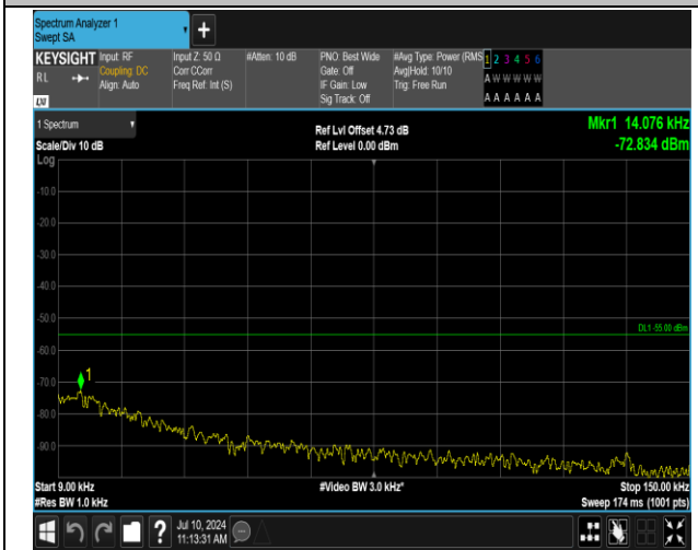
7-7-10MHz-20MHz-QPSK-QPSK-21206-21350-1RB#0-0R B#0-0.009~0.15MHz-PASS
