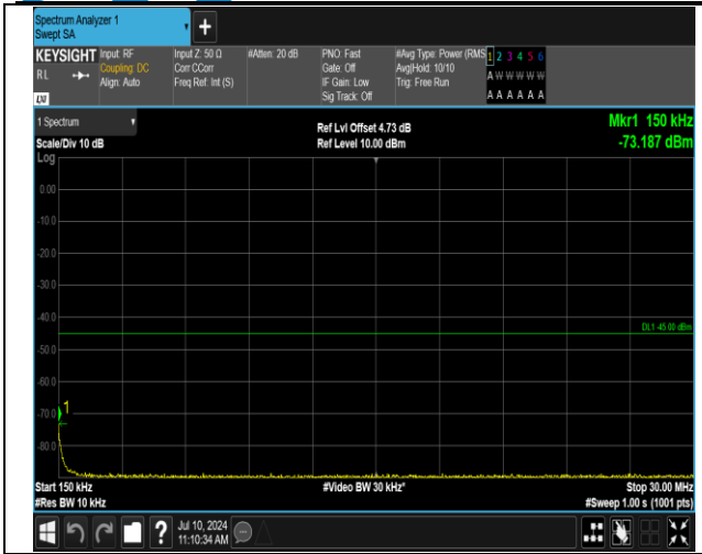
7-7-10MHz-20MHz-QPSK-QPSK-21006-21150-50RB#0-1 00RB#0-0.15~30MHz-PASS
