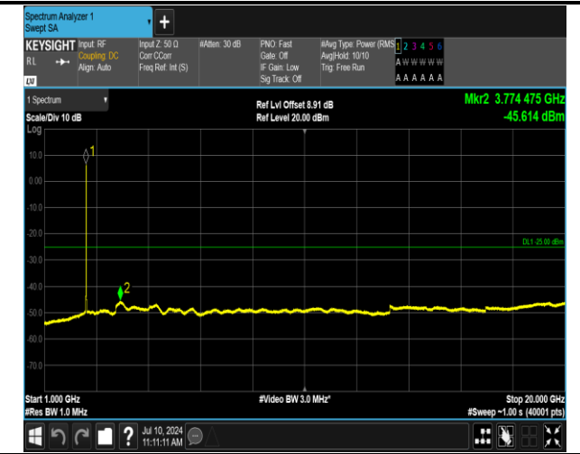
7-7-10MHz-20MHz-QPSK-QPSK-21006-21150-50RB#0-10 0RB#0-1000~20000MHz-PASS
