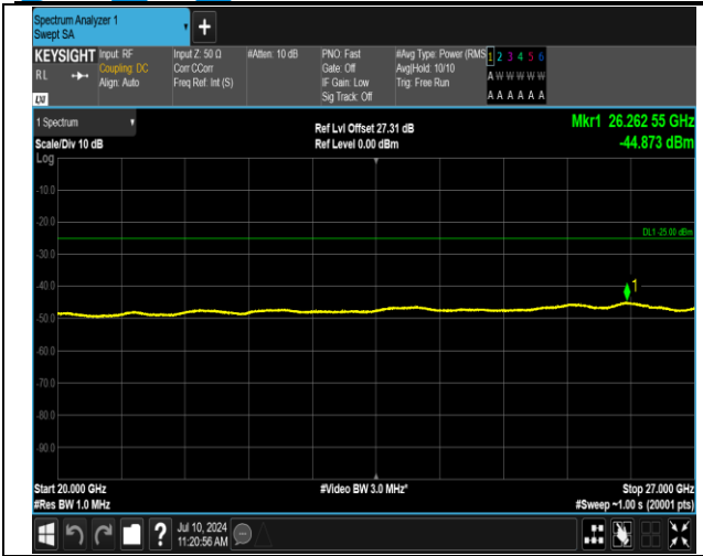
7-7-10MHz-20MHz-QPSK-QPSK-21206-21350-1RB#0-1R B#99-20000~27000MHz-PASS
