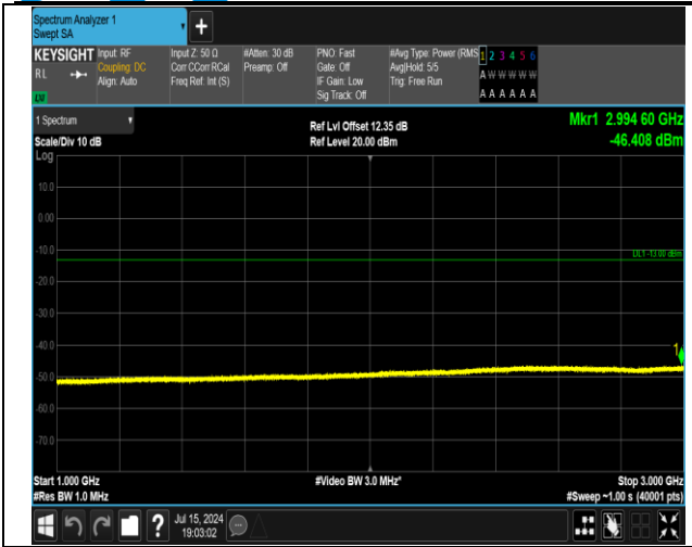
5-5-5MHz-3MHz-QPSK-QPSK-20425-20464-1RB#24-0RB #0-1000~3000MHz-PASS
