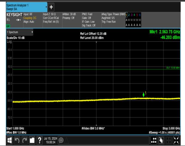
5-5-5MHz-3MHz-16QAM-16QAM-20425-20464-1RB#0-1R B#15-1000~3000MHz-PASS
