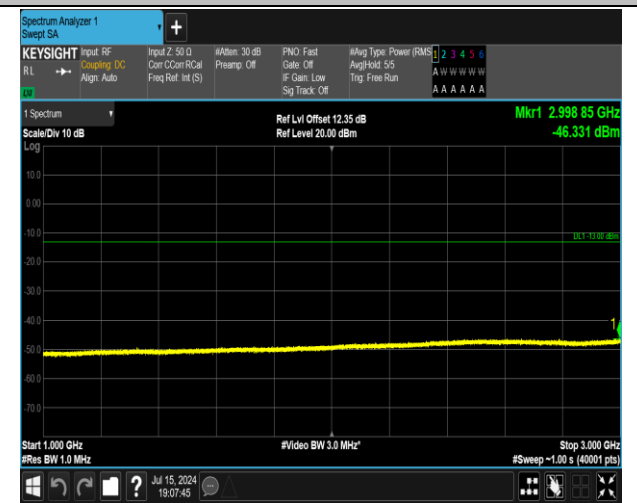
5-5-5MHz-3MHz-QPSK-QPSK-20425-20464-25RB#0-15R B#0-1000~3000MHz-PASS
