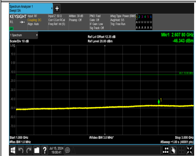
5-5-5MHz-3MHz-QPSK-QPSK-20425-20464-1RB#0-0RB# 0-1000~3000MHz-PASS
