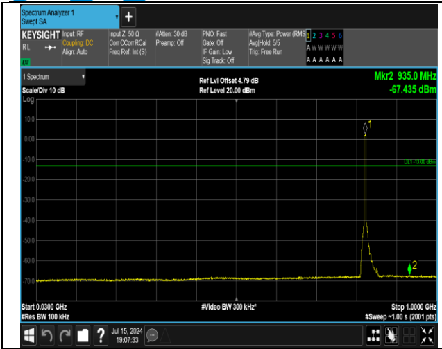
5-5-5MHz-3MHz-QPSK-QPSK-20425-20464-25RB#0-15R B#0-30~1000MHz-PASS
