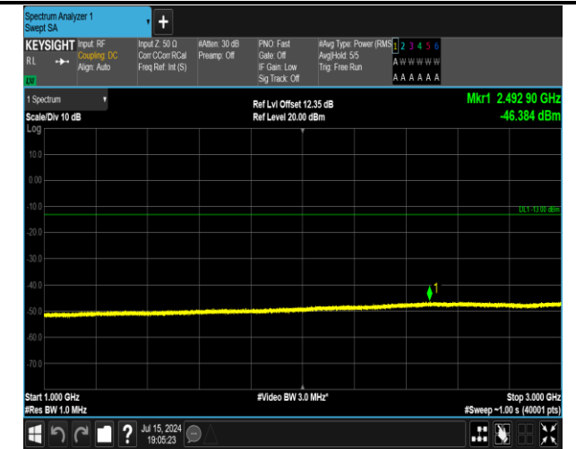
5-5-5MHz-3MHz-QPSK-QPSK-20425-20464-1RB#0-1RB# 15-1000~3000MHz-PASS
