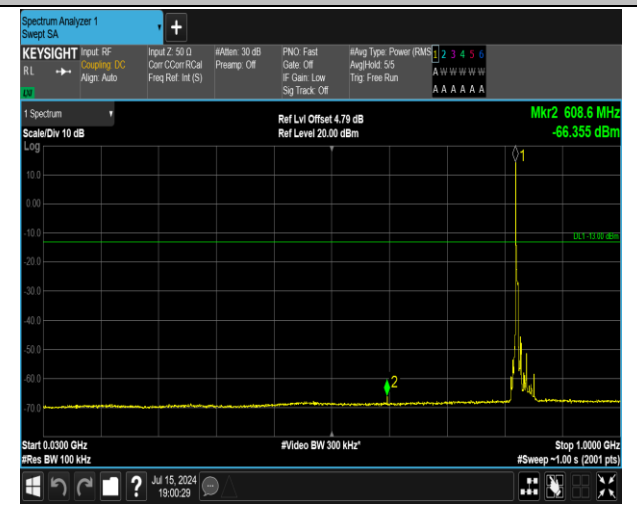
5-5-5MHz-3MHz-QPSK-QPSK-20425-20464-1RB#0-0RB# 0-30~1000MHz-PASS
