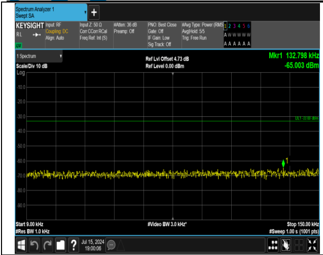
5-5-5MHz-3MHz-QPSK-QPSK-20425-20464-1RB#0-0RB# 0-0.009~0.15MHz-PASS
