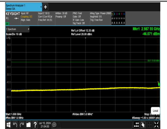
5-5-10MHz-10MHz-QPSK-QPSK-20501-20600-1RB#0-1R B#49-1000~3000MHz-PASS
