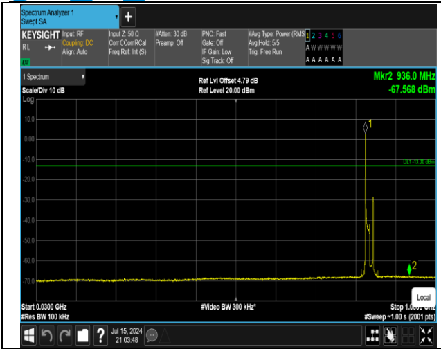
5-5-10MHz-10MHz-QPSK-QPSK-20501-20600-1RB#0-1R B#49-30~1000MHz-PASS
