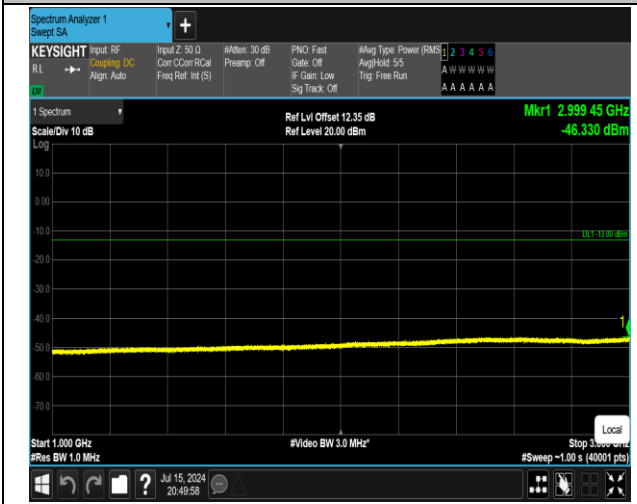
5-5-10MHz-10MHz-QPSK-QPSK-20476-20575-1RB#0-0R B#0-1000~3000MHz-PASS
