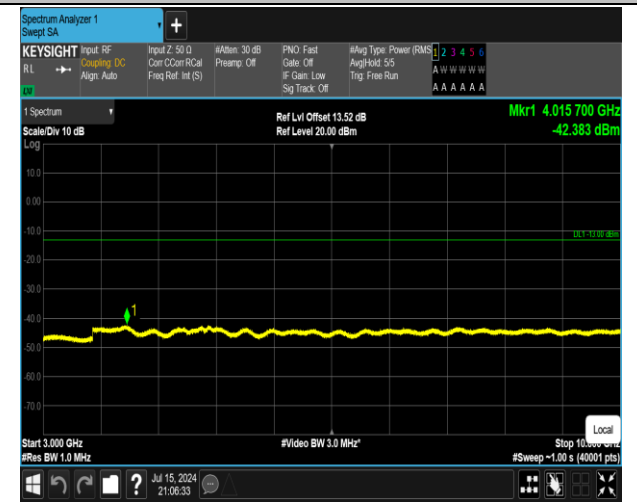
5-5-10MHz-10MHz-QPSK-QPSK-20501-20600-50RB#0-50 RB#0-3000~10000MHz-PASS
