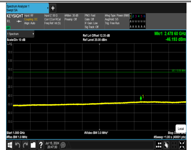
5-5-10MHz-10MHz-QPSK-QPSK-20450-20549-50RB#0-50 RB#0-1000~3000MHz-PASS
