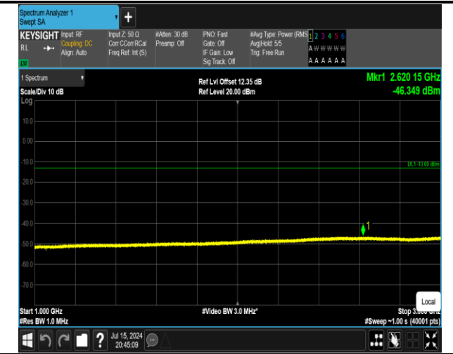
5-5-10MHz-10MHz-QPSK-QPSK-20450-20549-1RB#0-1R B#49-1000~3000MHz-PASS
