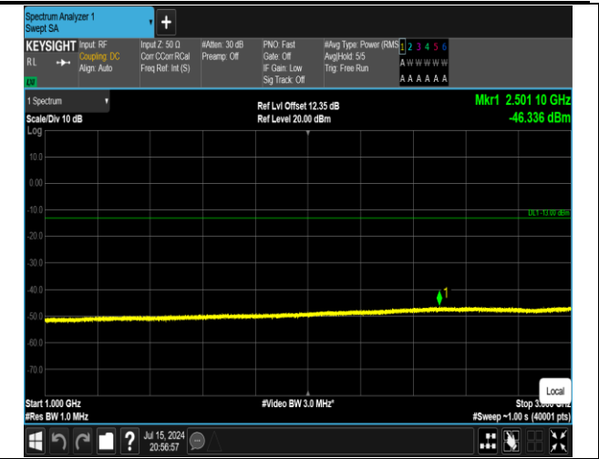
5-5-10MHz-10MHz-QPSK-QPSK-20476-20575-50RB#0-50 RB#0-1000~3000MHz-PASS
