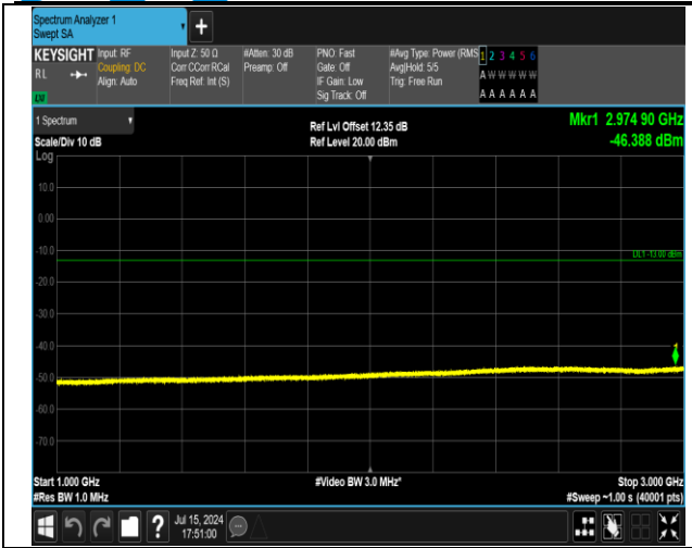
5-5-3MHz-5MHz-16QAM-16QAM-20416-20455-1RB#0-1R B#24-1000~3000MHz-PASS
