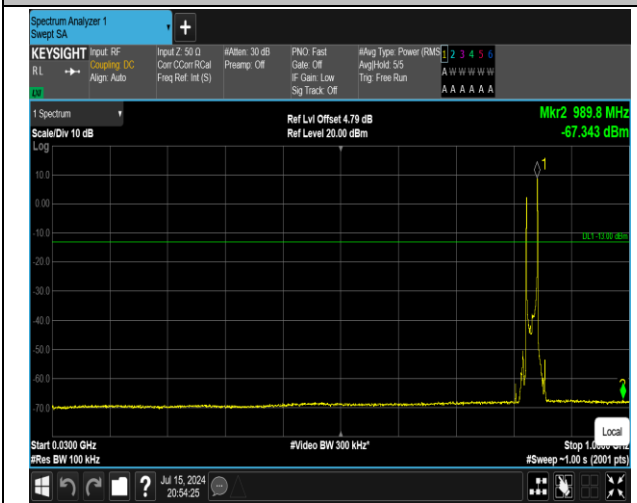
5-5-10MHz-10MHz-QPSK-QPSK-20476-20575-1RB#0-1R B#49-30~1000MHz-PASS
