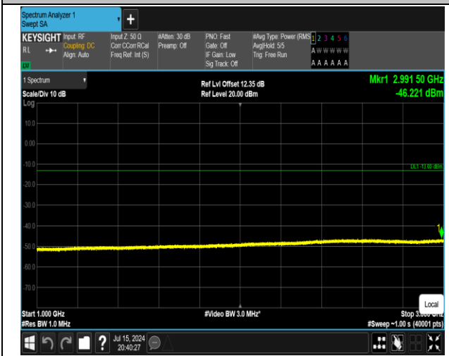
5-5-10MHz-10MHz-QPSK-QPSK-20450-20549-1RB#0-0R B#0-1000~3000MHz-PASS
