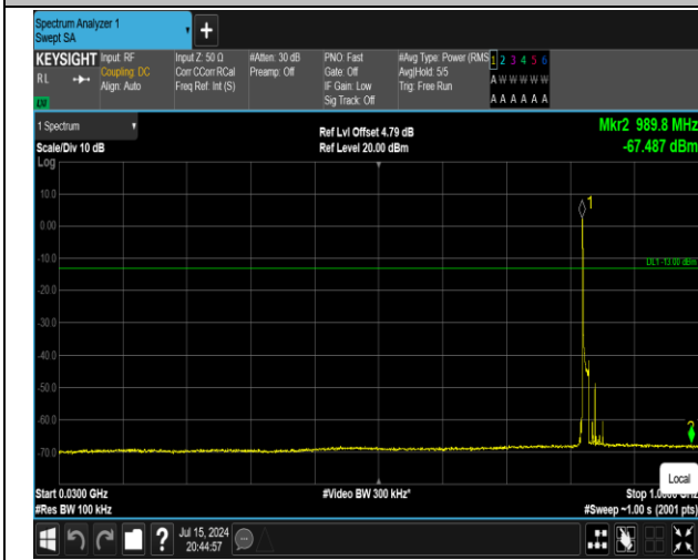
5-5-10MHz-10MHz-QPSK-QPSK-20450-20549-1RB#0-1R B#49-30~1000MHz-PASS
