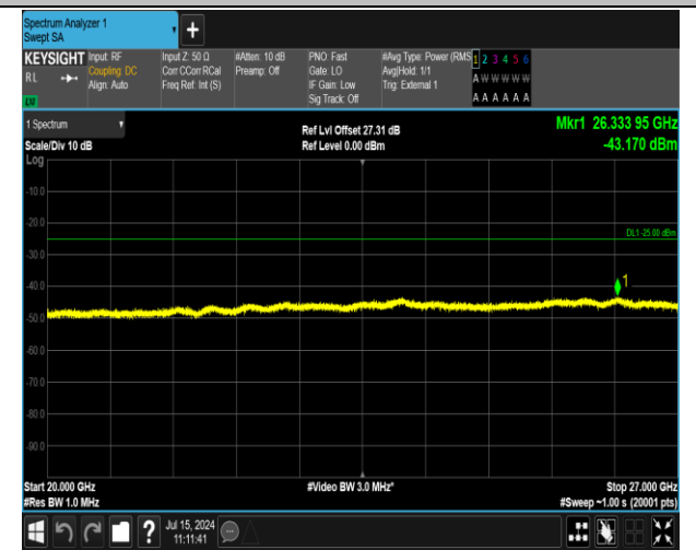
41(2555-2655)-41(2555-2655)-5MHz-20MHz-QPSK-QPSK -41023-41140-1RB#24-0RB#0-20000~27000MHz-PASS
