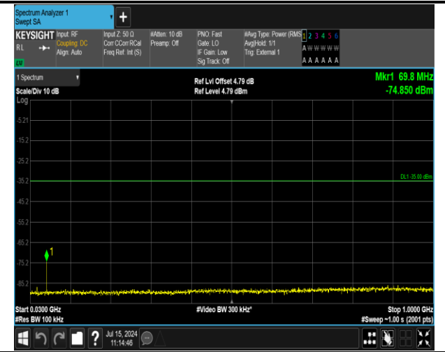
41(2555-2655)-41(2555-2655)-5MHz-20MHz-QPSK-QPSK -41023-41140-1RB#0-1RB#99-30~1000MHz-PASS
