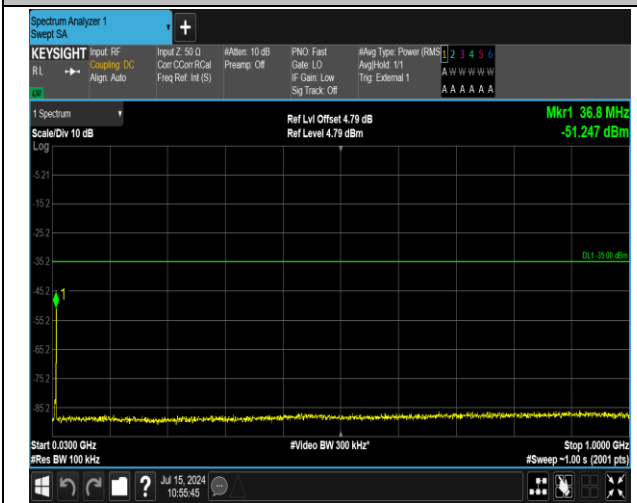
41(2555-2655)-41(2555-2655)-5MHz-20MHz-QPSK-QPSK K-40648-40765-1RB#24-ORB#0-30~1000MHz-PASS
