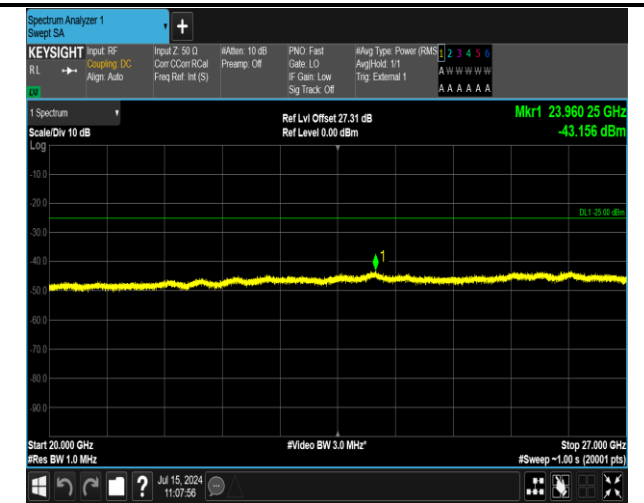
41(2555-2655)-41(2555-2655)-5MHz-20MHz-QPSK-QPSK -41023-41140-1RB#0-0RB#0-20000~27000MHz-PASS
