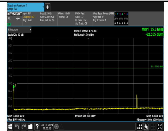
41(2555-2655)-41(2555-2655)-5MHz-20MHz-QPSK-QPSK -40648-40765-25RB#0-100RB#0-30~1000MHz-PASS
