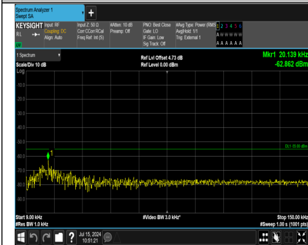
41(2555-2655)-41(2555-2655)-5MHz-20MHz-QPSK-QPS K-40648-40765-1RB#0-0RB#0-0.009~0.15MHz-PASS
