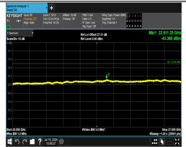
41(2555-2655)-41(2555-2655)-5MHz-20MHz-QPSK-QPSK -40648-40765-1RB#24-ORB#0-20000~27000MHz-PASS
