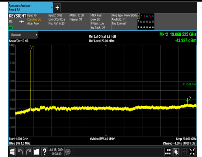
41(2555-2655)-41(2555-2655)-5MHz-20MHz-QPSK-QPSK -40648-40765-25RB#0-100RB#0-1000~20000MHz-PASS
