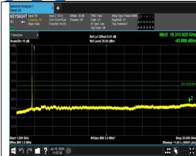
41(2555-2655)-41(2555-2655)-5MHz-20MHz-QPSK-QPS K-41023-41140-1RB#0-0RB#0-1000~20000MHz-PASS
