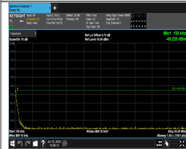
41(2555-2655)-41(2555-2655)-5MHz-20MHz-QPSK-QPSK K-40648-40765-1RB#0-1RB#99-0.15~30MHz-PASS
