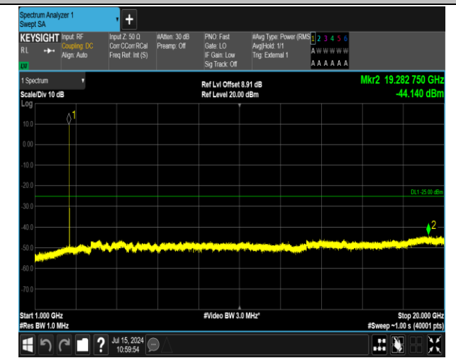
41(2555-2655)-41(2555-2655)-5MHz-20MHz-QPSK-QPSK -40648-40765-1RB#0-1RB#99-1000~20000MHz-PASS
