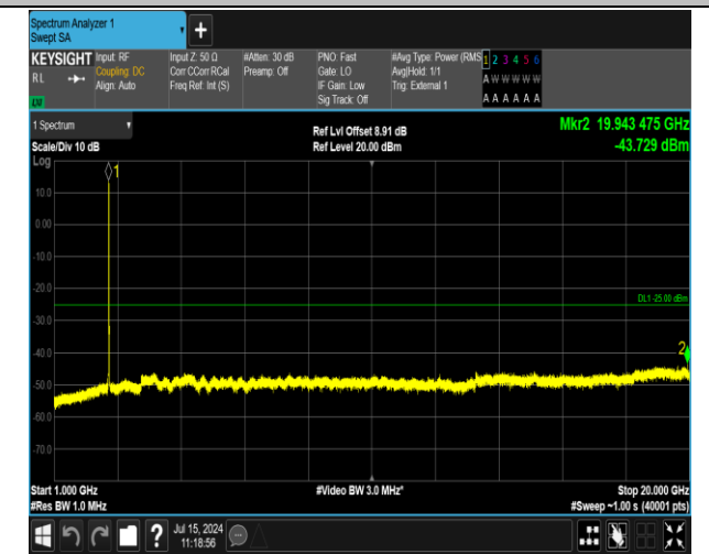
41(2555-2655)-41(2555-2655)-5MHz-20MHz-QPSK-QPSK -41023-41140-25RB#0-100RB#0-1000~20000MHz-PASS
