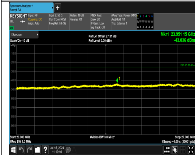
41(2555-2655)-41(2555-2655)-5MHz-20MHz-QPSK-QPS K-41023-41140-25RB#0-100RB#0-20000~27000MHz-PA SS
