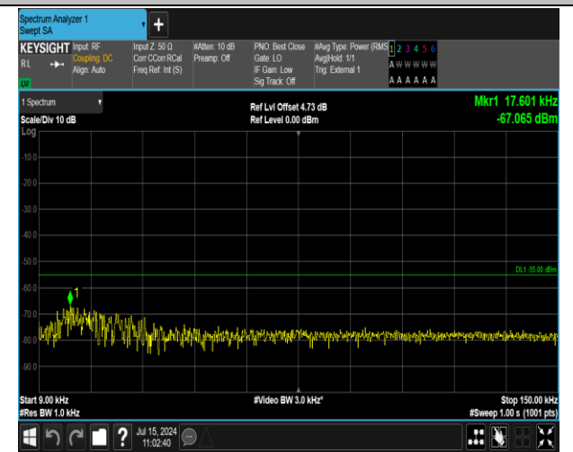
41(2555-2655)-41(2555-2655)-5MHz-20MHz-QPSK-QPSK -40648-40765-25RB#0-100RB#0-0.009~0.15MHz-PASS
