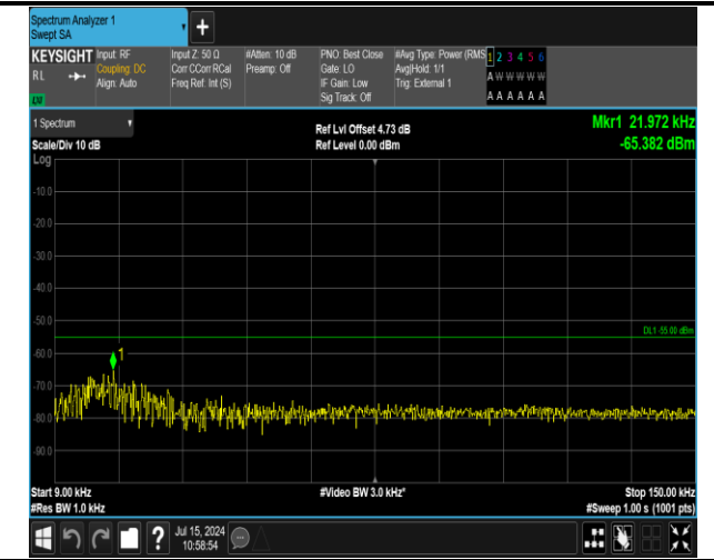
41(2555-2655)-41(2555-2655)-5MHz-20MHz-QPSK-QPSK -40648-40765-1RB#0-1RB#99-0.009~0.15MHz-PASS
