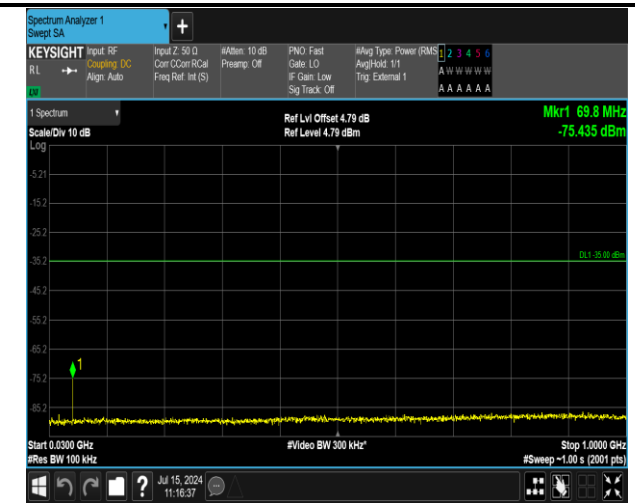
41(2555-2655)-41(2555-2655)-5MHz-20MHz-16QAM-16Q AM-41023-41140-1RB#0-1RB#99-30~1000MHz-PASS
