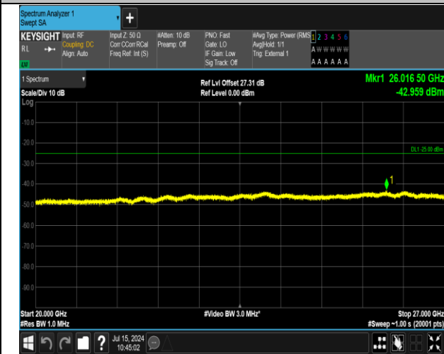
41(2555-2655)-41(2555-2655)-5MHz-20MHz-QPSK-QPS K-40273-40390-1RB#0-1RB#99-20000~27000MHz-PASS
