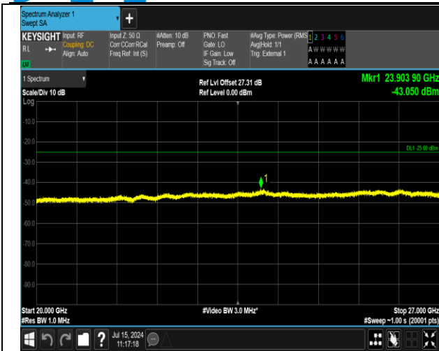
41(2555-2655)-41(2555-2655)-5MHz-20MHz-16QAM-16Q AM-41023-41140-1RB#0-1RB#99-20000~27000MHz-PAS S
