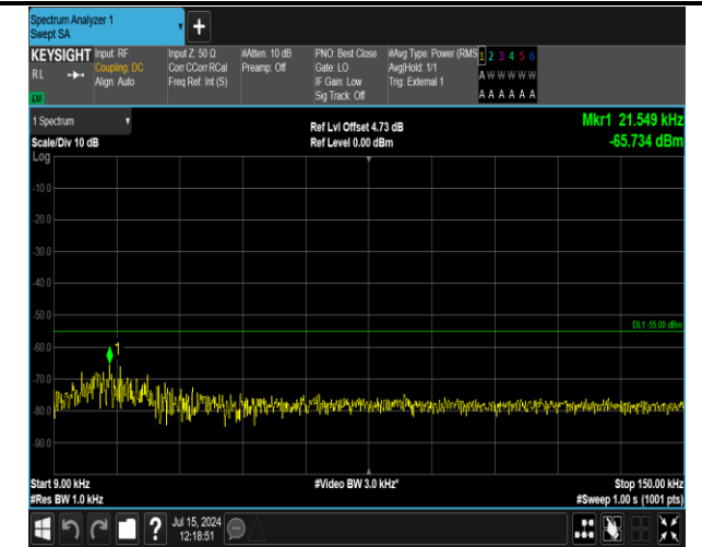
41(2555-2655)-41(2555-2655)-20MHz-5MHz-QPSK-QPSK -41090-41207-1RB#0-0RB#0-0.009~0.15MHz-PASS
