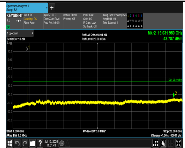
41(2555-2655)-41(2555-2655)-5MHz-20MHz-16QAM-16Q AM-40648-40765-1RB#0-1RB#99-1000~20000MHz-PASS
