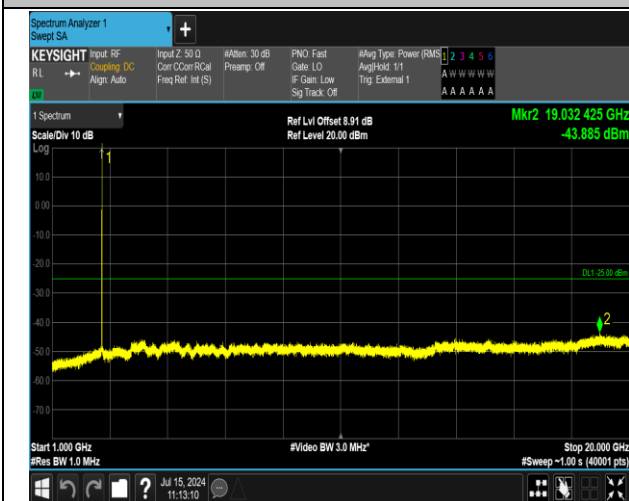
41(2555-2655)-41(2555-2655)-5MHz-20MHz-16QAM-16Q AM-41023-41140-1RB#24-0RB#0-1000~20000MHz-PASS
