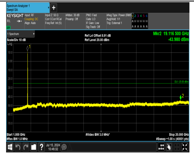
41(2555-2655)-41(2555-2655)-5MHz-20MHz-16QAM-16Q AM-40273-40390-1RB#0-1RB#99-1000~20000MHz-PASS
