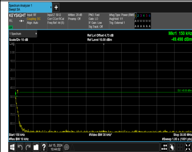
41(2555-2655)-41(2555-2655)-5MHz-20MHz-QPSK-QPS K-40273-40390-1RB#0-1RB#99-0.15~30MHz-PASS
