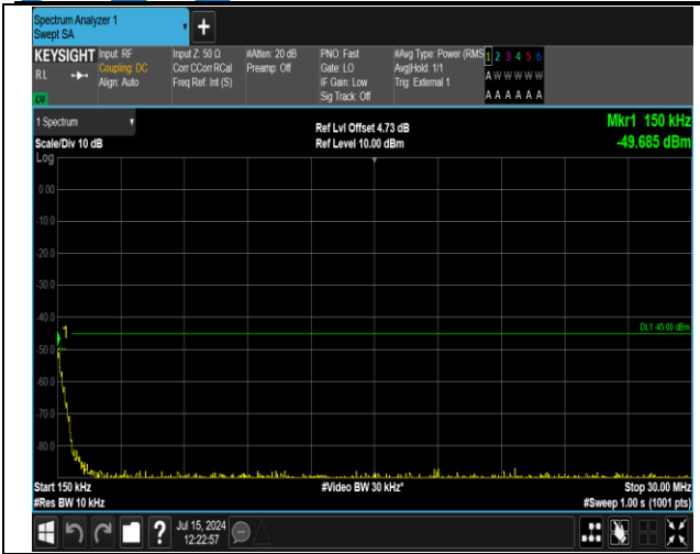
41(2555-2655)-41(2555-2655)-20MHz-5MHz-QPSK-QPSK K-41090-41207-1RB#99-0RB#0-0.15~30MHz-PASS
