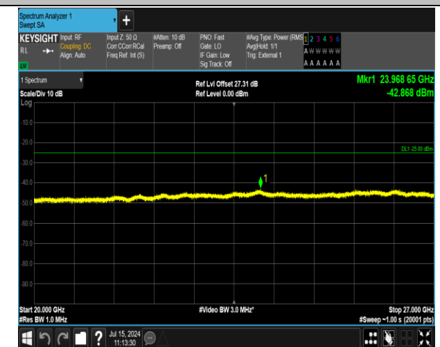
41(2555-2655)-41(2555-2655)-5MHz-20MHz-16QAM-16Q AM-41023-41140-1RB#24-0RB#0-20000~27000MHz-PAS
