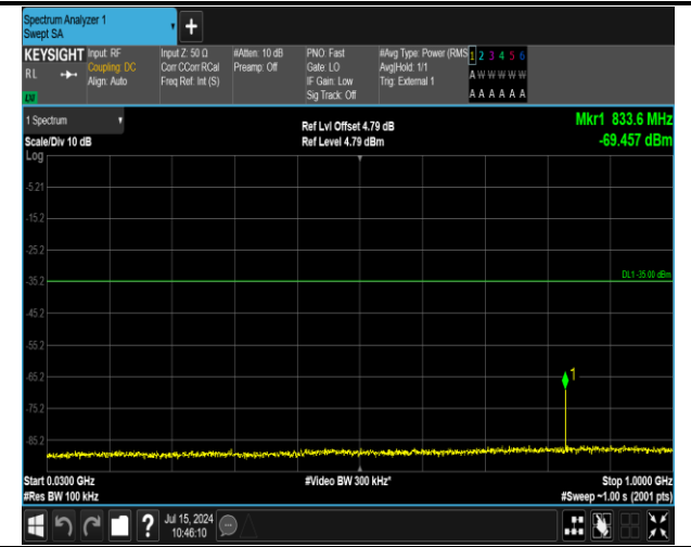
41(2555-2655)-41(2555-2655)-5MHz-20MHz-16QAM-16Q AM-40273-40390-1RB#0-1RB#99-30~1000MHz-PASS
