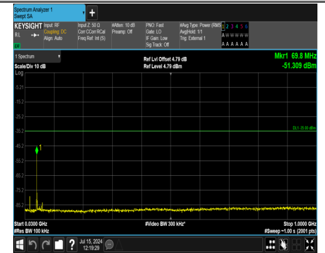
41(2555-2655)-41(2555-2655)-20MHz-5MHz-QPSK-QPSK -41090-41207-1RB#0-0RB#0-30~1000MHz-PASS
