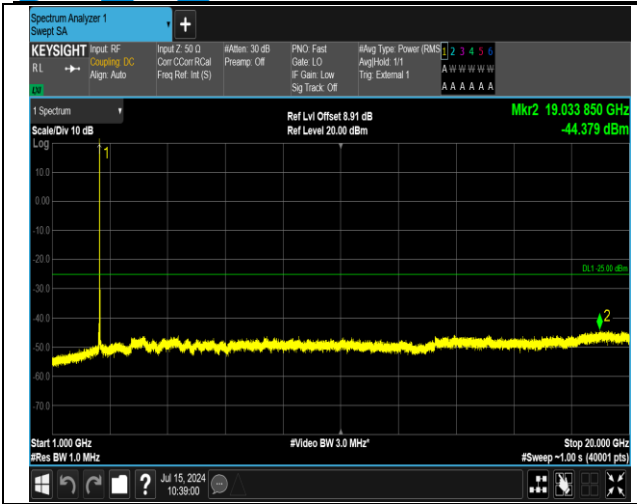
41(2555-2655)-41(2555-2655)-5MHz-20MHz-16QAM-16Q AM-40273-40390-1RB#0-ORB#0-1000~20000MHz-PASS
