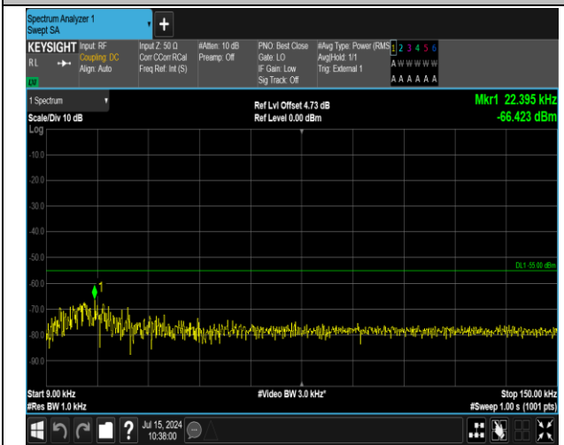
41(2555-2655)-41(2555-2655)-5MHz-20MHz-16QAM-16Q AM-40273-40390-1RB#0-0RB#0-0.009~0.15MHz-PASS
