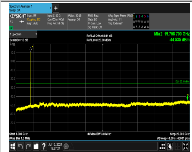
41(2555-2655)-41(2555-2655)-20MHz-5MHz-QPSK-QPS K-41090-41207-1RB#0-1RB#24-1000~20000MHz-PASS
