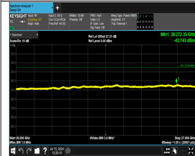
41(2555-2655)-41(2555-2655)-20MHz-5MHz-QPSK-QPSK K-41090-41207-1RB#0-0RB#0-20000~27000MHz-PASS
