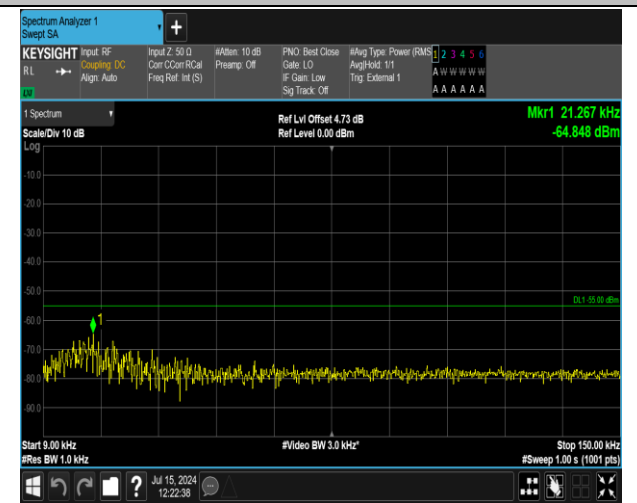
41(2555-2655)-41(2555-2655)-20MHz-5MHz-QPSK-QPSK -41090-41207-1RB#99-0RB#0-0.009~0.15MHz-PASS
