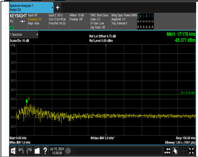
41(2555-2655)-41(2555-2655)-20MHz-5MHz-QPSK-QPS K-41090-41207-1RB#0-1RB#24-0.009~0.15MHz-PASS
