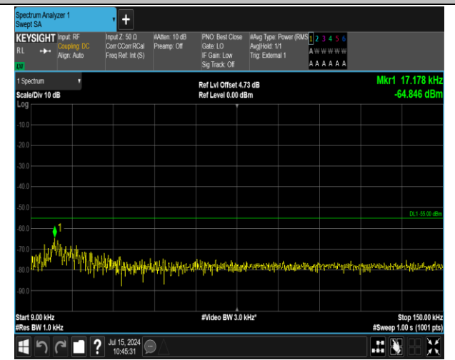
41(2555-2655)-41(2555-2655)-5MHz-20MHz-16QAM-16Q AM-40273-40390-1RB#0-1RB#99-0.009~0.15MHz-PASS
