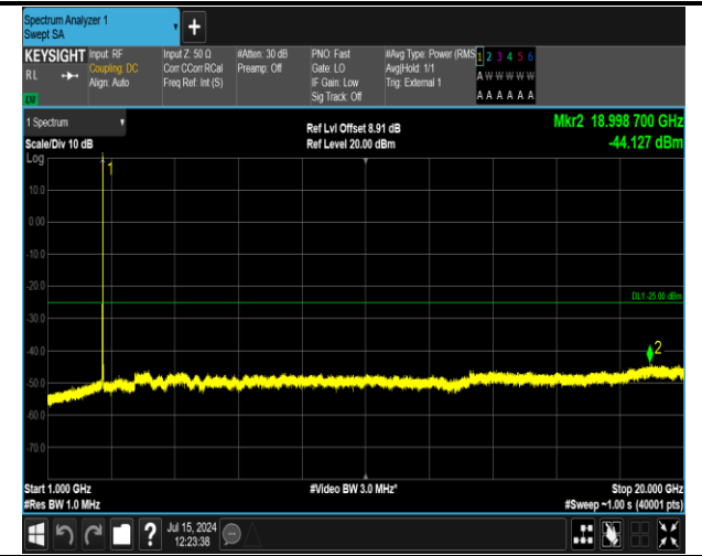
41(2555-2655)-41(2555-2655)-20MHz-5MHz-QPSK-QPSK -41090-41207-1RB#99-0RB#0-1000~20000MHz-PASS
