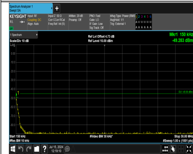
41(2555-2655)-41(2555-2655)-20MHz-5MHz-QPSK-QPSK K-41090-41207-1RB#0-0RB#0-0.15~30MHz-PASS
