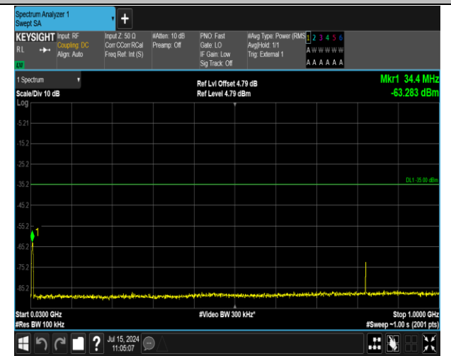
41(2555-2655)-41(2555-2655)-5MHz-20MHz-16QAM-16QAM-40648-40765-25RB#0-100RB#0-30~1000MHz-PASS
