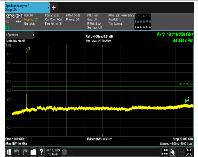
41(2555-2655)-41(2555-2655)-5MHz-20MHz-QPSK-QPSK -40273-40390-1RB#0-1RB#99-1000~20000MHz-PASS
