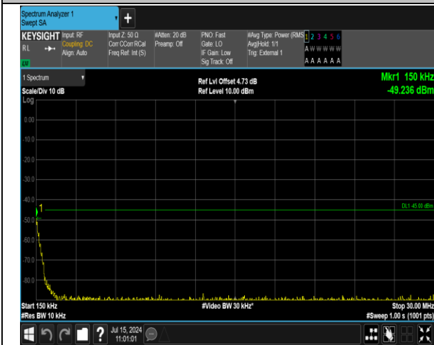
41(2555-2655)-41(2555-2655)-5MHz-20MHz-16QAM-16Q AM-40648-40765-1RB#0-1RB#99-0.15~30MHz-PASS
