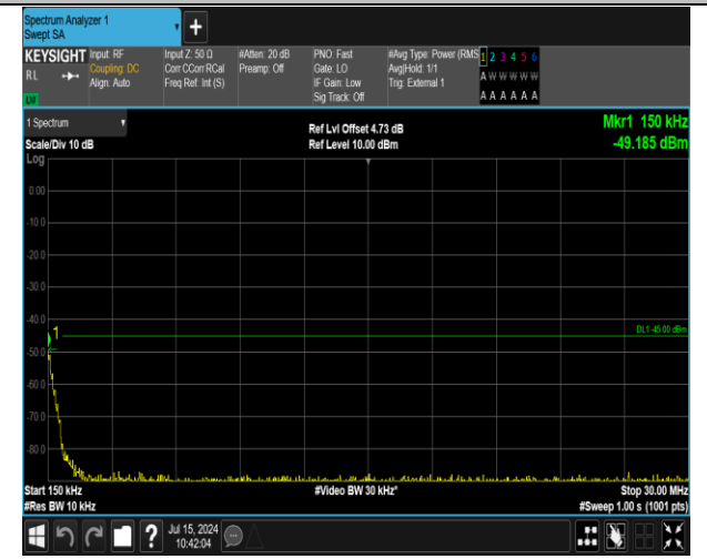
41(2555-2655)-41(2555-2655)-5MHz-20MHz-16QAM-16Q AM-40273-40390-1RB#24-0RB#0-0.15~30MHz-PASS
