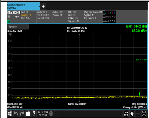
41(2555-2655)-41(2555-2655)-5MHz-20MHz-16QAM-16Q AM-40273-40390-1RB#0-ORB#0-30~1000MHz-PASS
