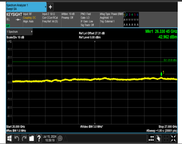
41(2555-2655)-41(2555-2655)-5MHz-20MHz-16QAM-16Q AM-40273-40390-1RB#0-ORB#0-20000~27000MHz-PASS
