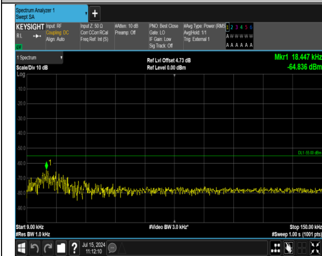
41(2555-2655)-41(2555-2655)-5MHz-20MHz-16QAM-16Q AM-41023-41140-1RB#24-0RB#0-0.009~0.15MHz-PASS
