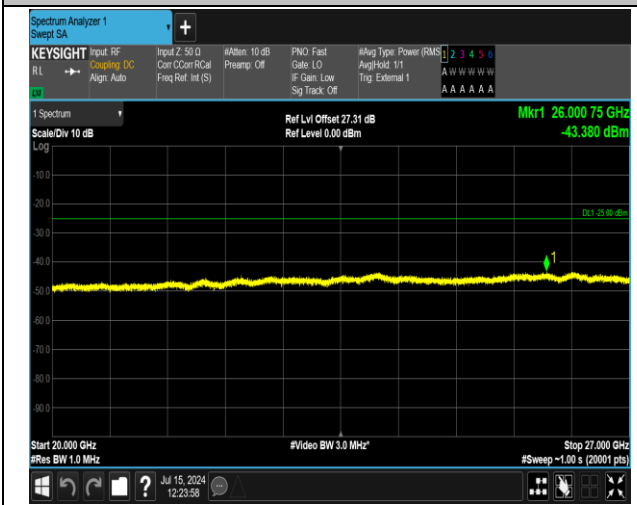
41(2555-2655)-41(2555-2655)-20MHz-5MHz-QPSK-QPSK K-41090-41207-1RB#99-0RB#0-20000~27000MHz-PASS
