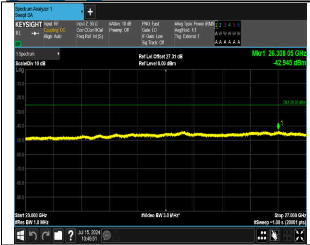
41(2555-2655)-41(2555-2655)-5MHz-20MHz-16QAM-16Q AM-40273-40390-1RB#0-1RB#99-20000~27000MHz-PAS S
