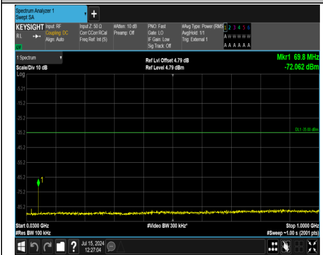
41(2555-2655)-41(2555-2655)-20MHz-5MHz-QPSK-QPS K-41090-41207-1RB#0-1RB#24-30~1000MHz-PASS
