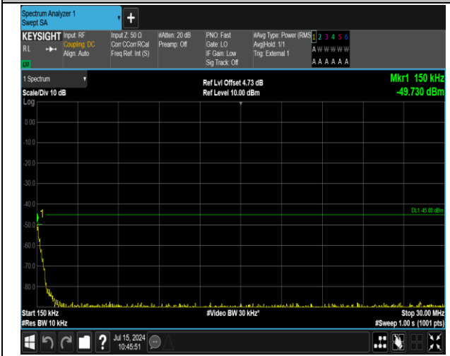
41(2555-2655)-41(2555-2655)-5MHz-20MHz-16QAM-16Q AM-40273-40390-1RB#0-1RB#99-0.15~30MHz-PASS
