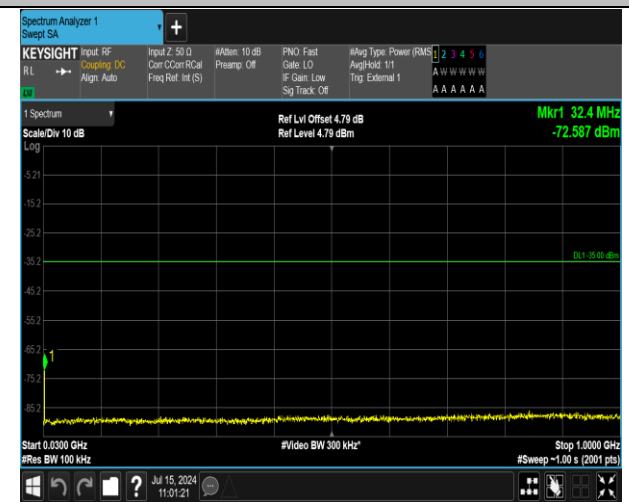
41(2555-2655)-41(2555-2655)-5MHz-20MHz-16QAM-16Q AM-40648-40765-1RB#0-1RB#99-30~1000MHz-PASS
