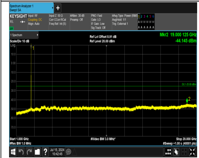
41(2555-2655)-41(2555-2655)-5MHz-20MHz-16QAM-16Q AM-40273-40390-1RB#24-0RB#0-1000~20000MHz-PASS
