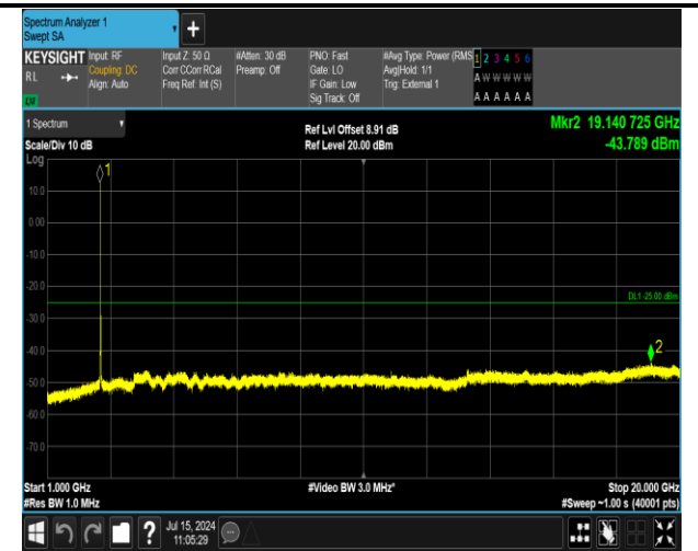
41(2555-2655)-41(2555-2655)-5MHz-20MHz-16QAM-16QAM-40648-40765-25RB#0-100RB#0-1000~20000MHz-PASS
