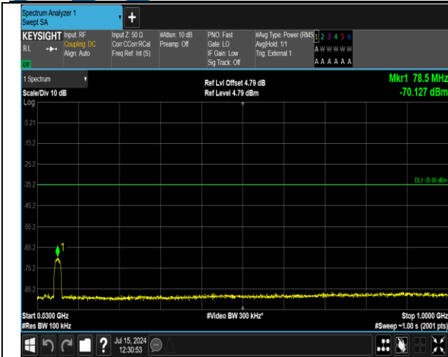
41(2555-2655)-41(2555-2655)-20MHz-5MHz-QPSK-QPSK K-41090-41207-100RB#0-25RB#0-30~1000MHz-PASS
