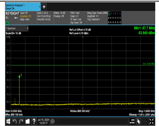
41(2555-2655)-41(2555-2655)-20MHz-5MHz-QPSK-QPSK -41090-41207-1RB#99-0RB#0-30~1000MHz-PASS
