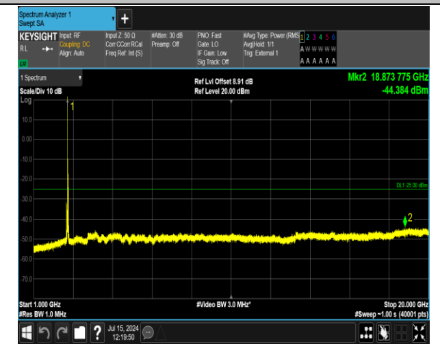
41(2555-2655)-41(2555-2655)-20MHz-5MHz-QPSK-QPSK -41090-41207-1RB#0-0RB#0-1000~20000MHz-PASS
