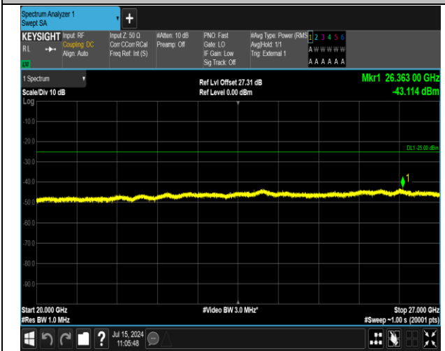
41(2555-2655)-41(2555-2655)-5MHz-20MHz-16QAM-16QAM-40648-40765-25RB#0-100RB#0-20000~27000MHz-PASS
