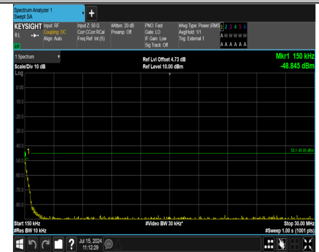
41(2555-2655)-41(2555-2655)-5MHz-20MHz-16QAM-16Q AM-41023-41140-1RB#24-0RB#0-0.15~30MHz-PASS
