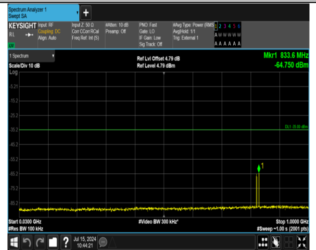
41(2555-2655)-41(2555-2655)-5MHz-20MHz-QPSK-QPSK -40273-40390-1RB#0-1RB#99-30~1000MHz-PASS
