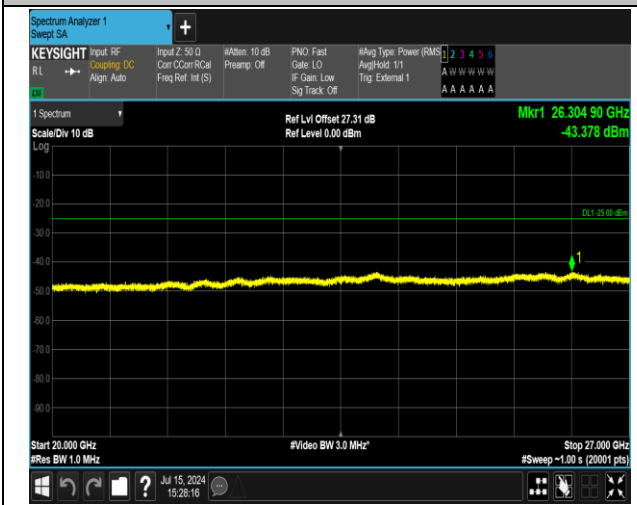
41(2555-2655)-41(2555-2655)-20MHz-20MHz-QPSK-QPS K-40942-41140-1RB#99-ORB#0-20000~27000MHz-PASS
