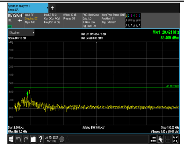
41(2555-2655)-41(2555-2655)-20MHz-20MHz-QPSK-QPS K-40641-40839-1RB#99-0RB#0-0.009~0.15MHz-PASS
