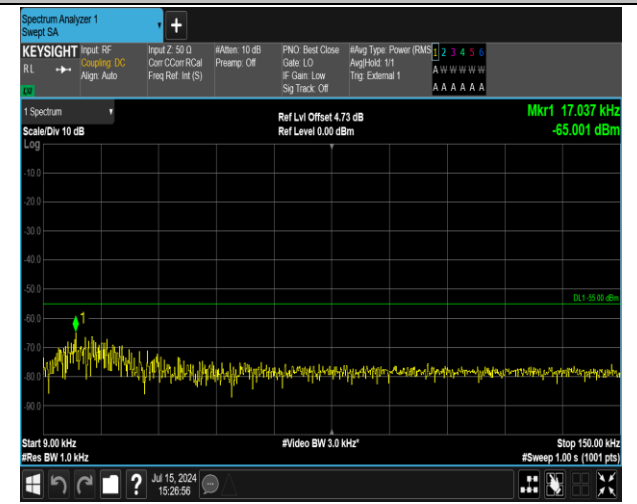
41(2555-2655)-41(2555-2655)-20MHz-20MHz-QPSK-QPS K-40942-41140-1RB#99-0RB#0-0.009~0.15MHz-PASS
