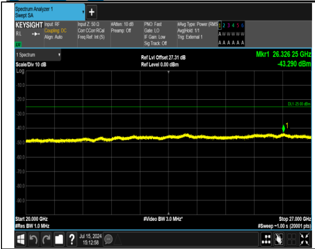
41(2555-2655)-41(2555-2655)-20MHz-20MHz-QPSK-QPS K-40641-40839-1RB#99-0RB#0-20000~27000MHz-PASS
