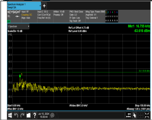
41(2555-2655)-41(2555-2655)-20MHz-20MHz-QPSK-QPS K-40942-41140-1RB#0-1RB#99-0.009~0.15MHz-PASS
