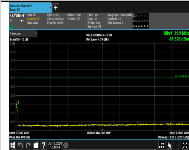
41(2555-2655)-41(2555-2655)-20MHz-20MHz-QPSK-QPS
