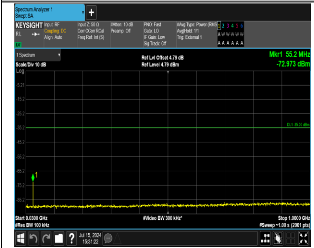
41(2555-2655)-41(2555-2655)-20MHz-20MHz-QPSK-QPS K-40942-41140-1RB#0-1RB#99-30~1000MHz-PASS
