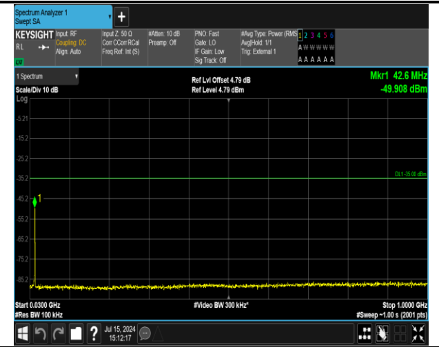
41(2555-2655)-41(2555-2655)-20MHz-20MHz-QPSK-QPS K-40641-40839-1RB#99-0RB#0-30~1000MHz-PASS
