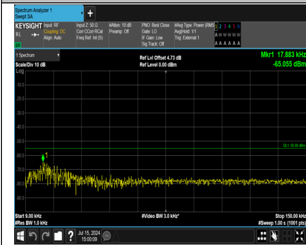
41(2555-2655)-41(2555-2655)-20MHz-20MHz-QPSK-QPS K-40340-40538-1RB#0-1RB#99-0.009~0.15MHz-PASS
