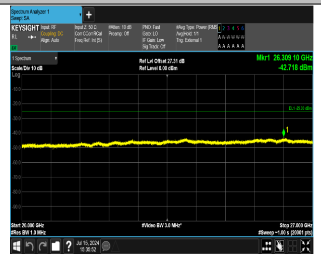
41(2555-2655)-41(2555-2655)-20MHz-20MHz-QPSK-QPS K-40942-41140-100RB#0-100RB#0-20000~27000MHz-PA
