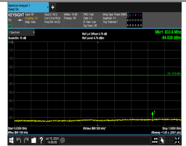
41(2555-2655)-41(2555-2655)-20MHz-20MHz-QPSK-QPS K-40340-40538-1RB#99-0RB#0-30~1000MHz-PASS
