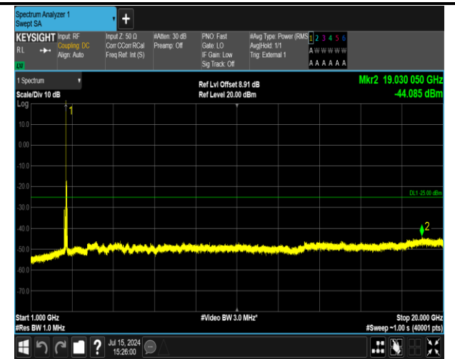
41(2555-2655)-41(2555-2655)-20MHz-20MHz-16QAM-16 QAM-40942-41140-1RB#0-ORB#0-1000~20000MHz-PASS
