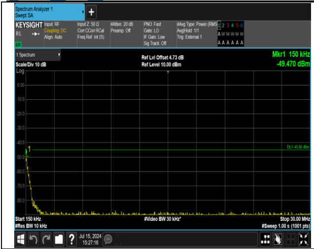
41(2555-2655)-41(2555-2655)-20MHz-20MHz-QPSK-QPS K-40942-41140-1RB#99-ORB#0-0.15~30MHz-PASS
