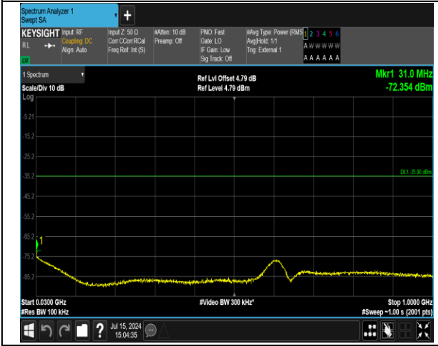
41(2555-2655)-41(2555-2655)-20MHz-20MHz-QPSK-QPS K-40340-40538-100RB#0-100RB#0-30~1000MHz-PASS
