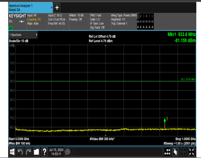
41(2555-2655)-41(2555-2655)-20MHz-20MHz-QPSK-QPS K-40340-40538-1RB#0-0RB#0-30~1000MHz-PASS
