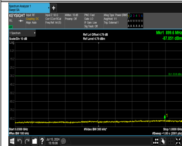
41(2555-2655)-41(2555-2655)-20MHz-20MHz-QPSK-QPS K-40641-40839-1RB#0-1RB#99-30~1000MHz-PASS
