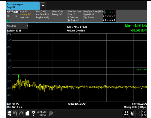
41(2555-2655)-41(2555-2655)-20MHz-20MHz-QPSK-QPS K-40340-40538-1RB#99-0RB#0-0.009~0.15MHz-PASS
