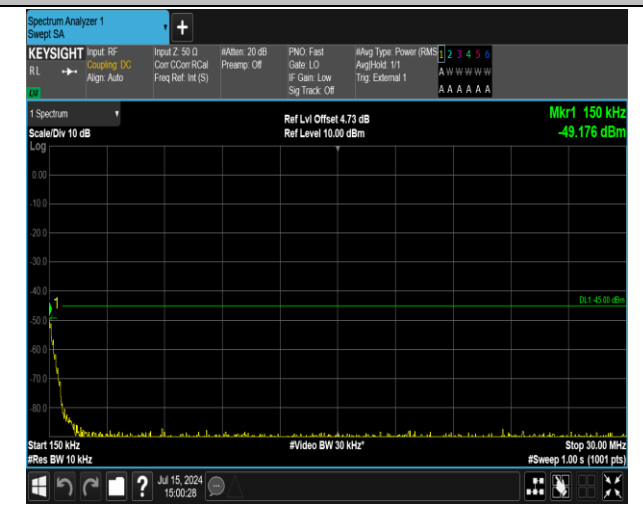
41(2555-2655)-41(2555-2655)-20MHz-20MHz-QPSK-QPS K-40340-40538-1RB#0-1RB#99-0.15~30MHz-PASS
