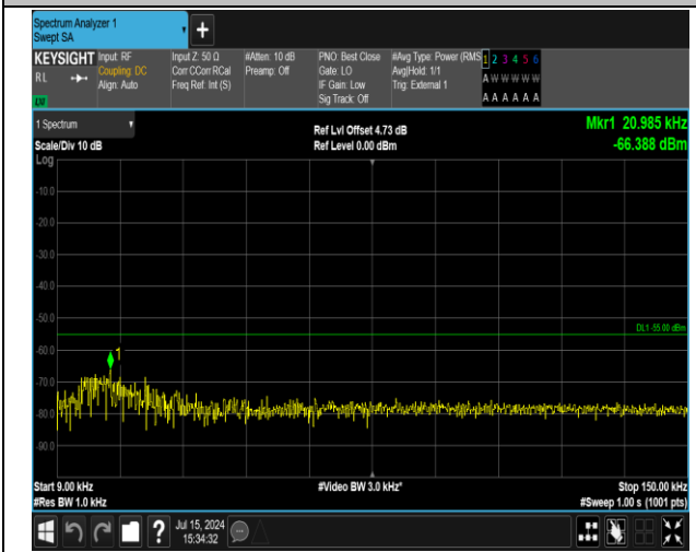
41(2555-2655)-41(2555-2655)-20MHz-20MHz-QPSK-QPS K-40942-41140-100RB#0-100RB#0-0.009~0.15MHz-PAS
