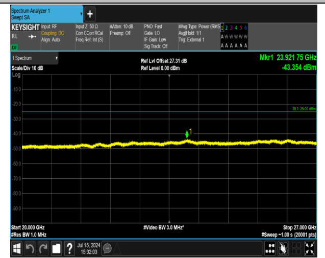
41(2555-2655)-41(2555-2655)-20MHz-20MHz-QPSK-QPS K-40942-41140-1RB#0-1RB#99-20000~27000MHz-PASS
