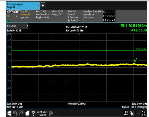
41(2555-2655)-41(2555-2655)-20MHz-20MHz-QPSK-QPS K-40641-40839-100RB#0-100RB#0-20000~27000MHz-PA SS
