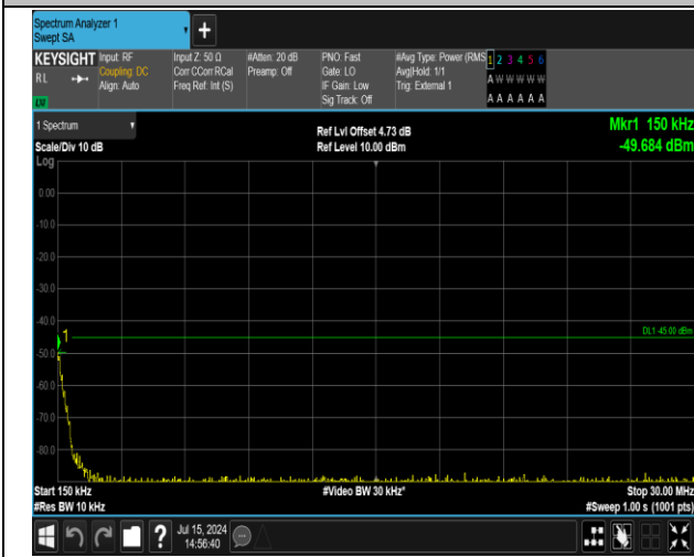
41(2555-2655)-41(2555-2655)-20MHz-20MHz-QPSK-QPS K-40340-40538-1RB#99-0RB#0-0.15~30MHz-PASS
