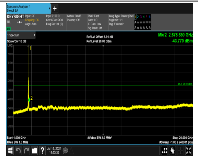
41(2555-2655)-41(2555-2655)-20MHz-20MHz-QPSK-QPS K-40340-40538-1RB#0-0RB#0-1000~20000MHz-PASS
