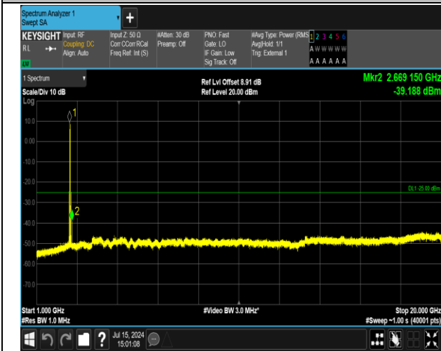
41(2555-2655)-41(2555-2655)-20MHz-20MHz-QPSK-QPS K-40340-40538-1RB#0-1RB#99-1000~20000MHz-PASS
