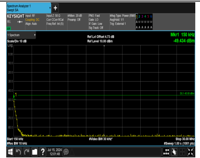
41(2555-2655)-41(2555-2655)-20MHz-5MHz-16QAM-16Q AM-40340-40457-100RB#0-25RB#0-0.15~30MHz-PASS
