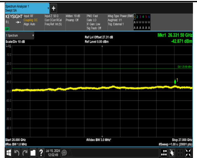
41(2555-2655)-41(2555-2655)-20MHz-5MHz-16QAM-16Q AM-40340-40457-100RB#0-25RB#0-20000~27000MHz-PA SS
