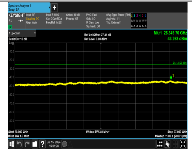
41(2555-2655)-41(2555-2655)-20MHz-20MHz-QPSK-QPS K-40340-40538-1RB#0-1RB#99-20000~27000MHz-PASS
