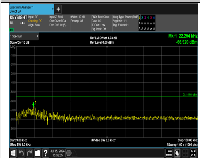
41(2555-2655)-41(2555-2655)-20MHz-20MHz-16QAM-16 QAM-40942-41140-1RB#0-1RB#99-0.009~0.15MHz-PASS
