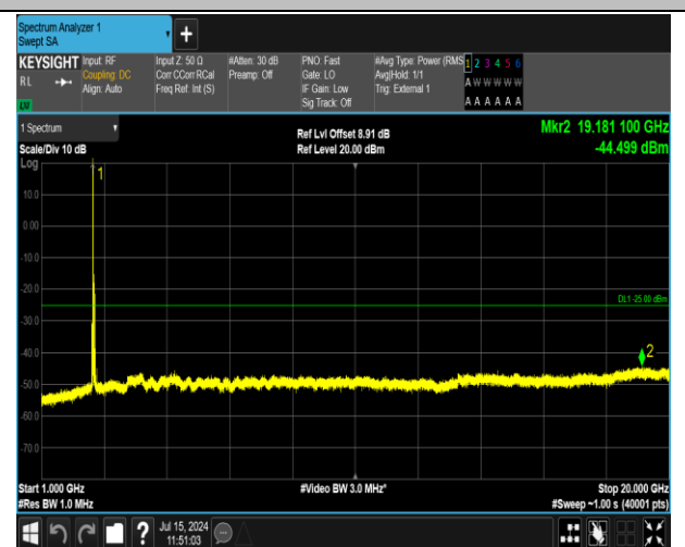
41(2555-2655)-41(2555-2655)-20MHz-5MHz-16QAM-16Q AM-40340-40457-1RB#0-0RB#0-1000~20000MHz-PASS
