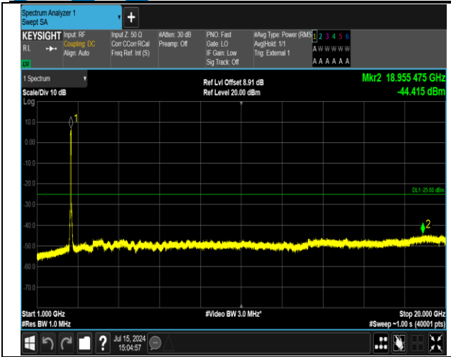
41(2555-2655)-41(2555-2655)-20MHz-20MHz-QPSK-QPS K-40340-40538-100RB#0-100RB#0-1000~20000MHz-PA SS
