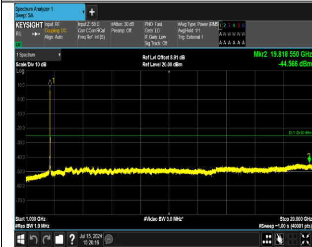
41(2555-2655)-41(2555-2655)-20MHz-20MHz-QPSK-QPS K-40641-40839-100RB#0-100RB#0-1000~20000MHz-PA SS
