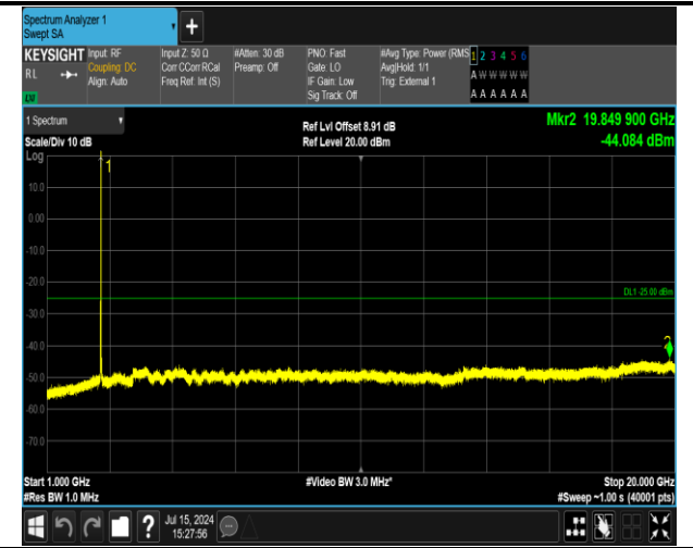
41(2555-2655)-41(2555-2655)-20MHz-20MHz-QPSK-QPS K-40942-41140-1RB#99-ORB#0-1000~20000MHz-PASS
