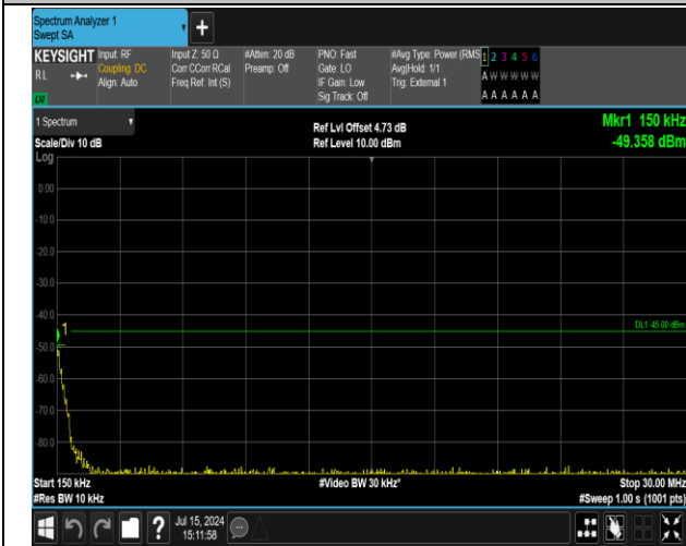
41(2555-2655)-41(2555-2655)-20MHz-20MHz-QPSK-QPS K-40641-40839-1RB#99-0RB#0-0.15~30MHz-PASS
