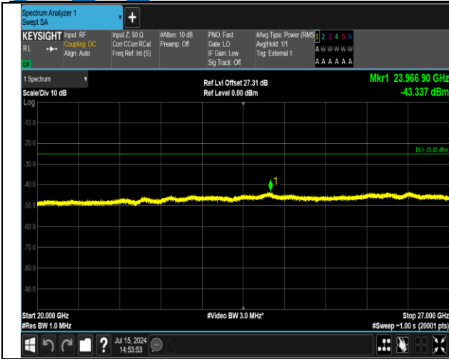
41(2555-2655)-41(2555-2655)-20MHz-20MHz-QPSK-QPS K-40340-40538-1RB#0-0RB#0-20000~27000MHz-PASS
