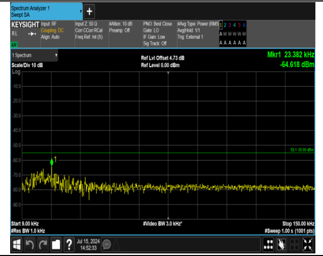
41(2555-2655)-41(2555-2655)-20MHz-20MHz-QPSK-QPS K-40340-40538-1RB#0-0RB#0-0.009~0.15MHz-PASS
