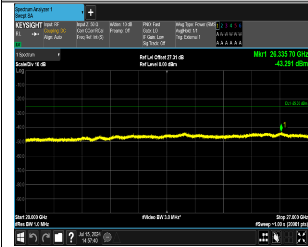
41(2555-2655)-41(2555-2655)-20MHz-20MHz-QPSK-QPS K-40340-40538-1RB#99-0RB#0-20000~27000MHz-PASS
