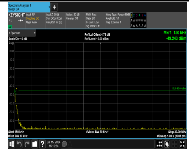
41(2555-2655)-41(2555-2655)-20MHz-20MHz-QPSK-QPS K-40641-40839-100RB#0-100RB#0-0.15~30MHz-PASS
