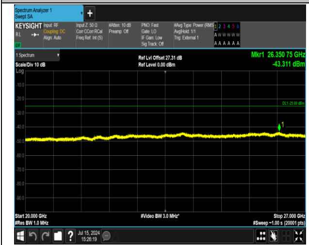
41(2555-2655)-41(2555-2655)-20MHz-20MHz-16QAM-16 QAM-40942-41140-1RB#0-ORB#0-20000~27000MHz-PASS
