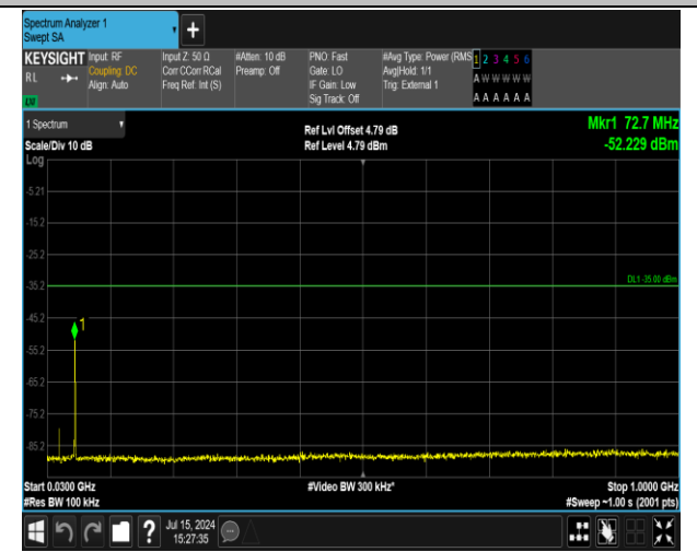
41(2555-2655)-41(2555-2655)-20MHz-20MHz-QPSK-QPS K-40942-41140-1RB#99-ORB#0-30~1000MHz-PASS
