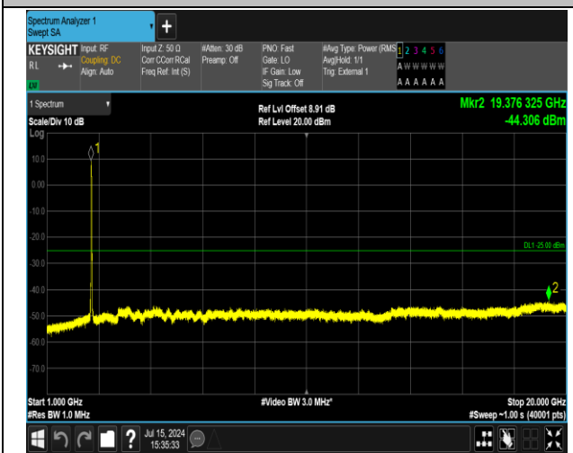
41(2555-2655)-41(2555-2655)-20MHz-20MHz-QPSK-QPS K-40942-41140-100RB#0-100RB#0-1000~20000MHz-PA
