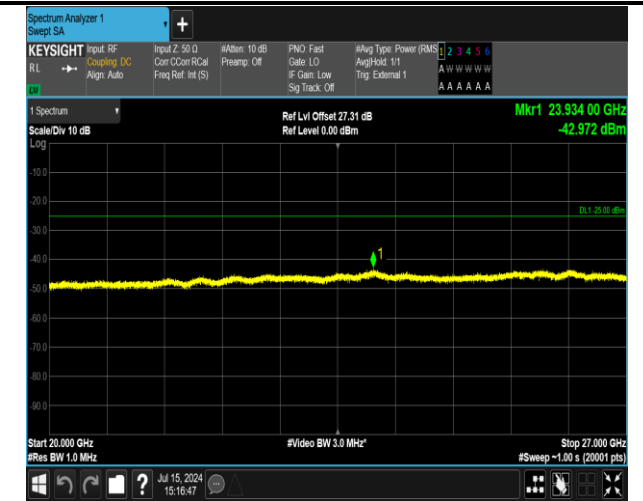
41(2555-2655)-41(2555-2655)-20MHz-20MHz-QPSK-QPS K-40641-40839-1RB#0-1RB#99-20000~27000MHz-PASS
