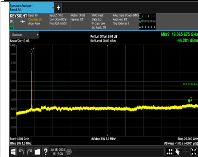
41(2555-2655)-41(2555-2655)-20MHz-20MHz-QPSK-QPS K-40641-40839-1RB#0-1RB#99-1000~20000MHz-PASS
