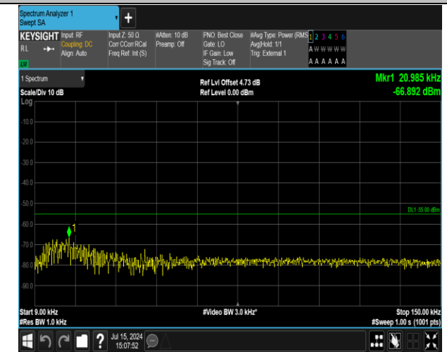
41(2555-2655)-41(2555-2655)-20MHz-20MHz-QPSK-QPS
