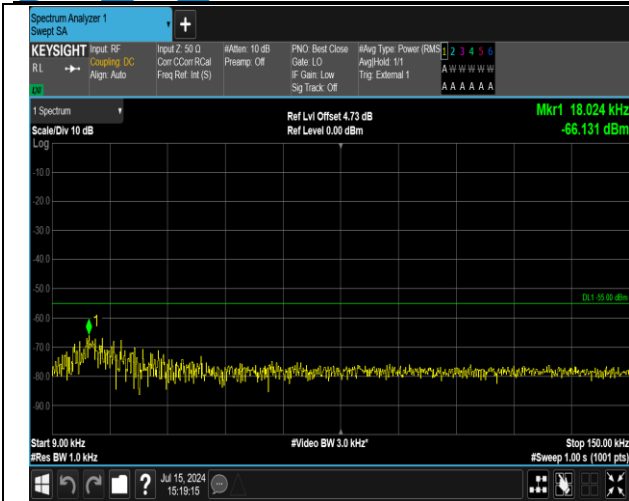
41(2555-2655)-41(2555-2655)-20MHz-20MHz-QPSK-QPS K-40641-40839-100RB#0-100RB#0-0.009~0.15MHz-PAS S
