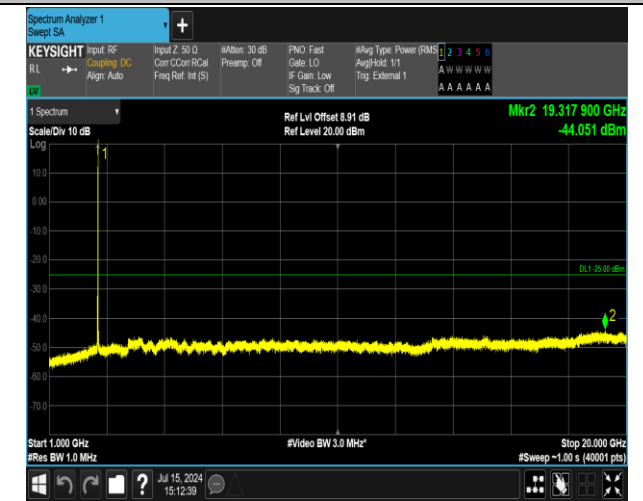
41(2555-2655)-41(2555-2655)-20MHz-20MHz-QPSK-QPS K-40641-40839-1RB#99-0RB#0-1000~20000MHz-PASS
