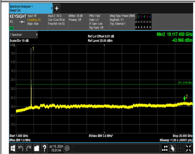
41(2555-2655)-41(2555-2655)-20MHz-20MHz-QPSK-QPS K-40942-41140-1RB#0-1RB#99-1000~20000MHz-PASS
