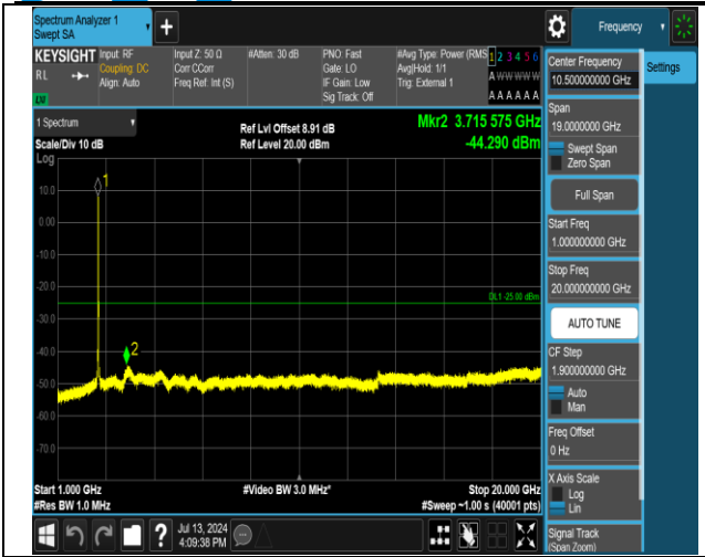
38-38-20MHz-20MHz-QPSK-QPSK-37901-38099-100RB# 0-100RB#0-1000~20000MHz-PASS
