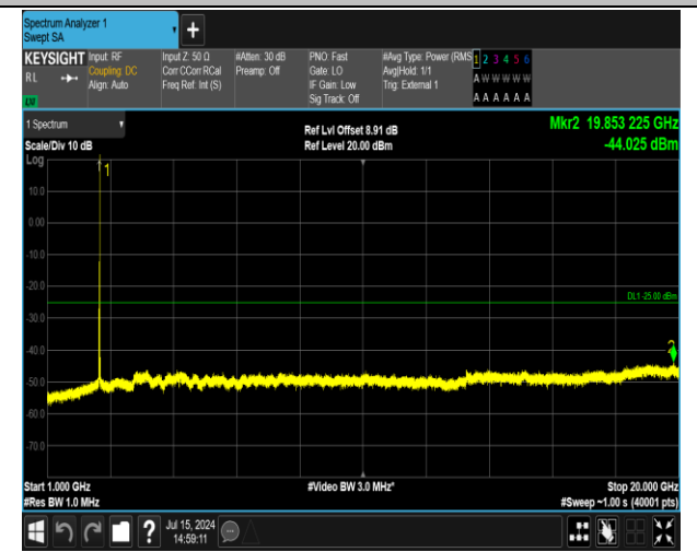
41(2555-2655)-41(2555-2655)-20MHz-20MHz-16QAM-16 QAM-40340-40538-1RB#99-0RB#0-1000~20000MHz-PAS S
