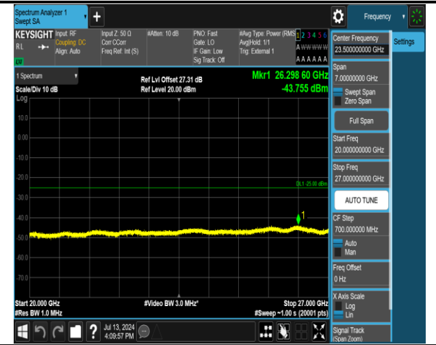
38-38-20MHz-20MHz-QPSK-QPSK-37901-38099-100RB# 0-100RB#0-20000~27000MHz-PASS
