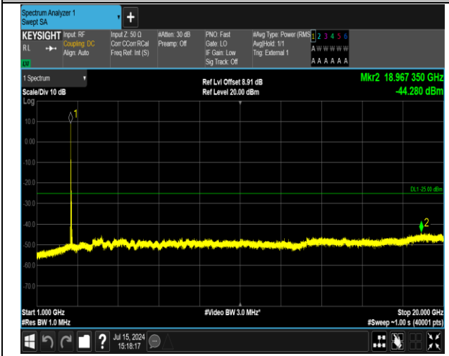
41(2555-2655)-41(2555-2655)-20MHz-20MHz-16QAM-16 QAM-40641-40839-1RB#0-1RB#99-1000~20000MHz-PA SS
