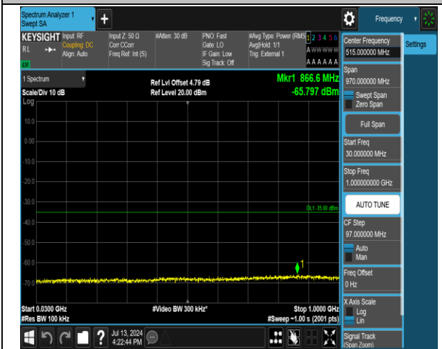
38-38-20MHz-20MHz-QPSK-QPSK-37952-38150-100RB# 0-100RB#0-30~1000MHz-PASS
