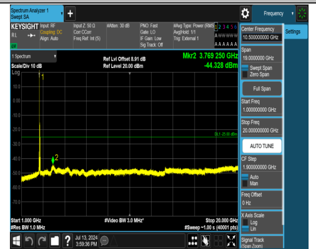
38-38-20MHz-20MHz-QPSK-QPSK-37901-38099-1RB#0-0 RB#0-1000~20000MHz-PASS
