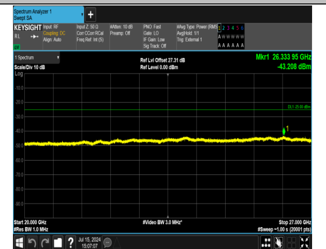
41(2555-2655)-41(2555-2655)-20MHz-20MHz-16QAM-16 QAM-40340-40538-100RB#0-100RB#0-20000~27000MHz
