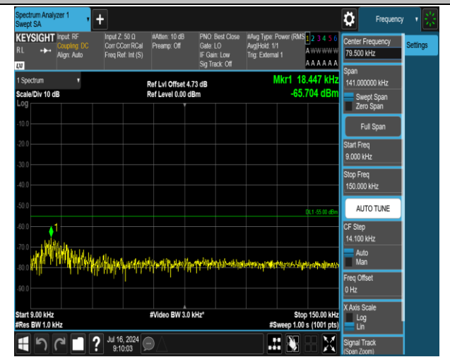
38-38-20MHz-20MHz-QPSK-QPSK-37952-38150-1RB#99-0RB#0-0.009~0.15MHz-PASS
