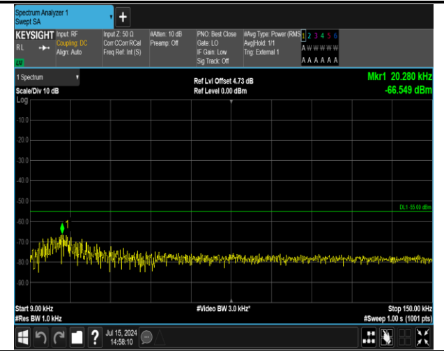
41(2555-2655)-41(2555-2655)-20MHz-20MHz-16QAM-16 QAM-40340-40538-1RB#99-0RB#0-0.009~0.15MHz-PASS
