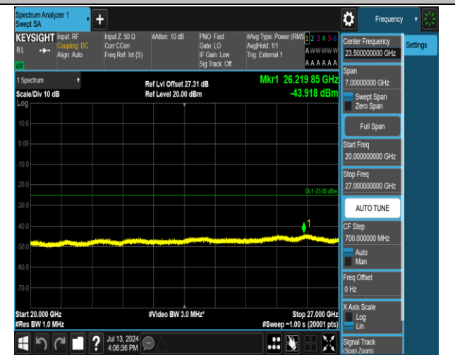
38-38-20MHz-20MHz-QPSK-QPSK-37901-38099-1RB#0-1RB#99-20000~27000MHz-PASS
