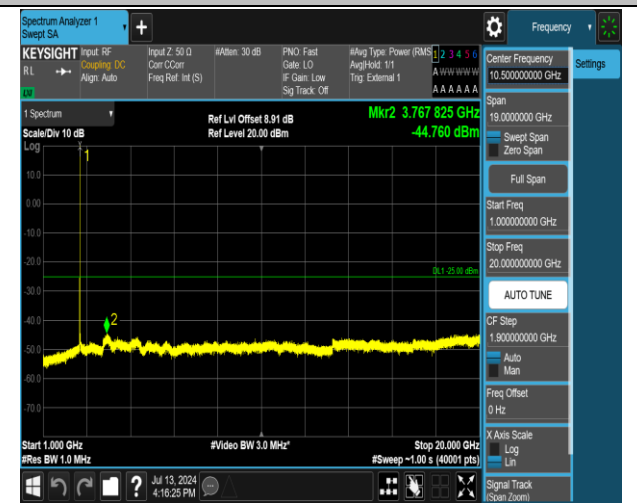
38-38-20MHz-20MHz-QPSK-QPSK-37952-38150-1RB#99-0RB#0-1000~20000MHz-PASS
