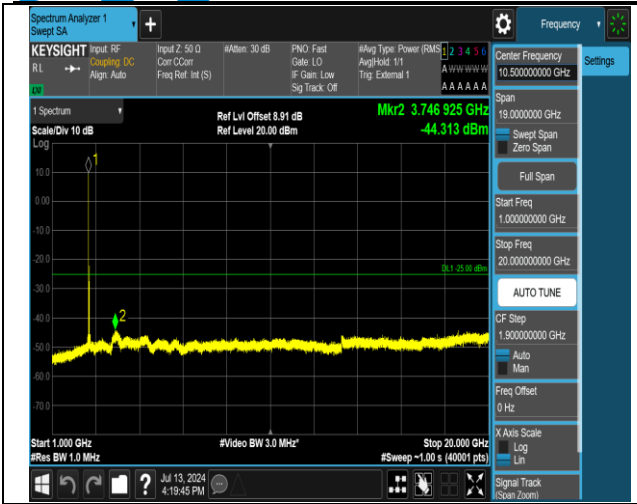
38-38-20MHz-20MHz-QPSK-QPSK-37952-38150-1RB#0-1RB#99-1000~20000MHz-PASS
