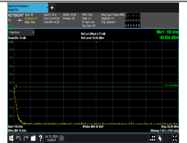
41(2555-2655)-41(2555-2655)-20MHz-20MHz-16QAM-16 QAM-40340-40538-100RB#0-100RB#0-0.15~30MHz-PAS S
