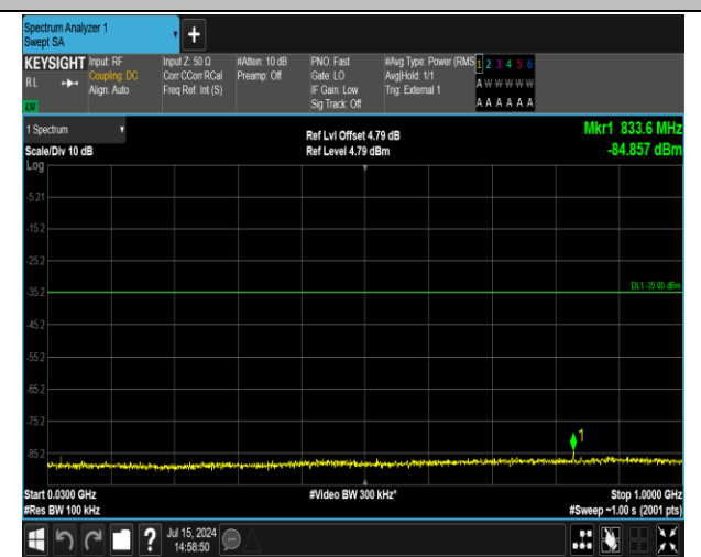
41(2555-2655)-41(2555-2655)-20MHz-20MHz-16QAM-16 QAM-40340-40538-1RB#99-0RB#0-30~1000MHz-PASS
