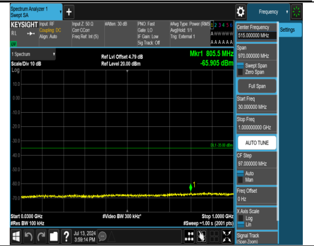
38-38-20MHz-20MHz-QPSK-QPSK-37901-38099-1RB#0-RB#0-30~1000MHz-PASS
