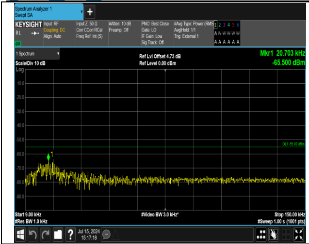
41(2555-2655)-41(2555-2655)-20MHz-20MHz-16QAM-16 QAM-40641-40839-1RB#0-1RB#99-0.009~0.15MHz-PAS S
