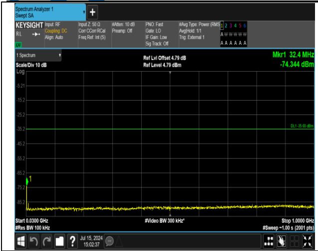
41(2555-2655)-41(2555-2655)-20MHz-20MHz-16QAM-16 QAM-40340-40538-1RB#0-1RB#99-30~1000MHz-PASS
