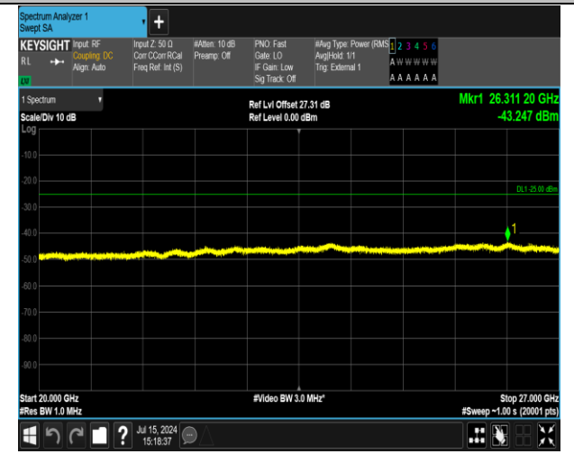
41(2555-2655)-41(2555-2655)-20MHz-20MHz-16QAM-16 QAM-40641-40839-1RB#0-1RB#99-20000~27000MHz-PA SS
