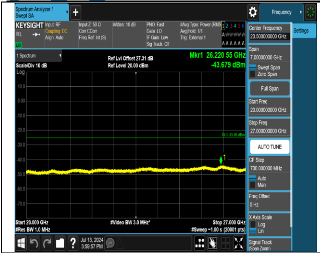
38-38-20MHz-20MHz-QPSK-QPSK-37901-38099-1RB#0-ORB#0-20000~27000MHz-PASS
