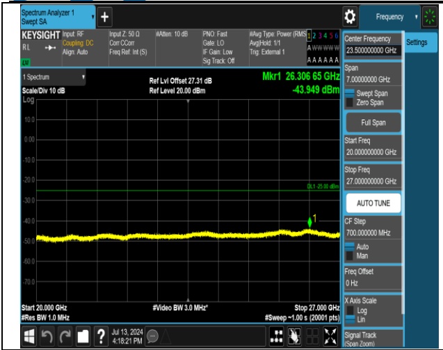
38-38-20MHz-20MHz-16QAM-16QAM-37952-38150-1RB #99-0RB#0-20000~27000MHz-PASS
