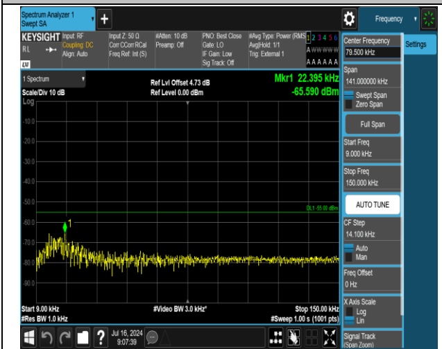
38-38-20MHz-20MHz-QPSK-QPSK-37901-38099-100RB# 0-100RB#0-0.009~0.15MHz-PASS
