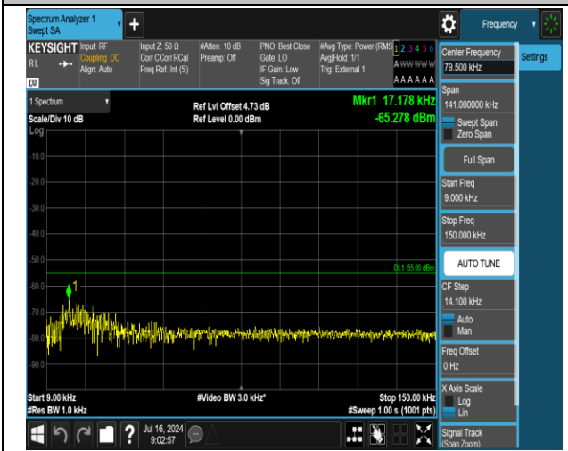
38-38-20MHz-20MHz-QPSK-QPSK-37850-38048-100RB# 0-100RB#0-0.009~0.15MHz-PASS
