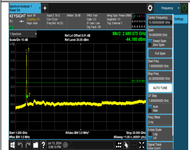
38-38-20MHz-20MHz-QPSK-QPSK-37850-38048-100RB# 0-100RB#0-1000~20000MHz-PASS
