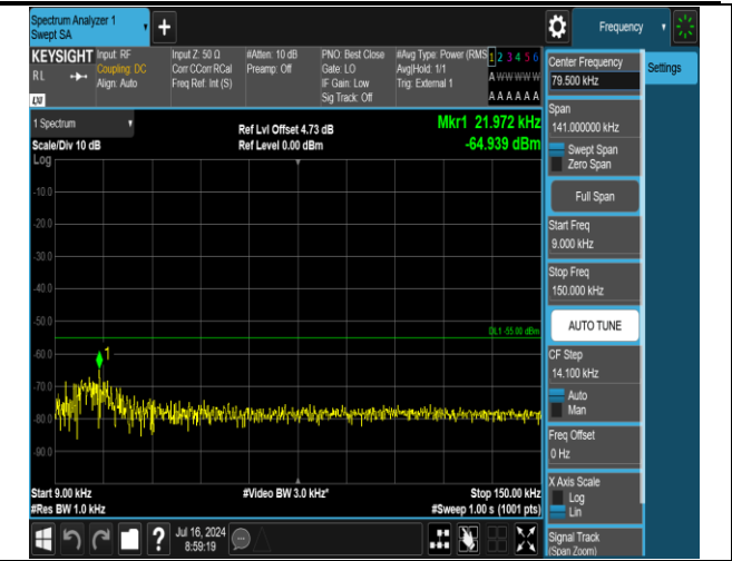
38-38-20MHz-20MHz-QPSK-QPSK-37850-38048-1RB#0-0-RB#0-0.009~0.15MHz-PASS
