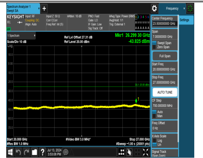
38-38-20MHz-20MHz-QPSK-QPSK-37850-38048-1RB#0-1RB#99-20000~27000MHz-PASS
