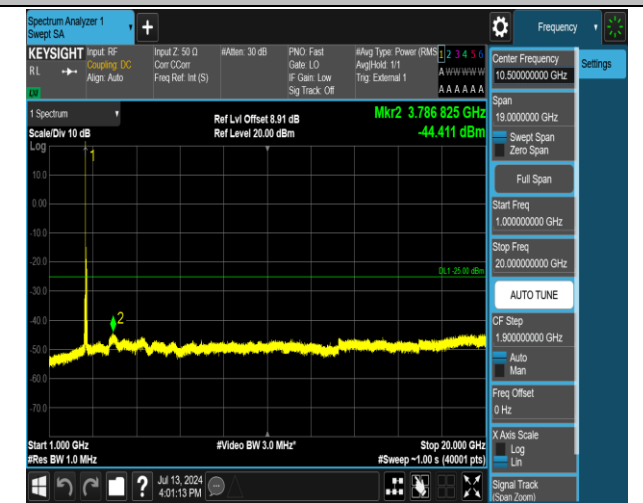
38-38-20MHz-20MHz-16QAM-16QAM-37901-38099-1RB# 0-0-ORB#0-1000~20000MHz-PASS
