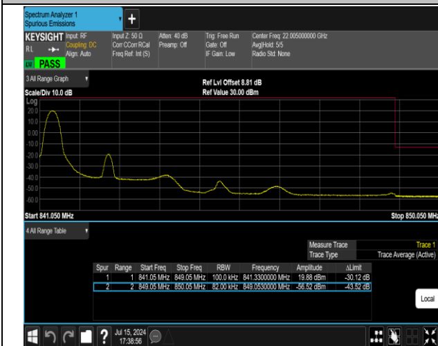
5-5-3MHz-5MHz-16QAM@16QAM-16QAM@16QAM-2058
