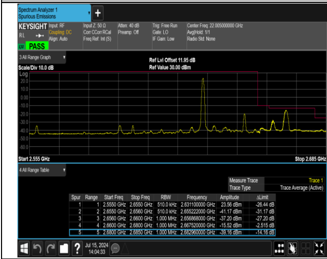
41(2555-2655)-41(2555-2655)-20MHz-5MHz-16QAM@16
