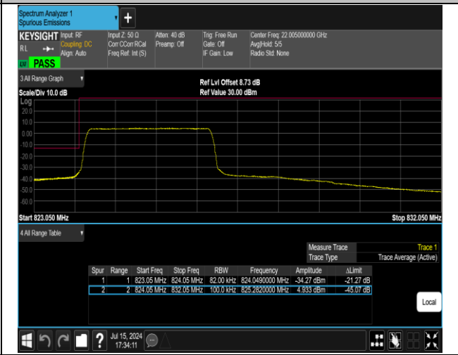
5-5-3MHz-5MHz-16QAM@16QAM-16QAM@16QAM-204
