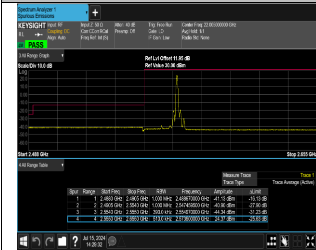
41(2555-2655)-41(2555-2655)-20MHz-20MHz-QPSK@QP
