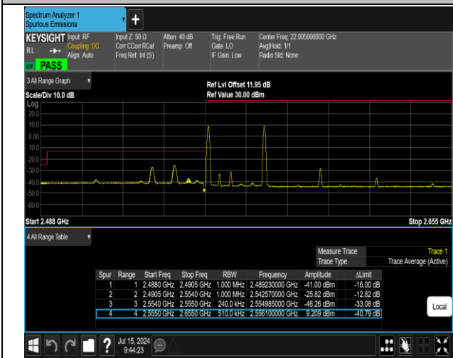
41(2555-2655)-41(2555-2655)-5MHz-20MHz-16QAM@16 QAM-16QAM@16QAM-40273-40390-1RB#0@25RB#0-1R
