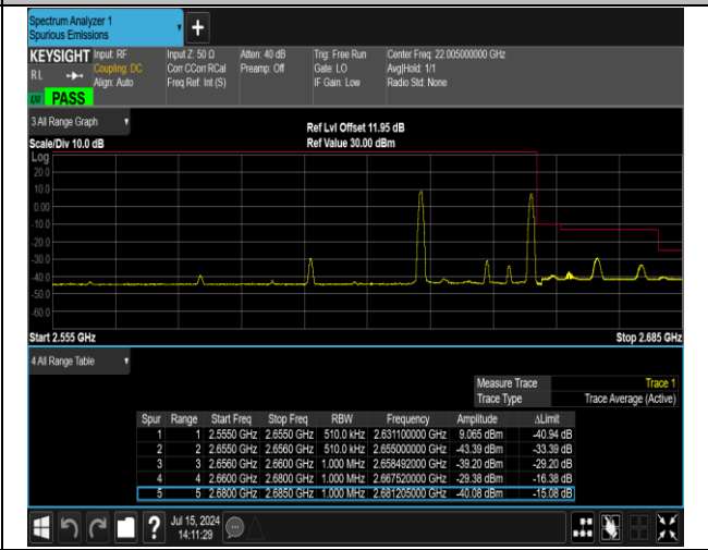
41(2555-2655)-41(2555-2655)-20MHz-5MHz-16QAM@16
