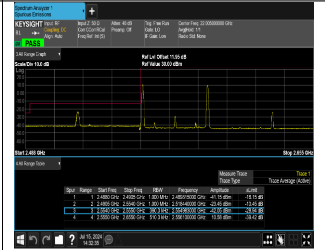
41(2555-2655)-41(2555-2655)-20MHz-20MHz-QPSK@Q PSK-QPSK@QPSK-40340-40538-1RB#0@100RB#0-1R B#99@100RB#0-PASS
