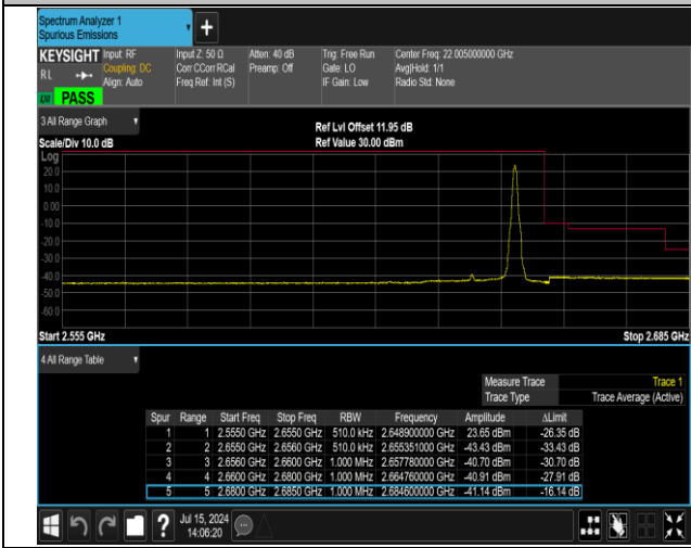
41(2555-2655)-41(2555-2655)-20MHz-5MHz-QPSK@QPS
