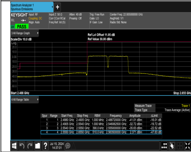
41(2555-2655)-41(2555-2655)-20MHz-20MHz-16QAM@16
