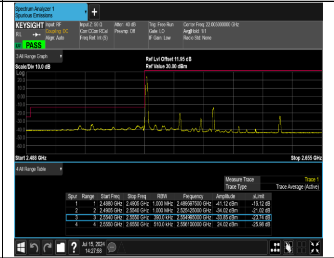
41(2555-2655)-41(2555-2655)-20MHz-20MHz-16QAM@16
