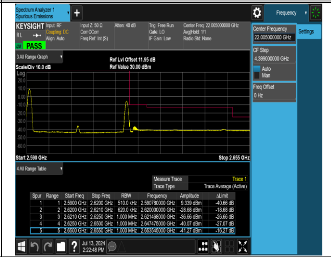
38-38-15MHz-15MHz-16QAM@16QAM-16QAM@16QAM
