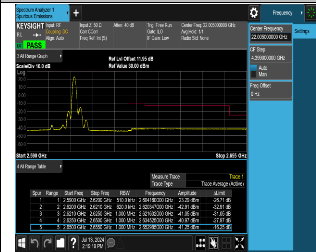
38025-38175-1RB#0@75RB#0-0RB#0@75RB#0-PASS
