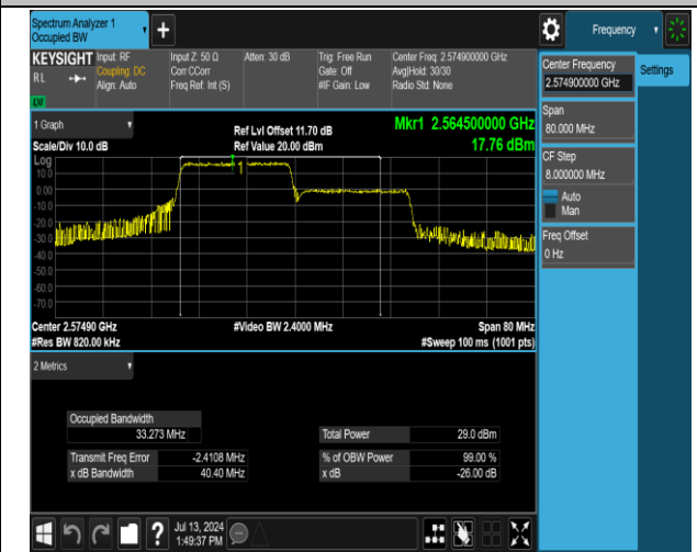
41(2555-2655)-41(2555-2655)-20MHz-20MHz-QPSK-QPS K-40340-40538-100RB#0-100RB#0-PASS
