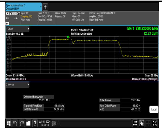
5-5-5MHz-10MHz-QPSK-QPSK-20428-20500-25RB#0-50RB#0-PASS
