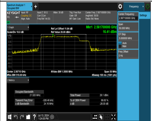
41(2555-2655)-41(2555-2655)-20MHz-5MHz-QPSK-QPSK -40340-40457-100RB#0-25RB#0-PASS
