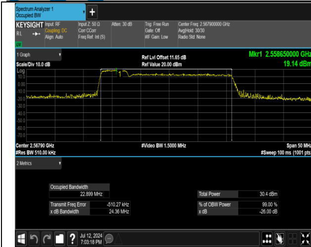
41(2555-2655)-41(2555-2655)-5MHz-20MHz-16QAM-16Q AM-40273-40390-25RB#0-100RB#0-PASS
