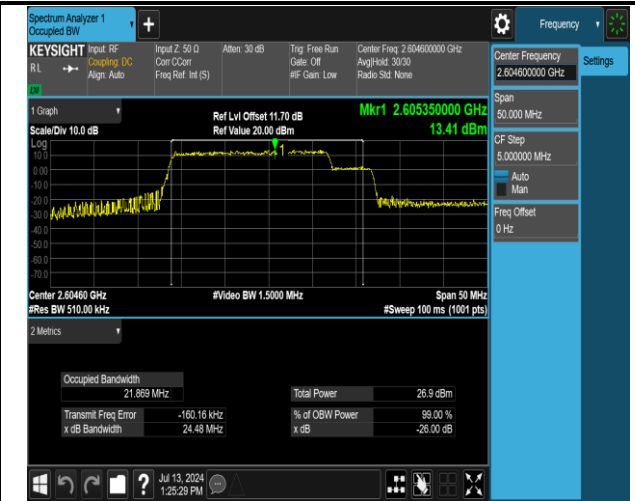
41(2555-2655)-41(2555-2655)-20MHz-5MHz-16QAM-16Q AM-40715-40832-100RB#0-25RB#0-PASS
