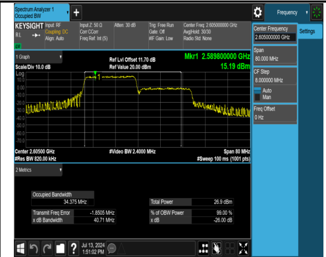
41(2555-2655)-41(2555-2655)-20MHz-20MHz-16QAM-16 QAM-40641-40839-100RB#0-100RB#0-PASS
