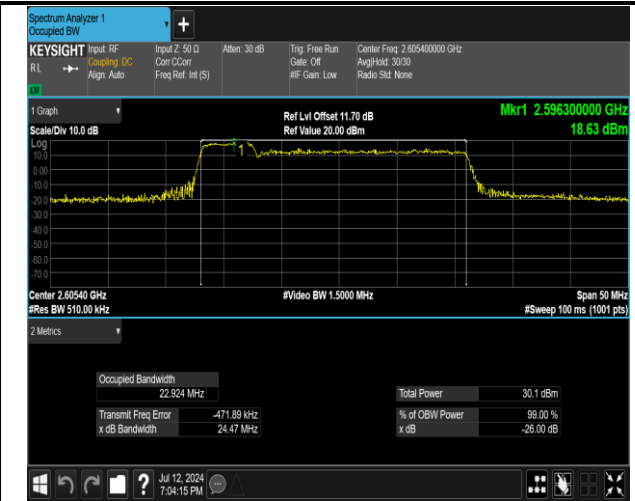
41(2555-2655)-41(2555-2655)-5MHz-20MHz-16QAM-16Q AM-40648-40765-25RB#0-100RB#0-PASS
