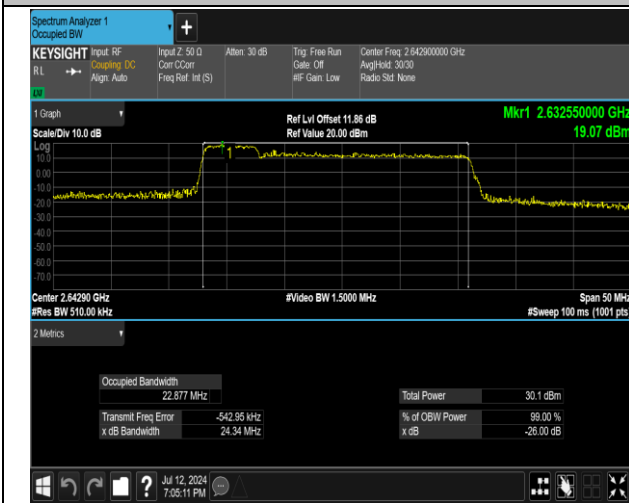
41(2555-2655)-41(2555-2655)-5MHz-20MHz-16QAM-16Q AM-41023-41140-25RB#0-100RB#0-PASS
