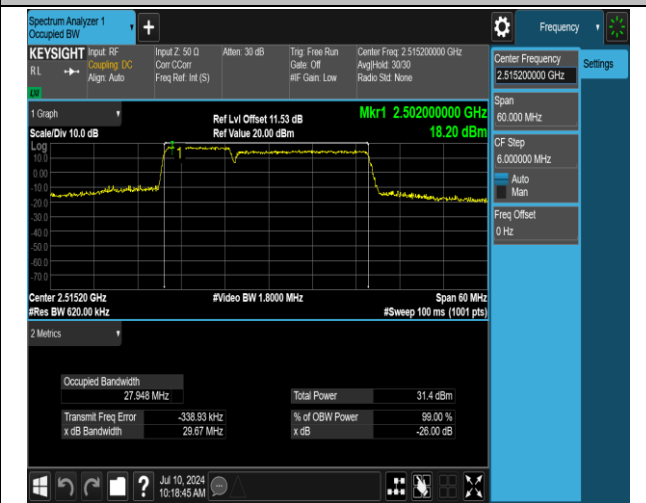
7-7-10MHz-20MHz-QPSK-QPSK-20805-20949-50RB#0-1 00RB#0-PASS
