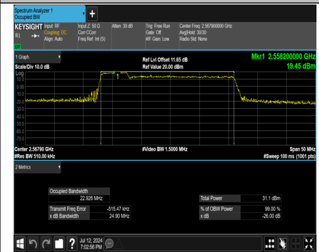
41(2555-2655)-41(2555-2655)-5MHz-20MHz-QPSK-QPSK -40273-40390-25RB#0-100RB#0-PASS
