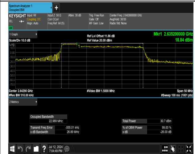
41(2555-2655)-41(2555-2655)-5MHz-20MHz-QPSK-QPSK -41023-41140-25RB#0-100RB#0-PASS
