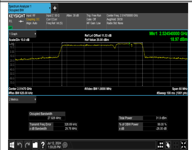
7-7-20MHz-10MHz-QPSK-QPSK-20850-20994-100RB#0- 50RB#0-PASS
