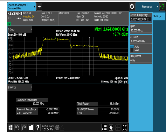
41(2555-2655)-41(2555-2655)-20MHz-20MHz-QPSK-QPS K-40942-41140-100RB#0-100RB#0-PASS
