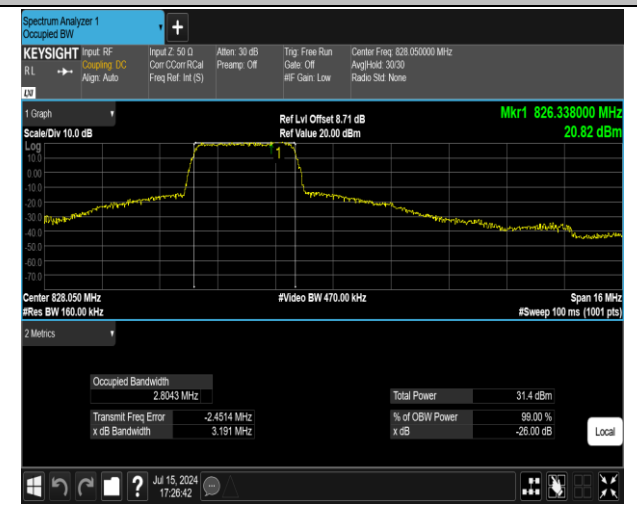
5-5-3MHz-5MHz-QPSK-QPSK-20416-20455-15RB#0-25R B#0-PASS
