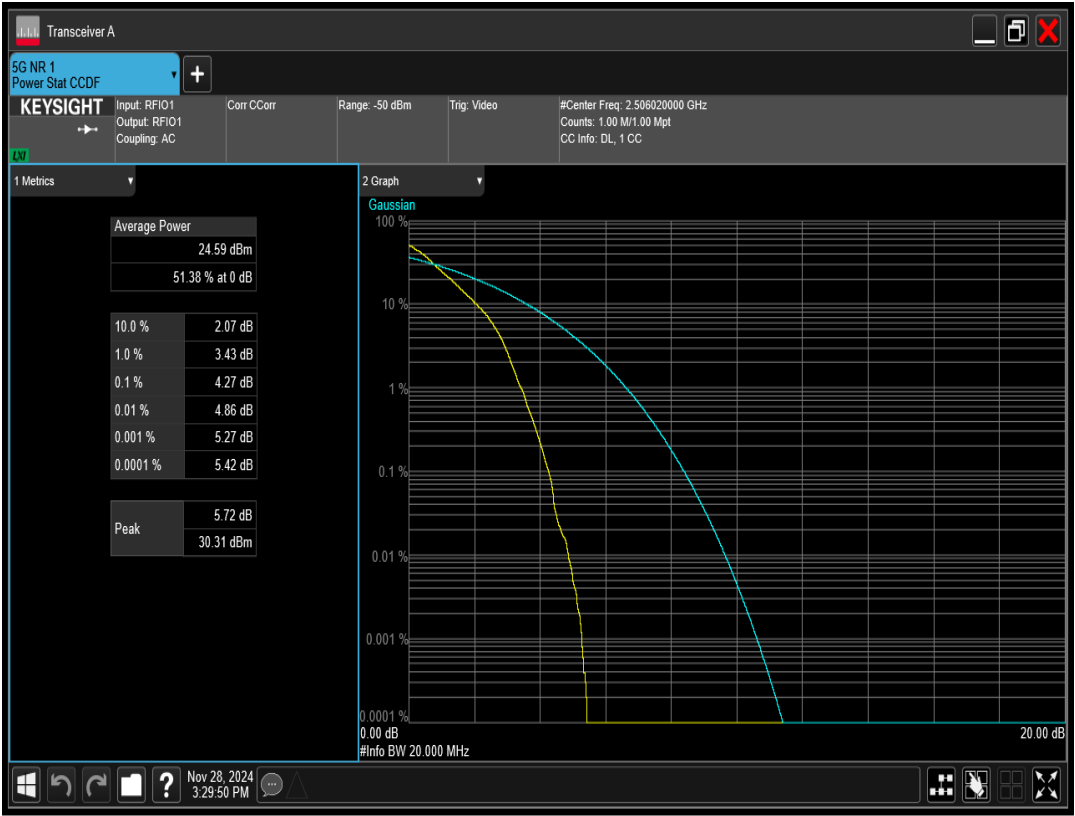
n41 SCS=30kHz DFT_BPSK BW=20MHz Channel=501204 RB=50@0
