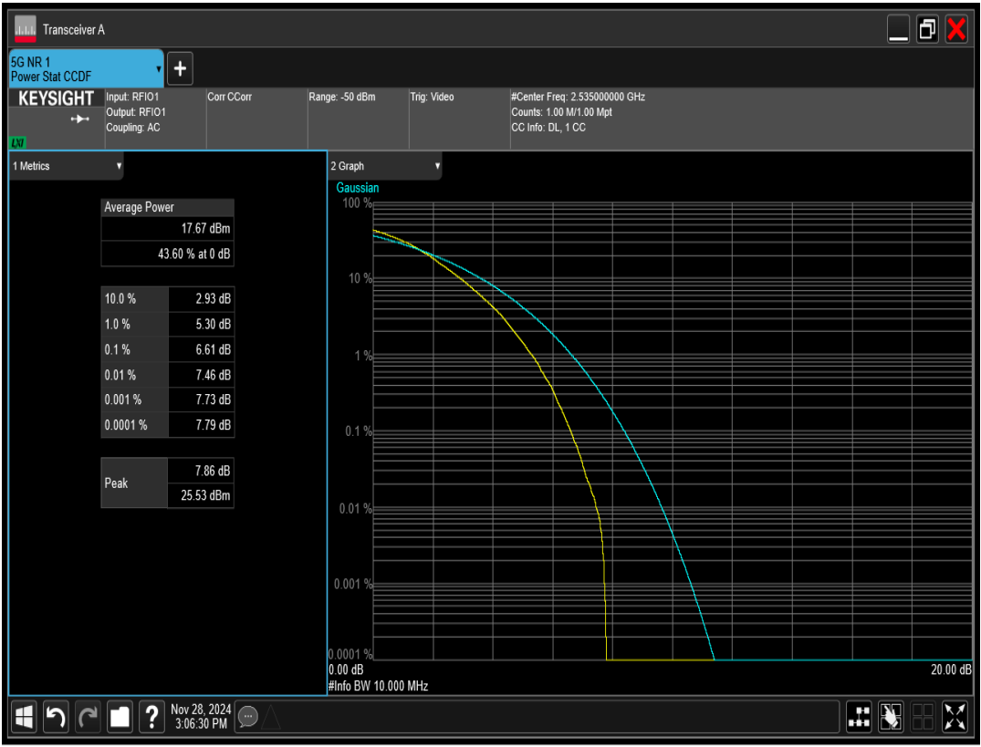
n7 SCS=15kHz DFT_QAM256 BW=10MHz Channel=507000 RB=50@0
