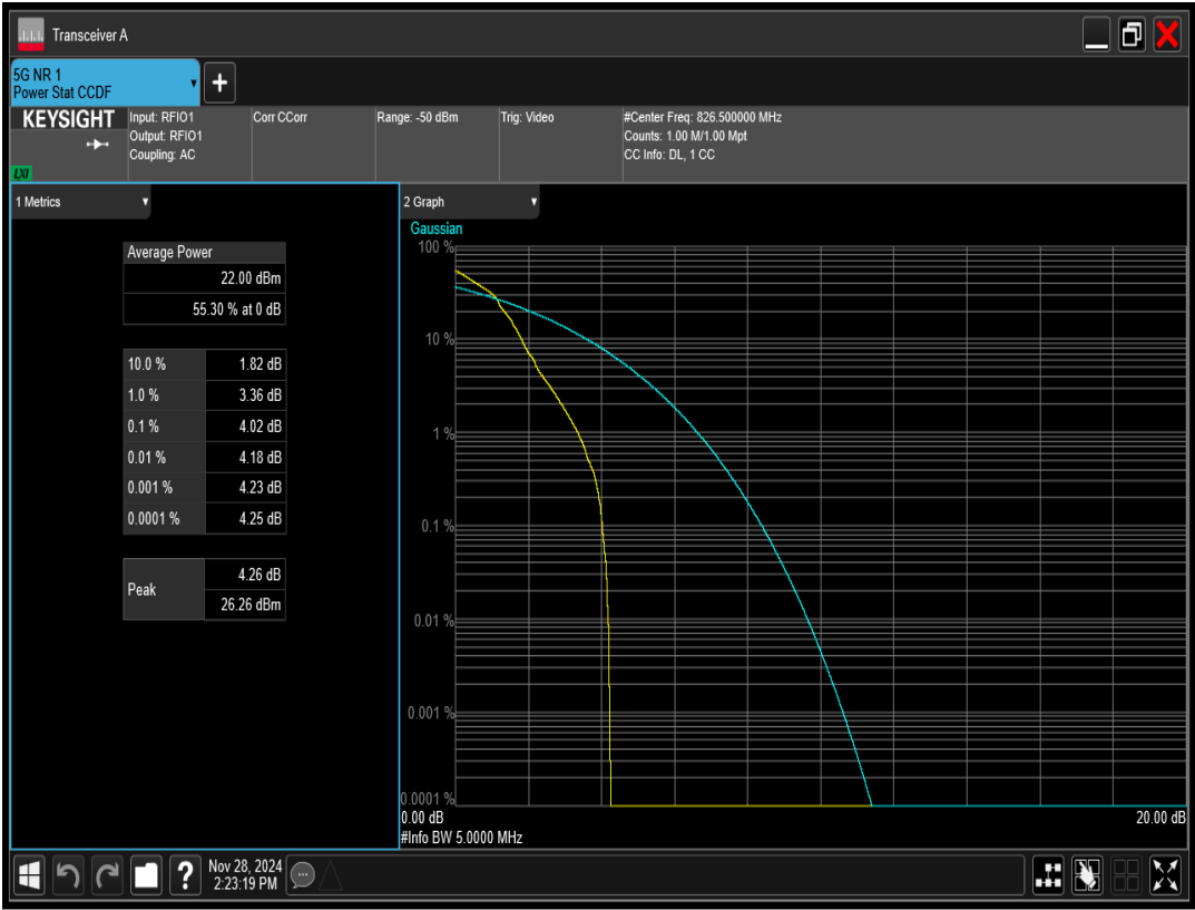
n5 SCS=15kHz DFT_BPSK BW=5MHz Channel=165300 RB=25@0
