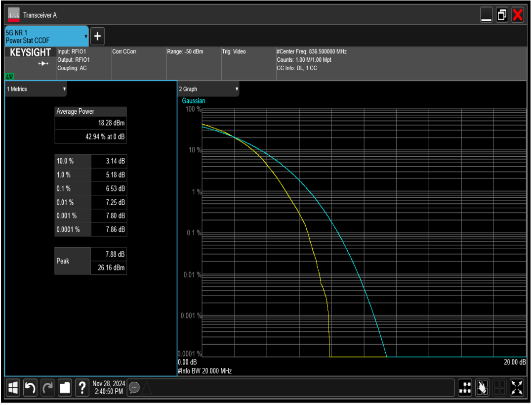
n5 SCS=15kHz DFT_QAM256 BW=20MHz Channel=167300 RB=100@0
