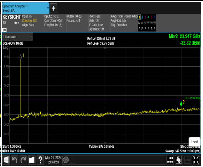
Band7-5MHz-QPSK-21100-1RB#0-Range2:1000~26500MHz
