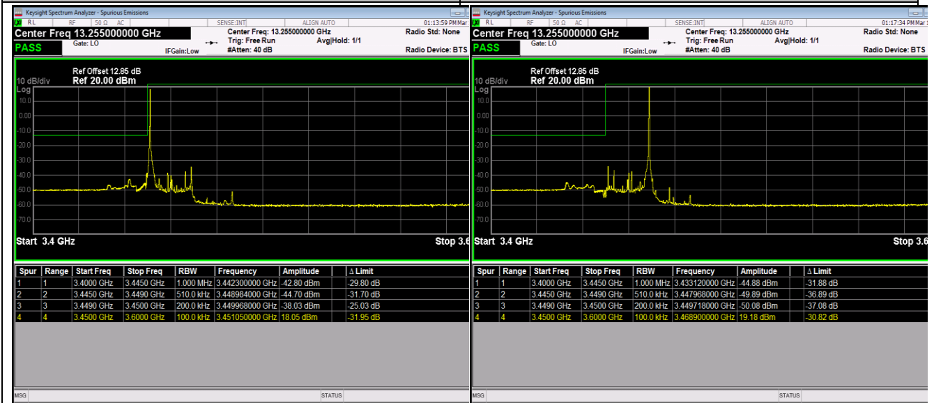
Band42_20MHz_QPSK_42990_1RB#99
