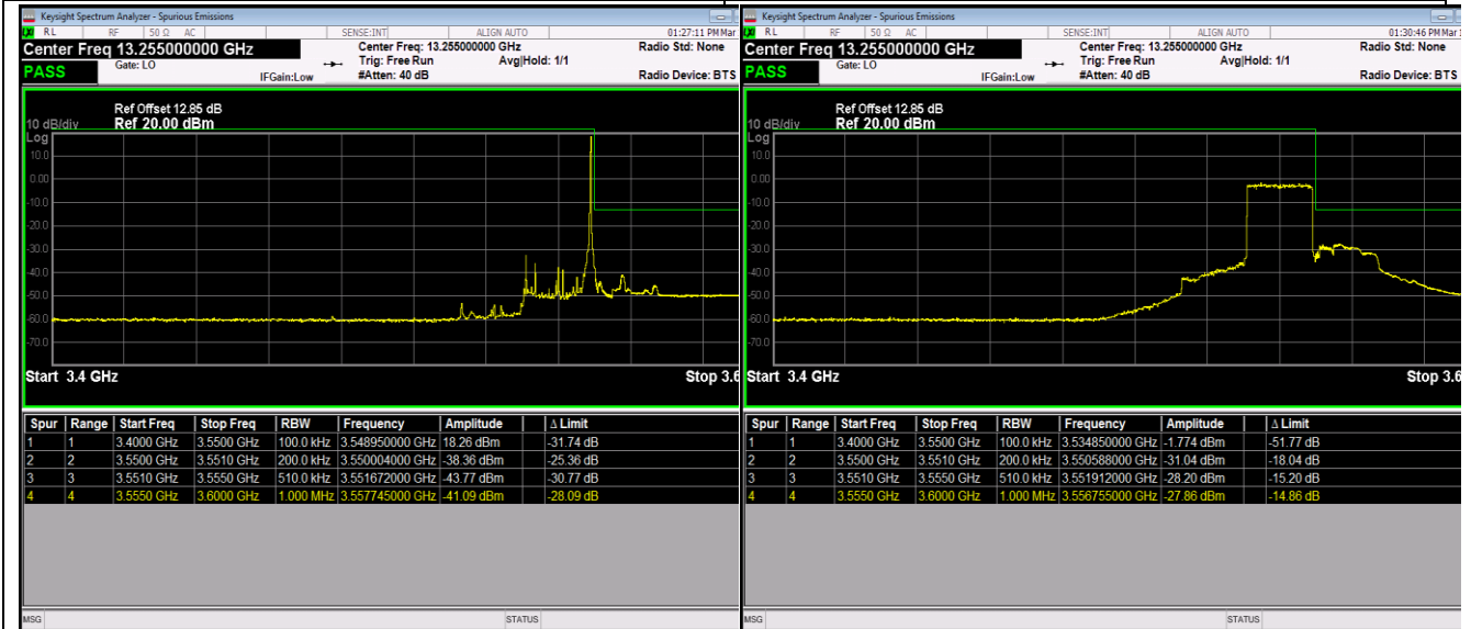
Band42_20MHz_QPSK_42990_1RB#99
