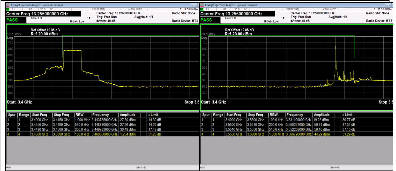
Band42_20MHz_QPSK_42190_100RB#0
