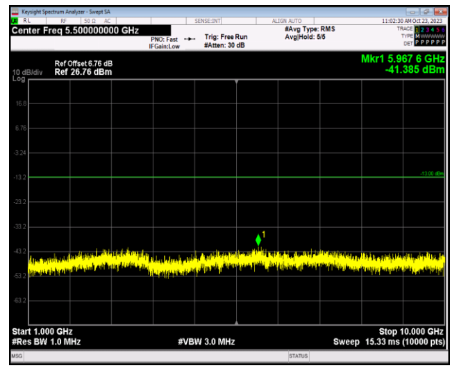
Band26-1.4MHz-QPSK-26697-1RB#0-Range2:1000~10000MHz
