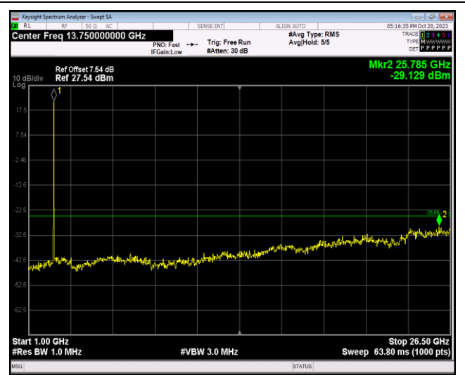
Band7-20MHz-QPSK-21350-1RB#0-Range2:1000~26500MHz
