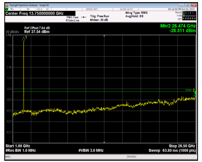
Band7-20MHz-16QAM-21350-1RB#0-Range2:1000~26500MHz
