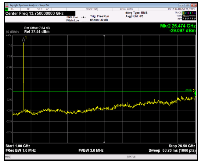
Band7-20MHz-QPSK-21100-1RB#0-Range2:1000~26500MHz
