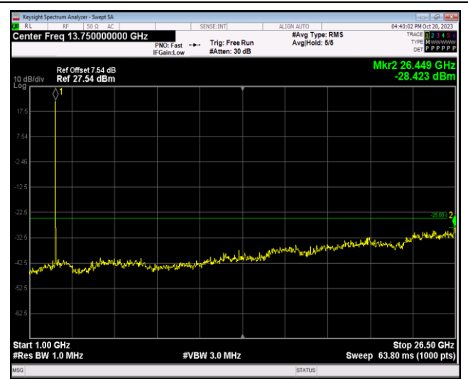
Band7-20MHz-QPSK-20850-1RB#0-Range2:1000~26500MHz
