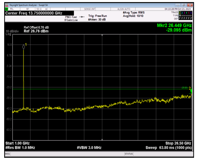
Band41-5MHz-QPSK-41215-1RB#0-Range2:1000~26500MHz
