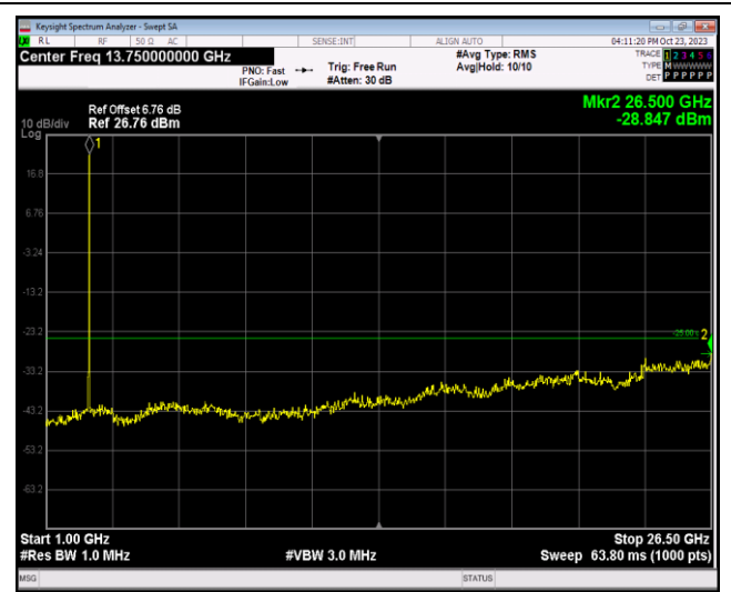
Band41-5MHz-16QAM-40065-1RB#0-Range2:1000~26500MHz
