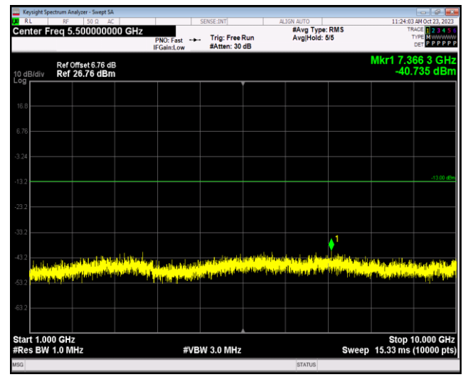
Band26-10MHz-QPSK-26740-1RB#0-Range2:1000~ 10000MHz
