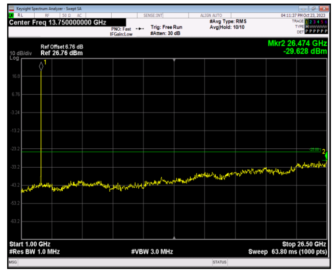
Band41-5MHz-64QAM-40065-1RB#0-Range2:1000~26500MHz
