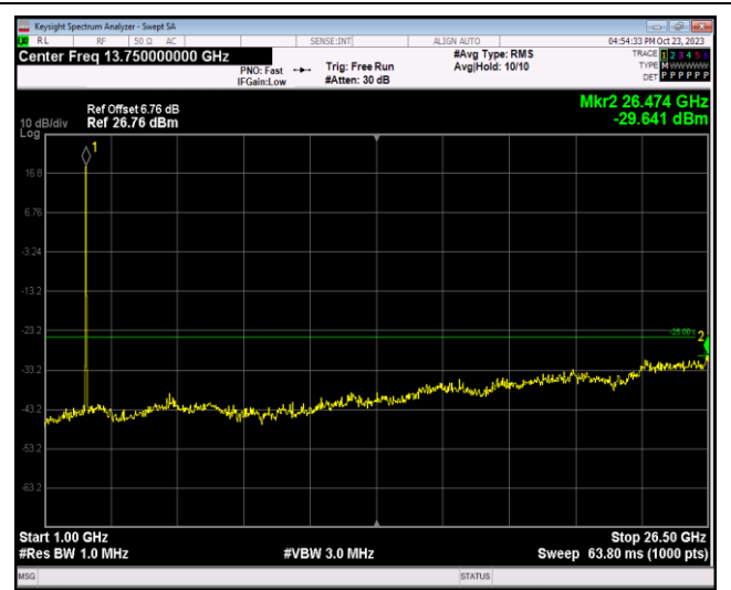
Band41-20MHz-QPSK-41140-1RB#0-Range2:1000~26500MHz
