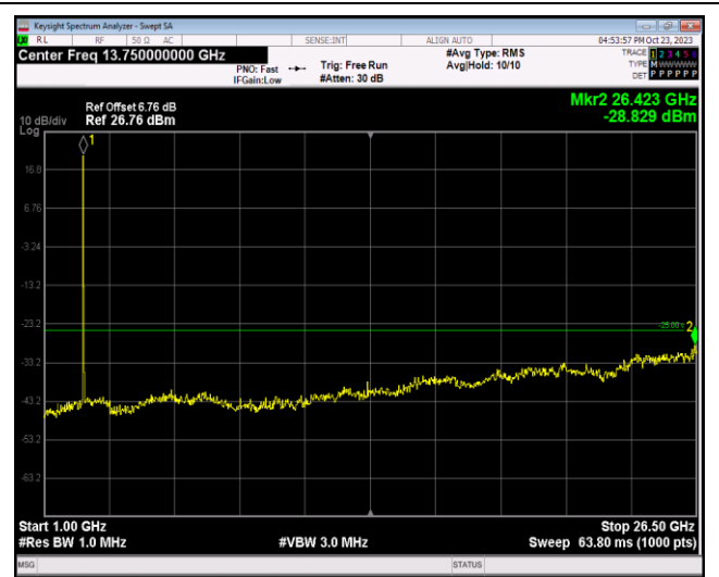
Band41-20MHz-16QAM-40640-1RB#0-Range2:1000~26500MHz
