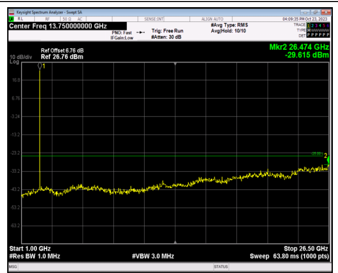
Band41-5MHz-QPSK-40640-1RB#0-Range2:1000~26500MHz
