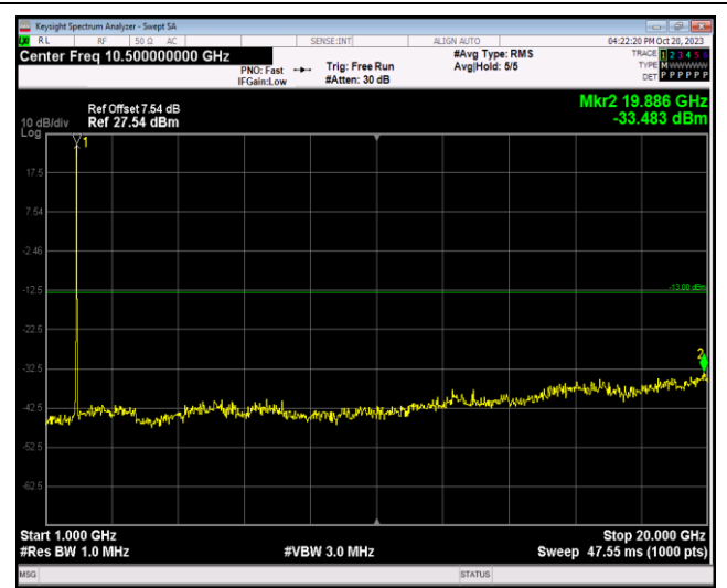
Band2-20MHz-64QAM-18700-1RB#0-Range2:1000~20000MHz
