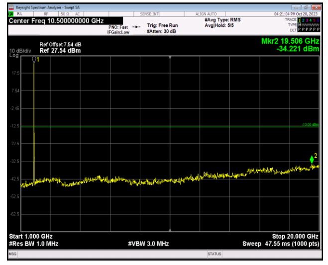
Band2-20MHz-64QAM-18900-1RB#0-Range2:1000~20000MHz
