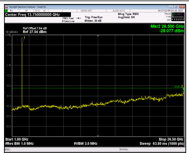
Band7-5MHz-QPSK-21100-1RB#0-Range2:1000~26 500MHz
