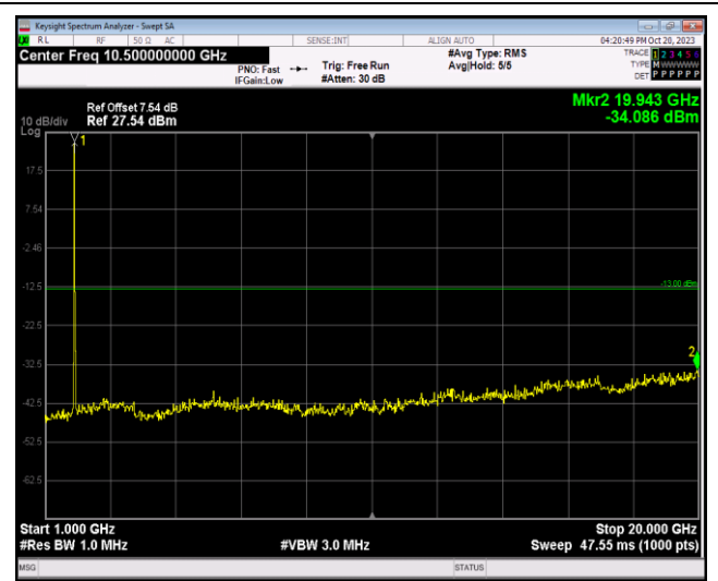
Band2-20MHz-16QAM-18900-1RB#0-Range2:1000~20000MHz
