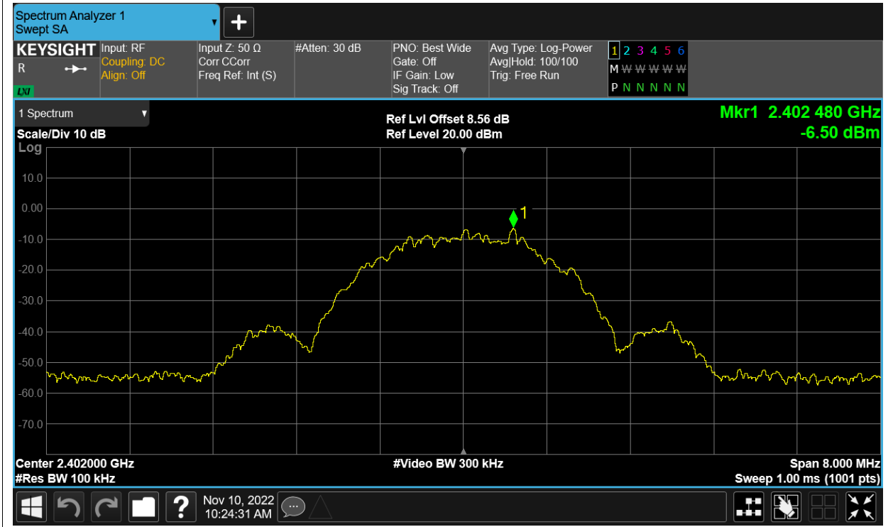
Band Edge NVNT BLE 2402MHz Ant3 Emission
