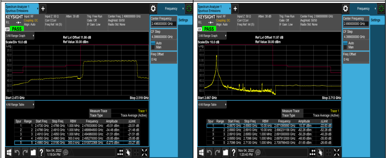
Band41-20MHz-QPSK-41490-1RB#99
