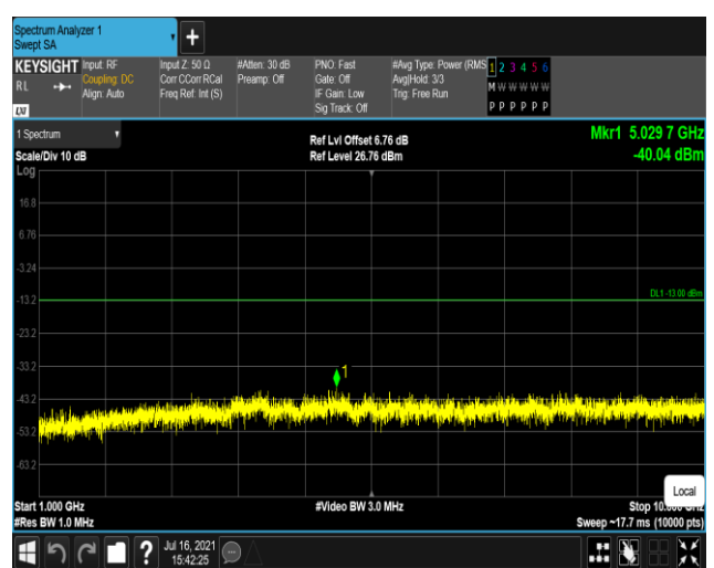
Band17-5MHz-QPSK-23825:1000~10000MHz
