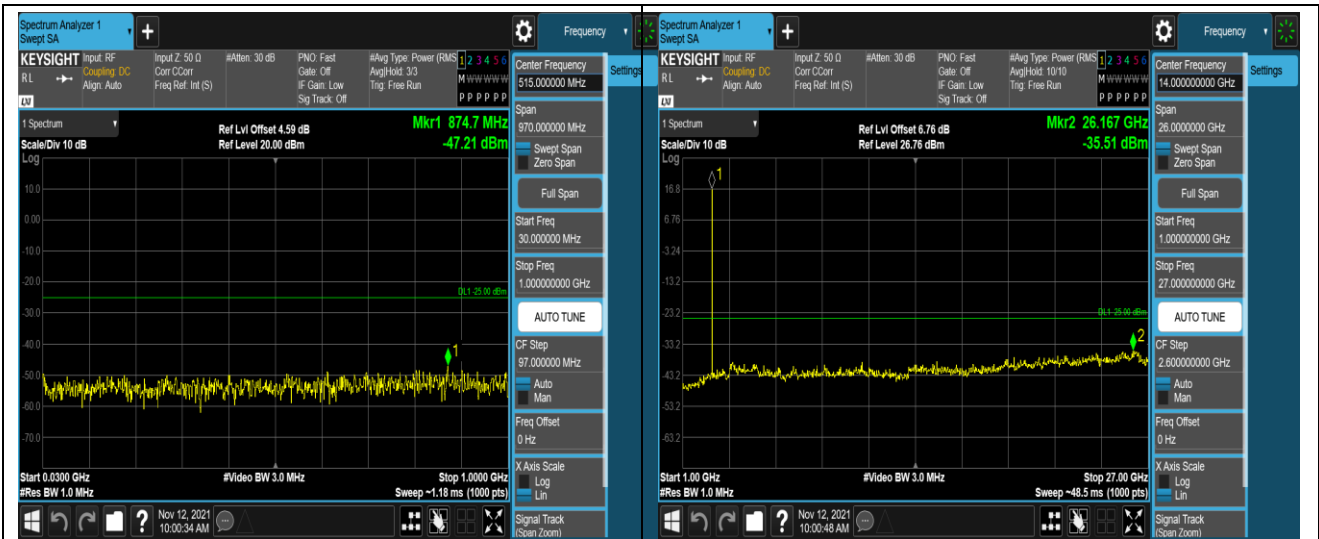
Band41-5MHz-QPSK-41215-1RB#0-Range 1:30~1000MHz
