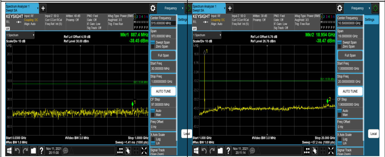
Band66-20MHz-QPSK-132072-1RB#0-Range 1:30 ~1000MHz
