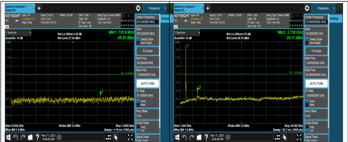
Band2-20MHz-QPSK-18900-1 RB#0-Range 1:30~1000MHz Band2-20MHz-QPSK-18900-1 RB#0-Range 2: 1000~20000MHz
