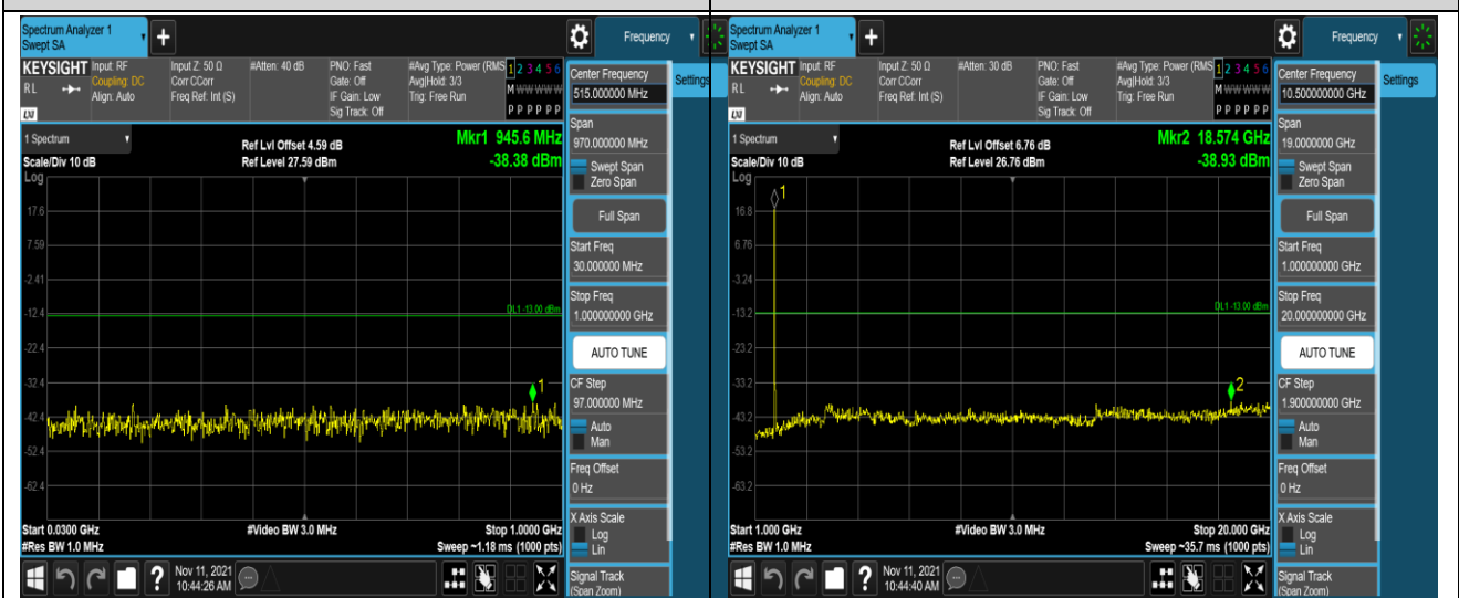
Band4-20MHz-QPSK-20050-1 RB#0-Range 1:30~1000MHz
