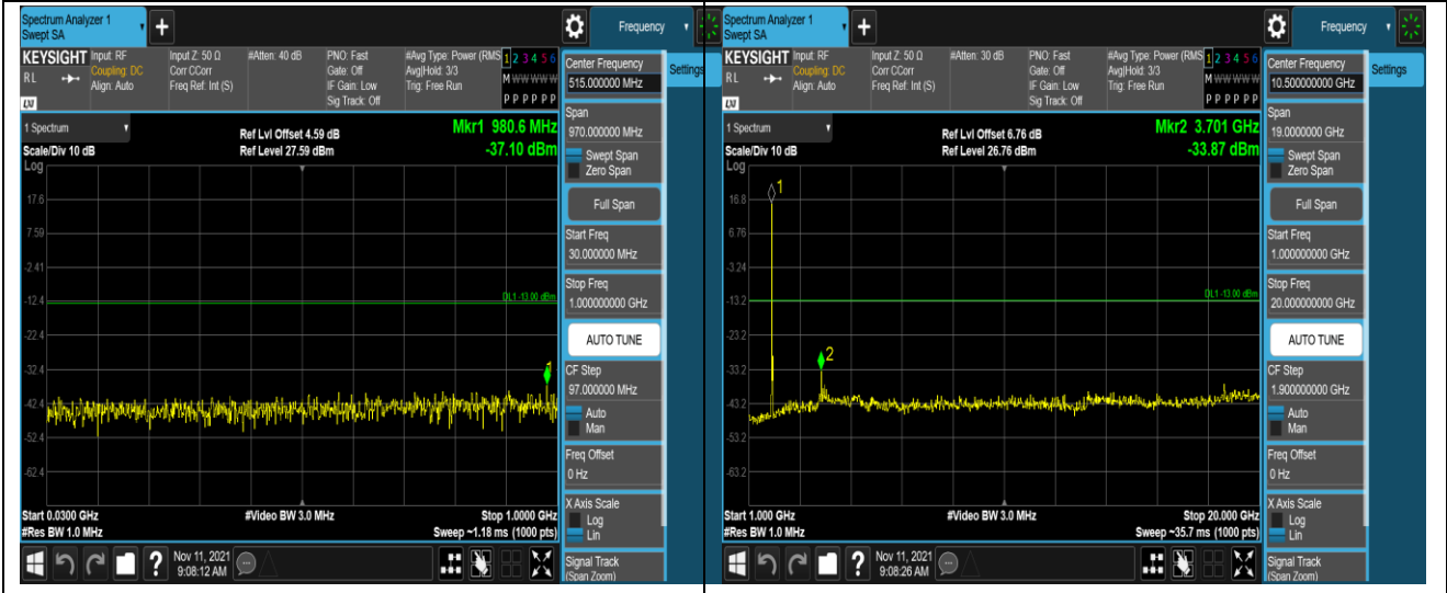
Band2-20MHz-QPSK-19100-1 RB#0-Range 1:30~1000MHz Band2-20MHz-QPSK-19100-1 RB#0-Range 2: 1000~20000MHz
