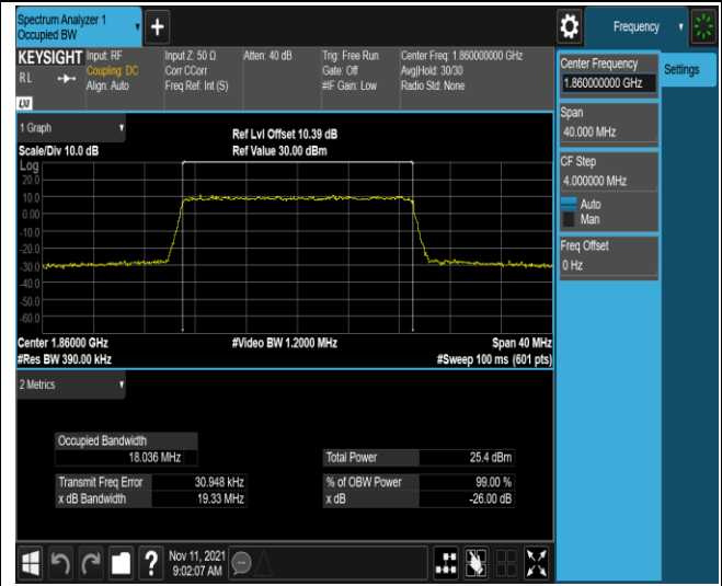
Band2-20MHz-16QAM-18700-100RB#0
