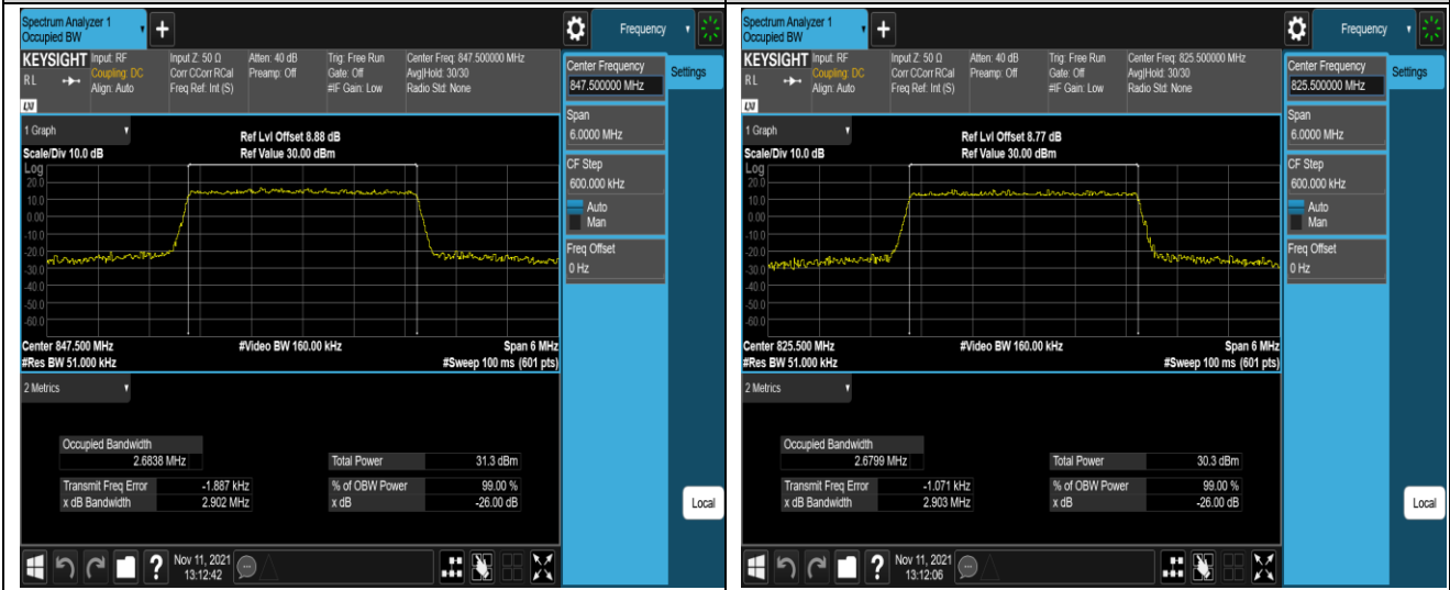
Band5-3MHz-QPSK-20635-15RB#0
