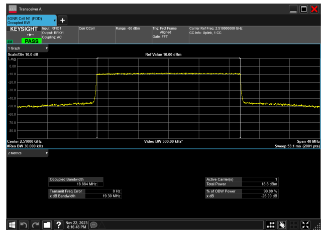
20MHz_15kHz_2510MHz_CP-OFDM 16 QAM_RB106@ 18.884 MHz
