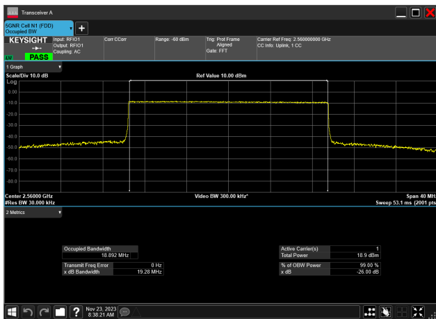
20MHz_15kHz_2560MHz_CP-OFDM QPSK_RB106@ 18.892 MHz
