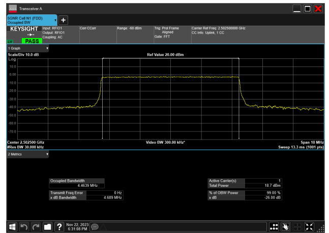
5MHz_15kHz_2502.5MHz_CP-OFDM QPSK_RB25@0 4.464 MHz
