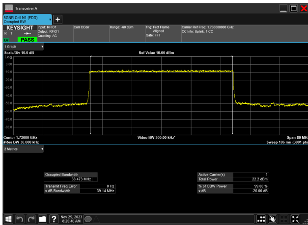
40MHz_15kHz_1730MHz_DFT-s-OFDM PI/2 BPSK_RB216@ 38.473 MHz
