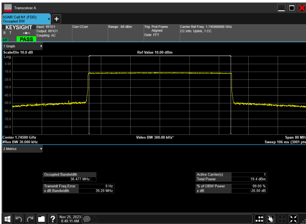
40MHz_15kHz_1745MHz_CP-OFDM QPSK_RB216@ 38.477 MHz
