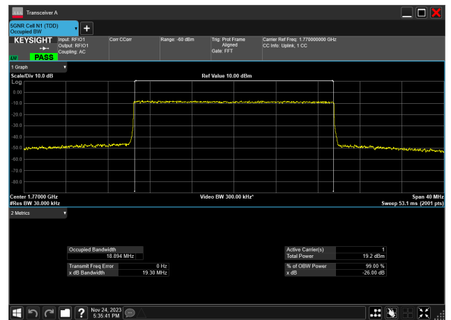
20MHz_15kHz_1770MHz_CP-OFDM 16 QAM_RB106@ 18.894 MHz
