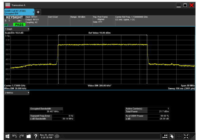
40MHz_15kHz_1730MHz_DFT-s-OFDM QPSK_RB216@ 38.467 MHz
