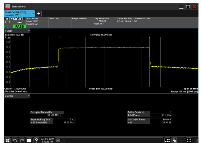
40MHz_15kHz_1730MHz_CP-OFDM QPSK_RB216@ 38.508 MHz
