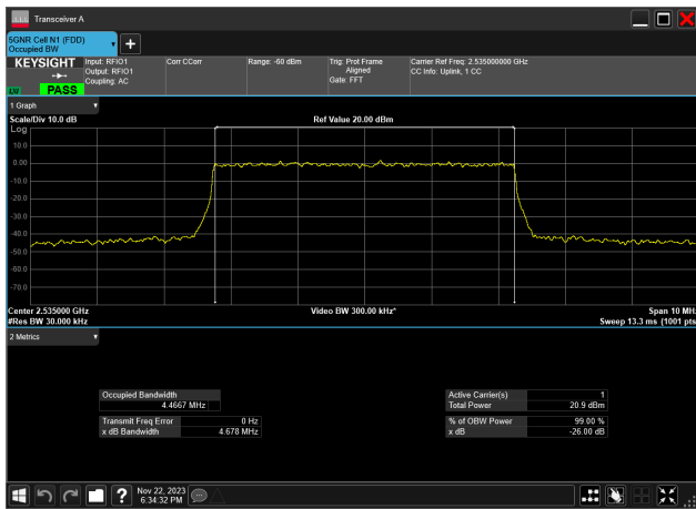
5MHz_15kHz_2535MHz_DFT-s-OFDM QPSK_RB25@0 4.467 MHz
