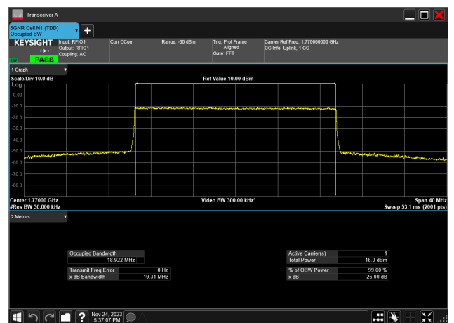
20MHz_15kHz_1770MHz_CP-OFDM 256 QAM_RB106@ 18.922 MHz
