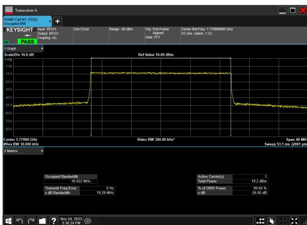
20MHz_15kHz_1770MHz_CP-OFDM 64 QAM_RB106@ 18.922 MHz
