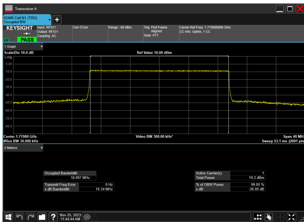
20MHz_15kHz_1770MHz_CP-OFDM QPSK_RB106@ 18.897 MHz
