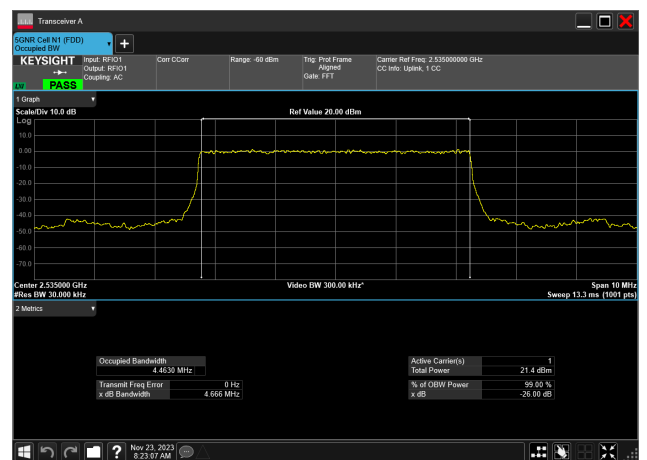
5MHz_15kHz_2535MHz_DFT-s-OFDM PI/2 BPSK_RB25@0 4.463 MHz
