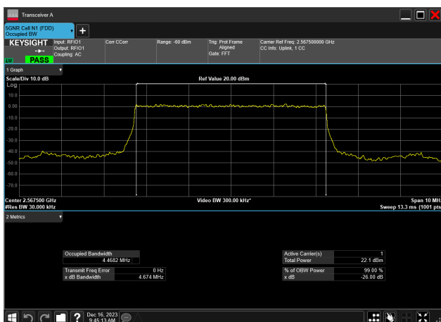
5MHz_15kHz_2567.5MHz_DFT-s-OFDM PI/2 BPSK_RB25@ 4.468 MHz
