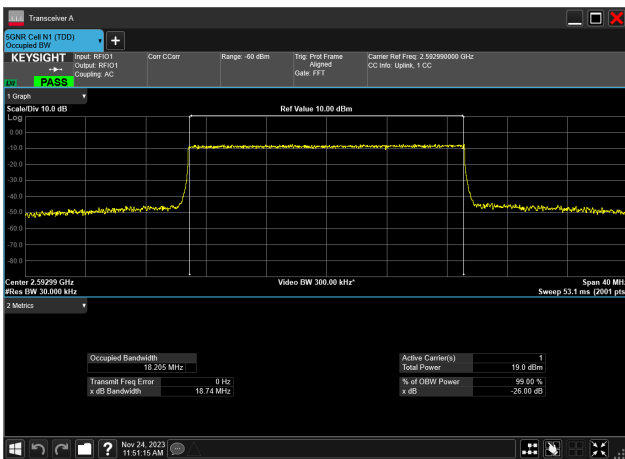
20MHz_30kHz_2592.99MHz_CP-OFDM QPSK_RB51@0 18.205 MHz
