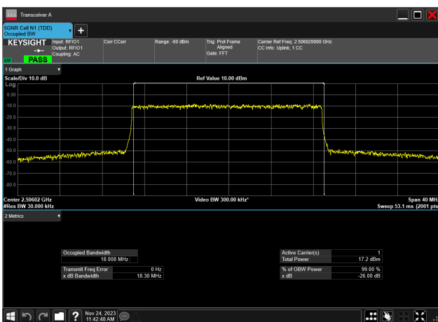
20MHz_30kHz_2506.02MHz_DFT-s-OFDM 256 QAM_RB50@0 18.008 MHz
