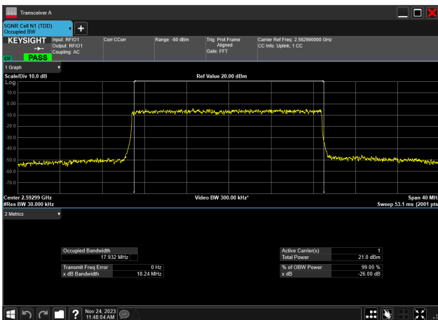
20MHz_30kHz_2592.99MHz_DFT-s-OFDM QPSK_RB50@0 17.932 MHz
