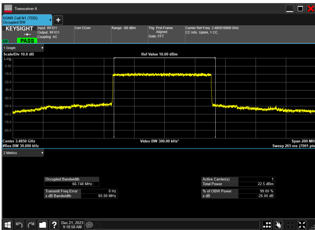
70MHz_30kHz_3485MHz_DFT-s-OFDM QPSK_RB180@0 66.748 MHz
