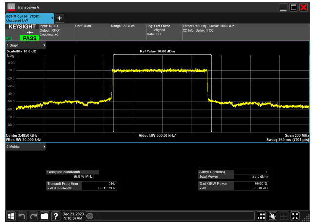
70MHz_30kHz_3485MHz_DFT-s-OFDM PI/2 BPSK_RB180@0 66.876 MHz
