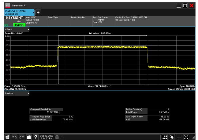
80MHz_30kHz_3490MHz_DFT-s-OFDM QPSK_RB216@ 76.972 MHz
