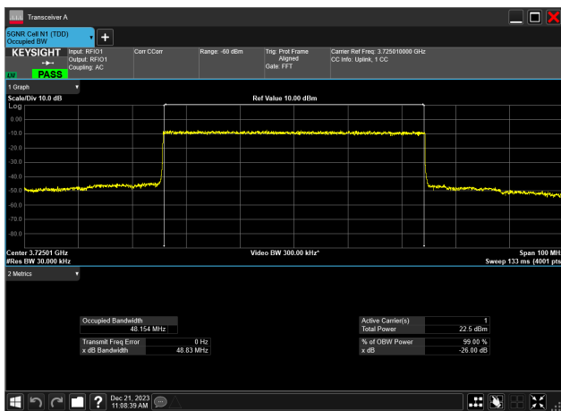
50MHz_15kHz_3725MHz_DFT-s-OFDM QPSK_RB270@0 48.154 MHz
