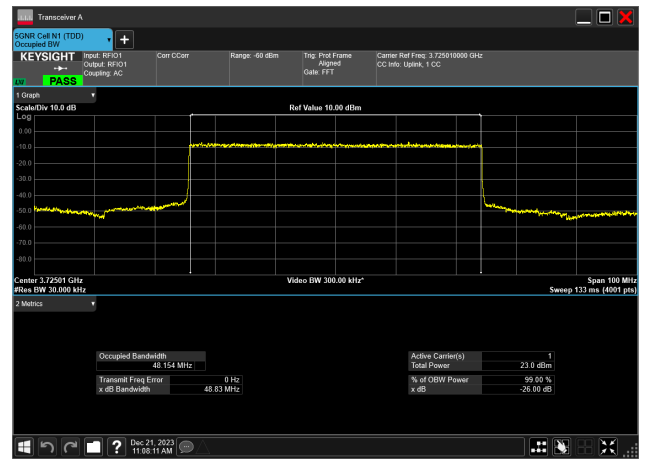
50MHz_15kHz_3725MHz_DFT-s-OFDM PI/2 BPSK_RB270@0 48.154 MHz
