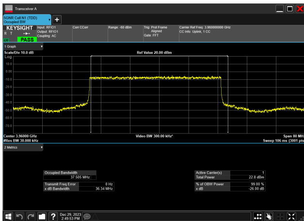
40MHz_30kHz_3960MHz_DFT-s-OFDM PI/2 BPSK_RB100@0 37.505 MHz
