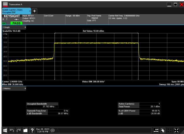
40MHz_30kHz_3960MHz_CP-OFDM QPSK_RB106@0 37.783 MHz
