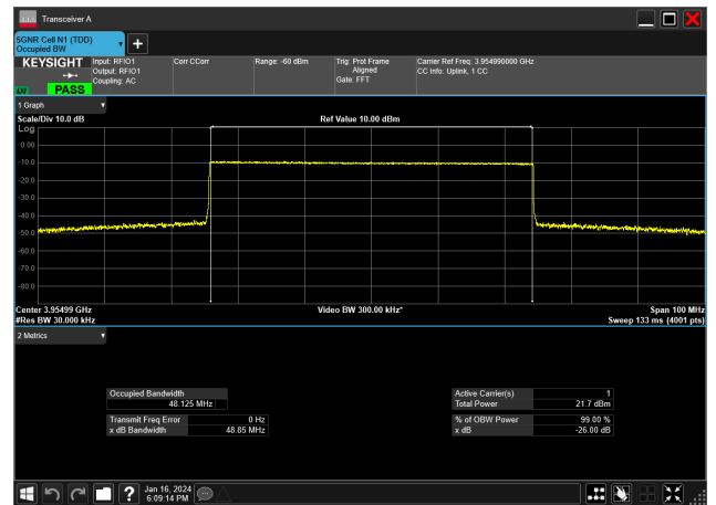
50MHz_15kHz_3955MHz_CP-OFDM QPSK_RB270@0 48.125 MHz
