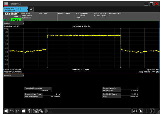
50MHz_15kHz_3955MHz_DFT-s-OFDM PI/2 BPSK_RB270@ 48.111 MHz
