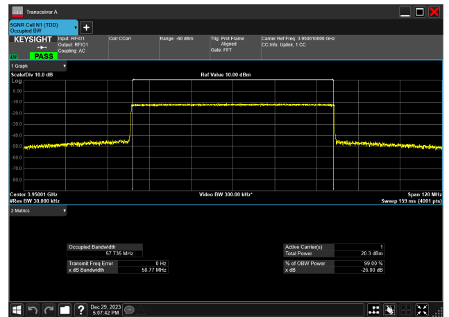
60MHz_30kHz_3950MHz_CP-OFDM QPSK_RB162@0 57.735 MHz
