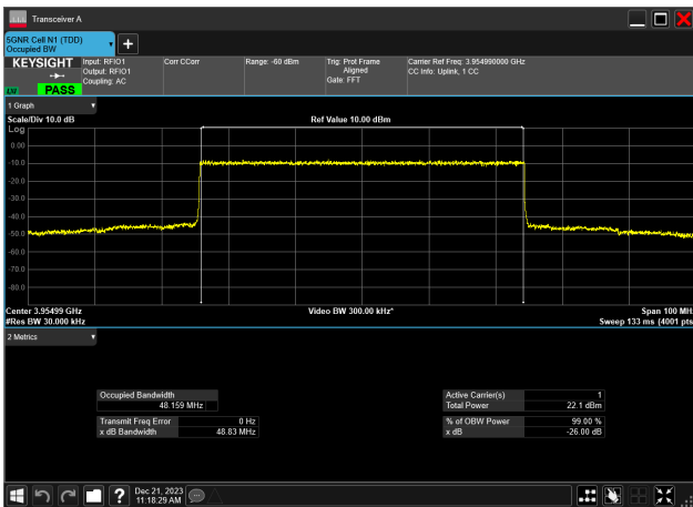
50MHz_15kHz_3955MHz_DFT-s-OFDM QPSK_RB270@ 48.159 MHz
