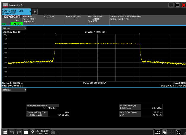
40MHz_30kHz_3720MHz_CP-OFDM QPSK_RB106@ 37.774 MHz
