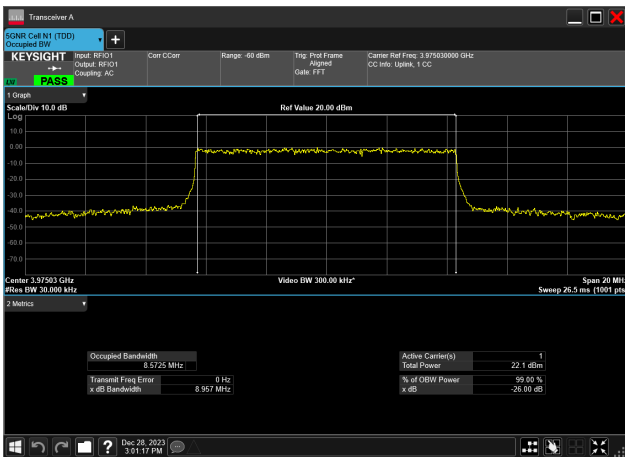
10MHz_30kHz_3975MHz_DFT-s-OFDM QPSK_RB24@0 8.573 MHz
