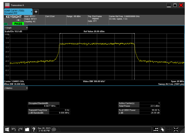
10MHz_30kHz_3840MHz_DFT-s-OFDM QPSK_RB24@0 8.568 MHz
