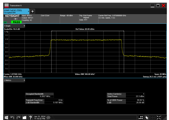
10MHz_15kHz_3975MHz_DFT-s-OFDM QPSK_RB50@0 9.206 MHz
