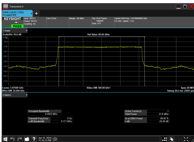
10MHz_15kHz_3975MHz_DFT-s-OFDM PI/2 BPSK_RB50@0 9.206 MHz
