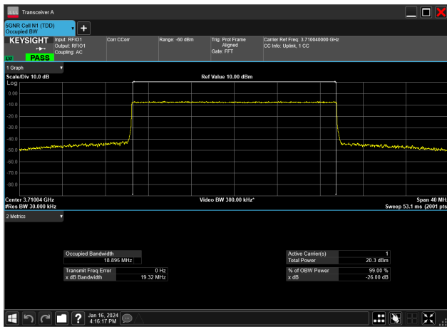
20MHz_15kHz_3710MHz_CP-OFDM QPSK_RB106@ 18.895 MHz
