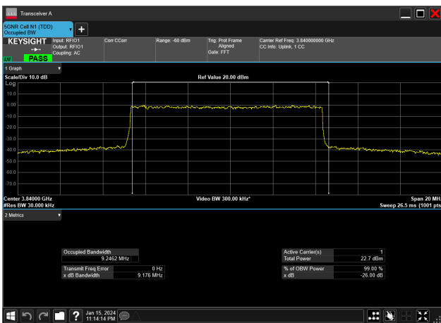
10MHz_15kHz_3840MHz_DFT-s-OFDM QPSK_RB50@0 9.246 MHz
