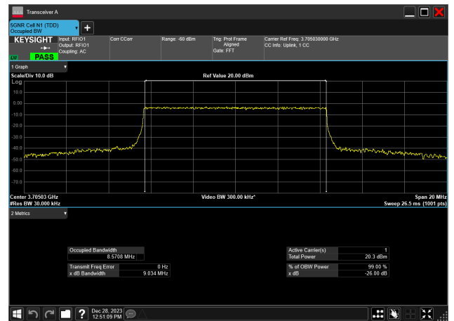
10MHz_30kHz_3705MHz_CP-OFDM QPSK_RB24@ 8.571 MHz
