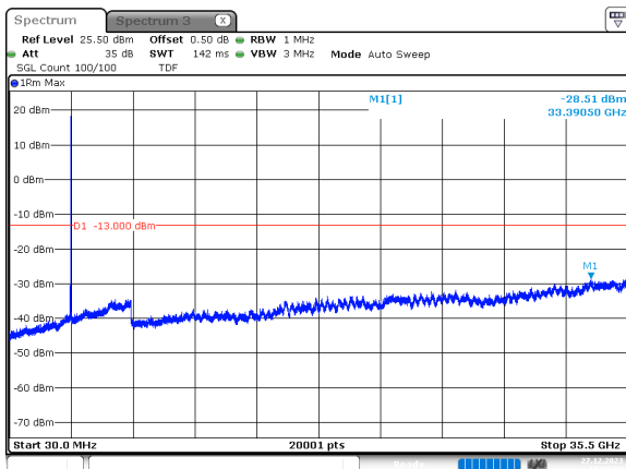
80MHz_30kHz_3510MHz_DFT-s-OFDM QPSK_RB1@216 -28.51 dBm
