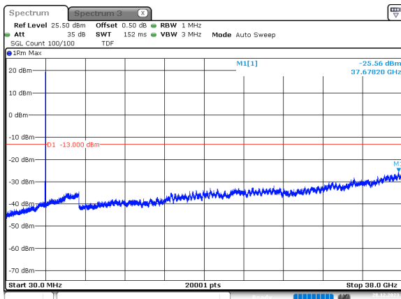
70MHz_30kHz_3750MHz_DFT-s-OFDM QPSK_RB1@188 -25.56 dBm
