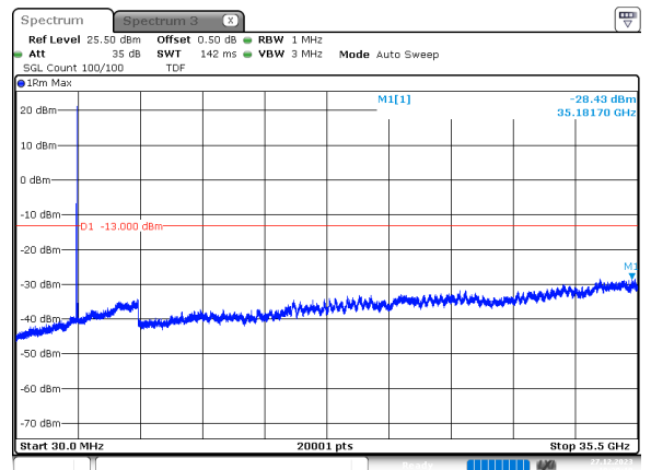
70MHz_30kHz_3500MHz_DFT-s-OFDM QPSK_RB1@0 -28.43 dBm
