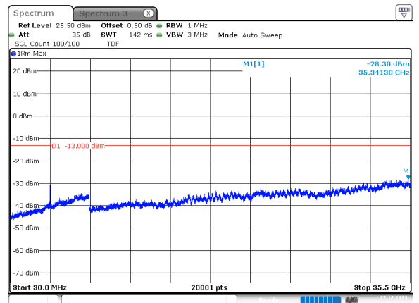
90MHz_30kHz_3500MHz_DFT-s-OFDM QPSK_RB1@0 -28.30 dBm
