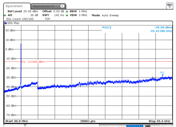
70MHz_30kHz_3500MHz_DFT-s-OFDM QPSK_RB180@0 -28.38 dBm
