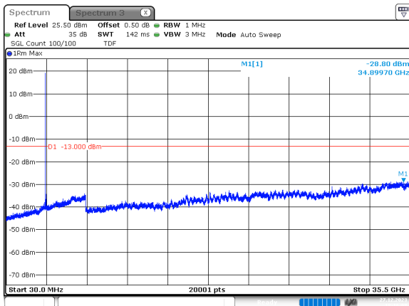
70MHz_30kHz_3485MHz_DFT-s-OFDM QPSK_RB1@0 -28.80 dBm
