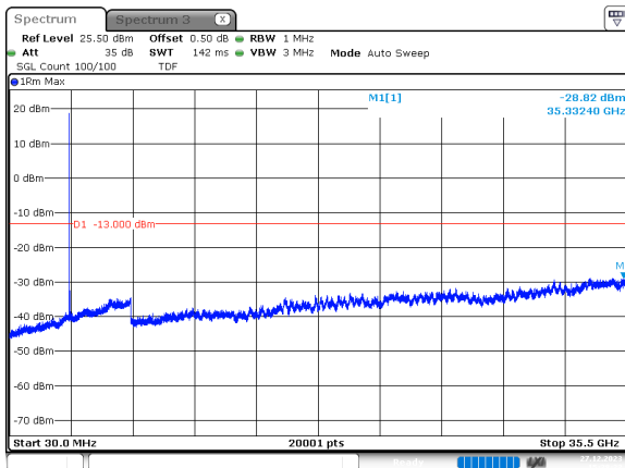
30MHz_30kHz_3465MHz_DFT-s-OFDM QPSK_RB1@0 -28.82 dBm
