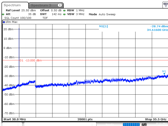
30MHz_30kHz_3535MHz_DFT-s-OFDM QPSK_RB1@0 -28.74 dBm
