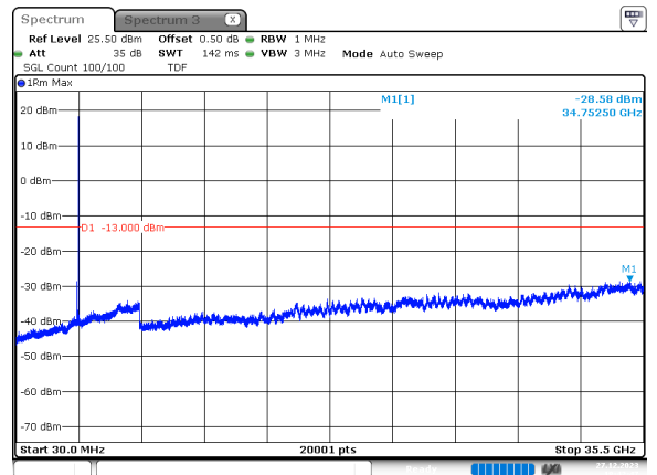
90MHz_30kHz_3495MHz_DFT-s-OFDM QPSK_RB1@244 -28.58 dBm
