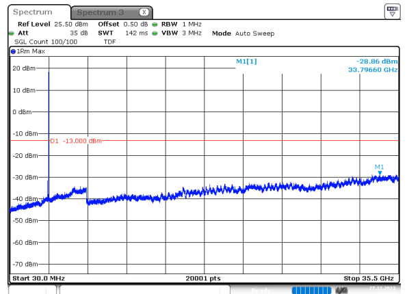
80MHz_30kHz_3500MHz_DFT-s-OFDM QPSK_RB1@216 -28.86 dBm
