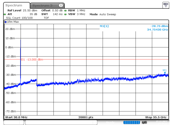
40MHz_30kHz_3530MHz_DFT-s-OFDM QPSK_RB100@0 -28.75 dBm
