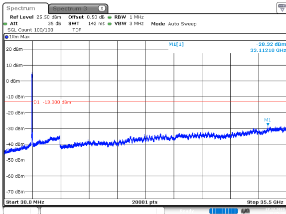
80MHz_30kHz_3500MHz_DFT-s-OFDM QPSK_RB216@0 -28.32 dBm
