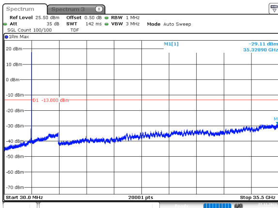
80MHz_30kHz_3490MHz_DFT-s-OFDM QPSK_RB1@216 -29.11 dBm
