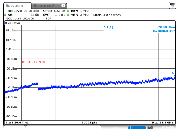
60MHz_30kHz_3520MHz_DFT-s-OFDM QPSK_RB1@0 -28.50 dBm
