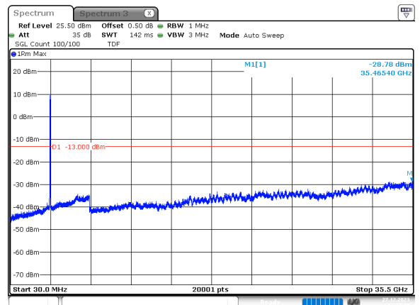
30MHz_30kHz_3500MHz_DFT-s-OFDM QPSK_RB75@0 -28.78 dBm
