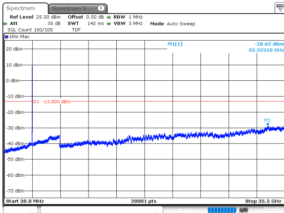
30MHz_30kHz_3535MHz_DFT-s-OFDM QPSK_RB75@0 -28.62 dBm
