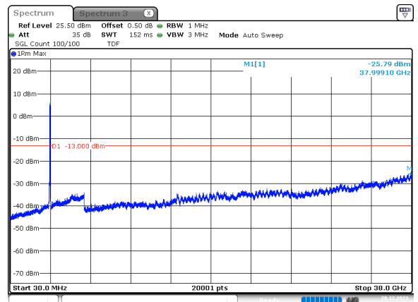
70MHz_30kHz_3750MHz_DFT-s-OFDM QPSK_RB180@0 -25.79 dBm
