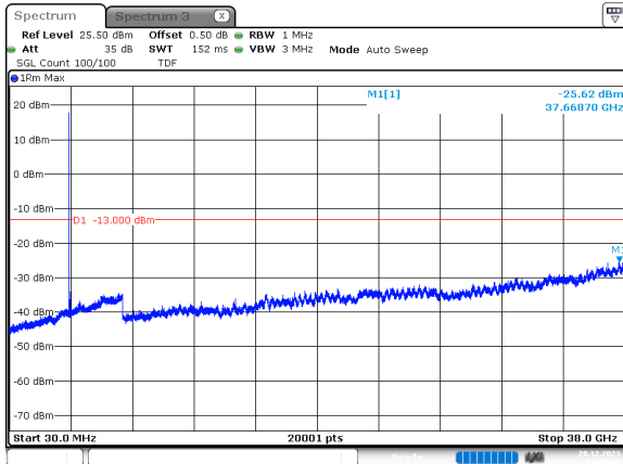
70MHz_30kHz_3735MHz_DFT-s-OFDM QPSK_RB1@0 -25.62 dBm
