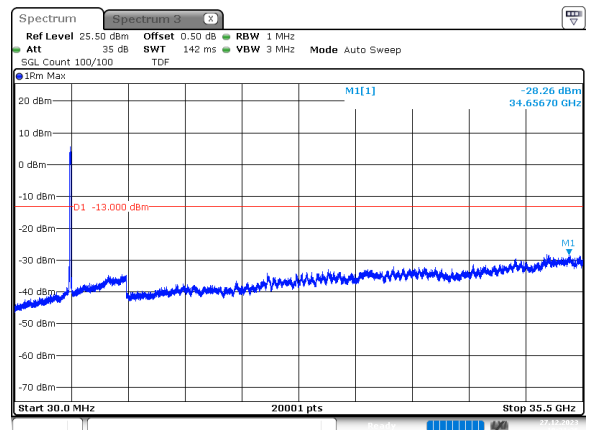
80MHz_30kHz_3490MHz_DFT-s-OFDM QPSK_RB216@0 -28.26 dBm
