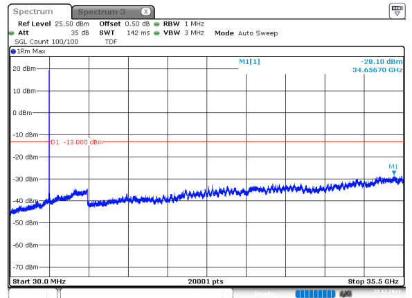
80MHz_30kHz_3510MHz_DFT-s-OFDM QPSK_RB1@0 -28.10 dBm
