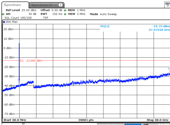
70MHz_30kHz_3765MHz_DFT-s-OFDM QPSK_RB180@0 -25.73 dBm
