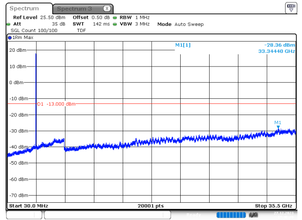
40MHz_30kHz_3530MHz_DFT-s-OFDM QPSK_RB1@0 -28.36 dBm
