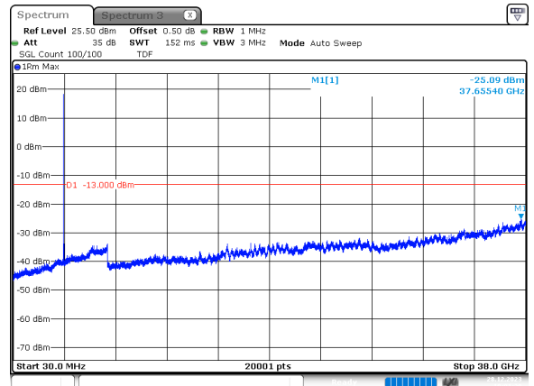
70MHz_30kHz_3750MHz_DFT-s-OFDM QPSK_RB1@0 -25.09 dBm
