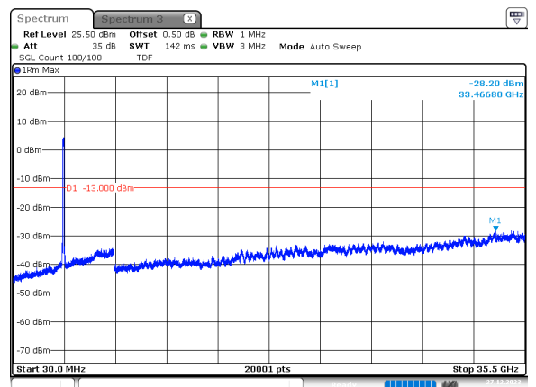
90MHz_30kHz_3500MHz_DFT-s-OFDM QPSK_RB243@0 -28.20 dBm
