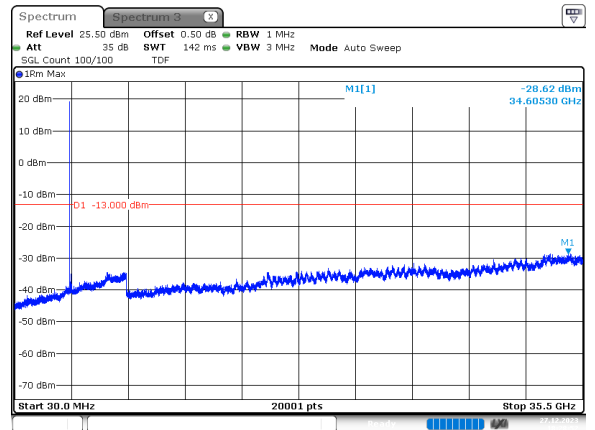
80MHz_30kHz_3490MHz_DFT-s-OFDM QPSK_RB1@0 -28.62 dBm
