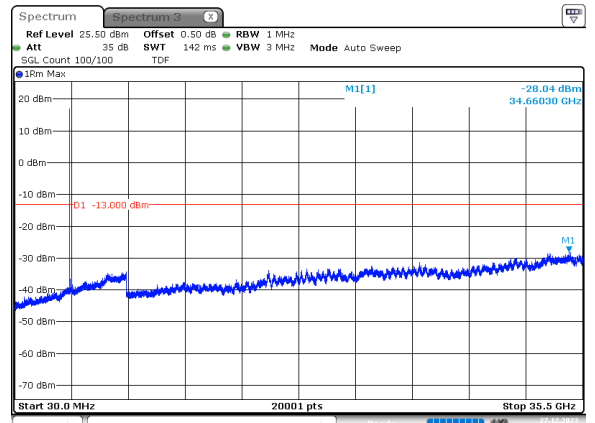
60MHz_30kHz_3480MHz_DFT-s-OFDM QPSK_RB1@0 -28.04 dBm
