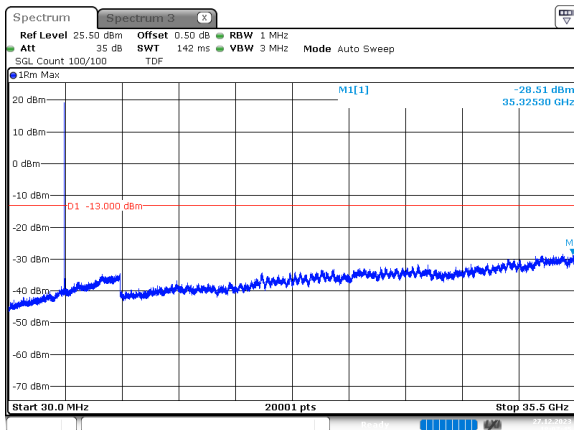
60MHz_30kHz_3500MHz_DFT-s-OFDM QPSK_RB1@0 -28.51 dBm
