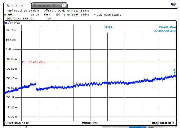
70MHz_30kHz_3765MHz_DFT-s-OFDM QPSK_RB1@188 -25.53 dBm
