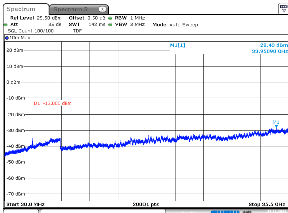
90MHz_30kHz_3505MHz_DFT-s-OFDM QPSK_RB1@0 -28.43 dBm
