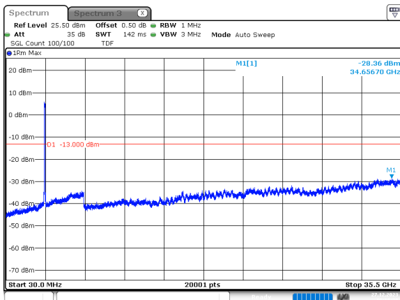
70MHz_30kHz_3485MHz_DFT-s-OFDM QPSK_RB180@0 -28.36 dBm
