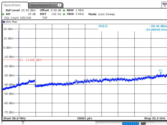
90MHz_30kHz_3495MHz_DFT-s-OFDM QPSK_RB1@0 -28.46 dBm
