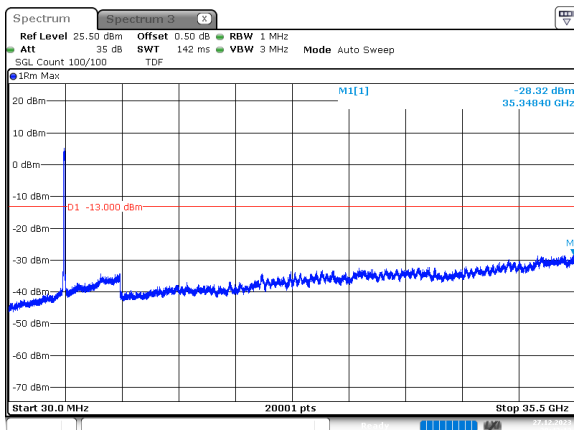
90MHz_30kHz_3495MHz_DFT-s-OFDM QPSK_RB243@0 -28.32 dBm
