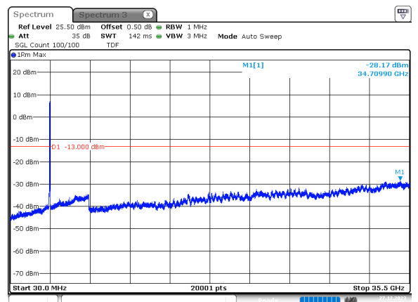
60MHz_30kHz_3520MHz_DFT-s-OFDM QPSK_RB162@0 -28.17 dBm
