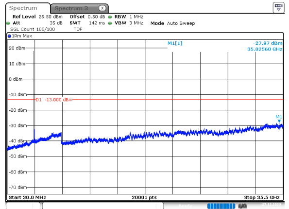
40MHz_30kHz_3470MHz_DFT-s-OFDM QPSK_RB1@0 -27.97 dBm
