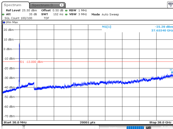
70MHz_30kHz_3735MHz_DFT-s-OFDM QPSK_RB180@0 -25.28 dBm
