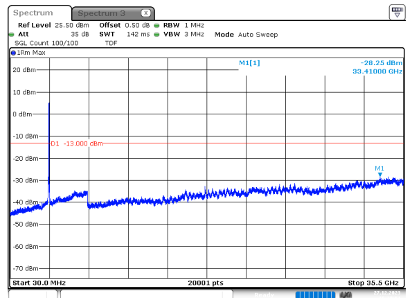
80MHz_30kHz_3510MHz_DFT-s-OFDM QPSK_RB216@0 -28.25 dBm
