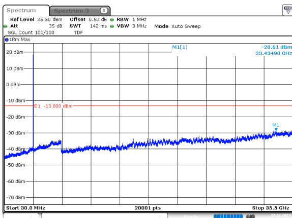
25MHz_30kHz_3537.5MHz_DFT-s-OFDM QPSK_RB1@64 -28.61 dBm
