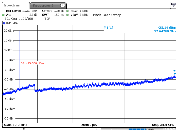
70MHz_30kHz_3765MHz_DFT-s-OFDM QPSK_RB1@0 -25.14 dBm
