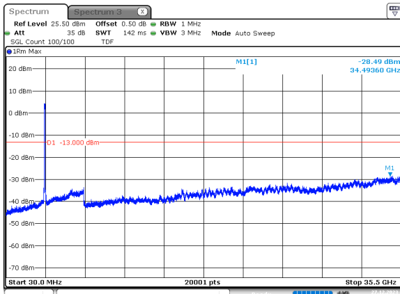
90MHz_30kHz_3505MHz_DFT-s-OFDM QPSK_RB243@0 -28.49 dBm
