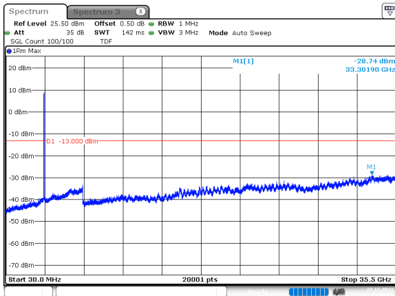
30MHz_30kHz_3465MHz_DFT-s-OFDM QPSK_RB75@0 -28.74 dBm
